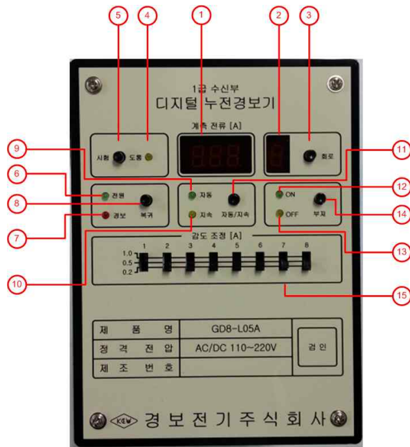
【Figure 1. 전면부】
