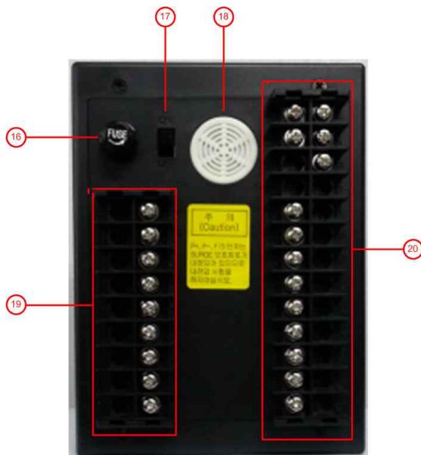
【Figure 2. 후면부】
