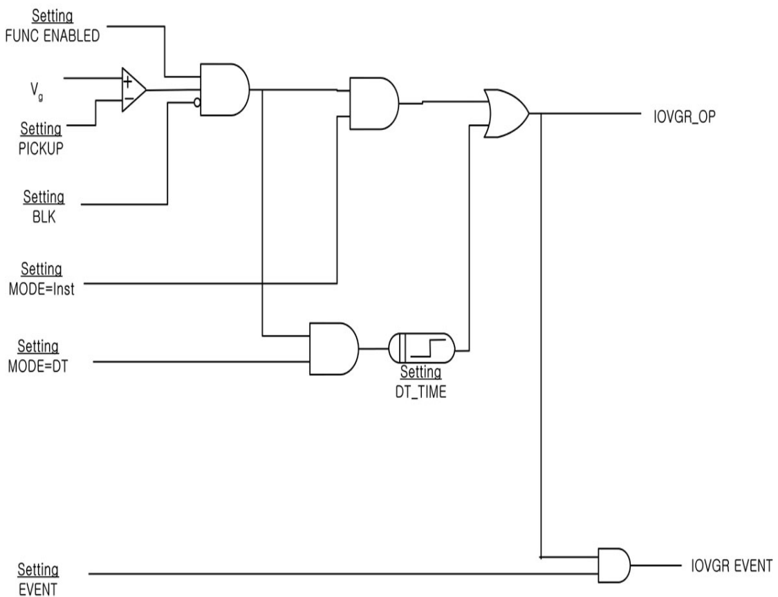
<Figure 5. 순시 지락 과전압 요소 Logic Diagram>
