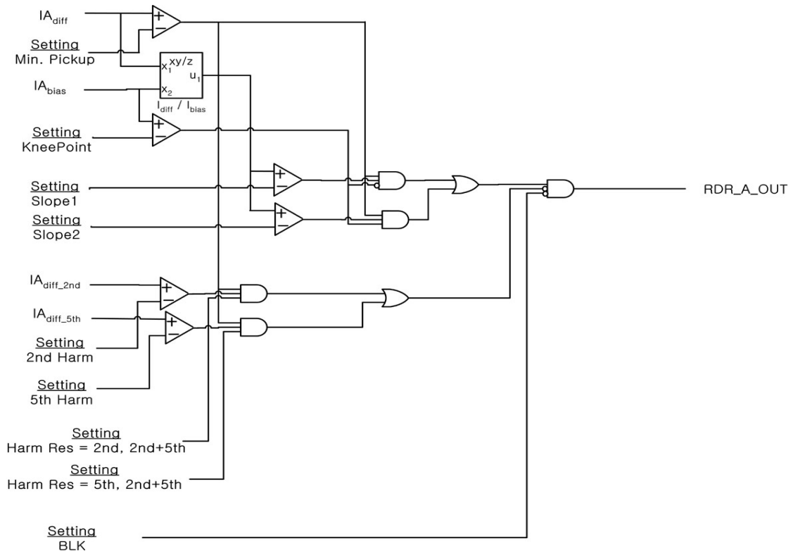
<Figure 4. 비율 차동 요소 A상 Logic Diagram>
