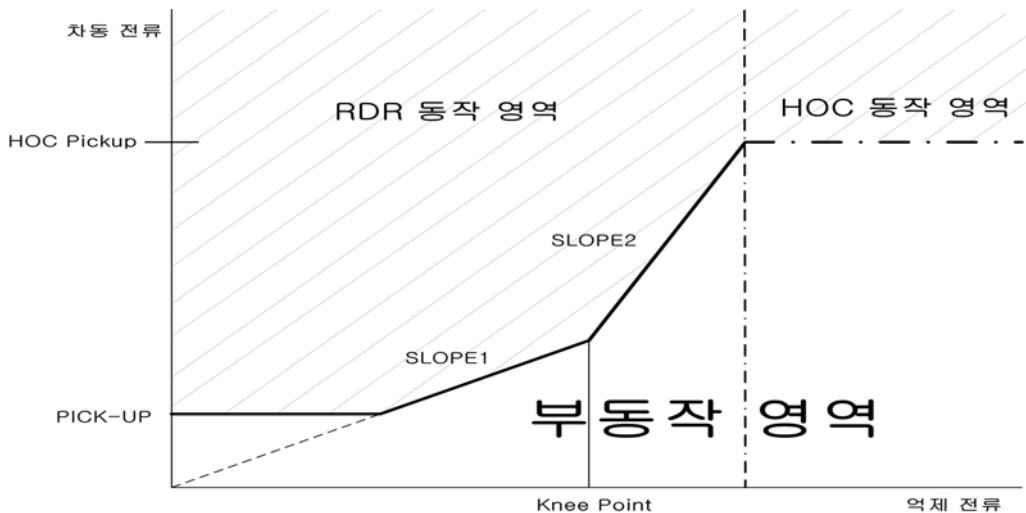
<Figure 2. 비율 차동 요소 동작 특성>
