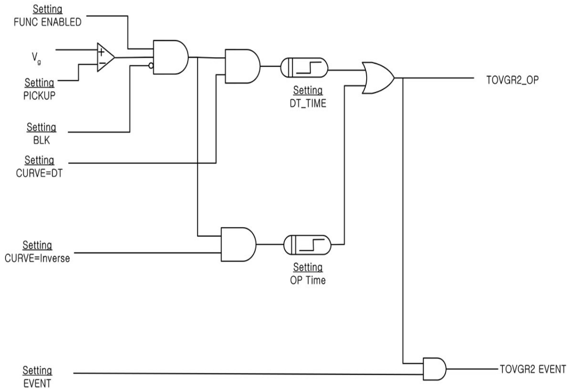
<Figure 7. Alarm용 한시 지락 과전압 요소 Logic Diagram>
