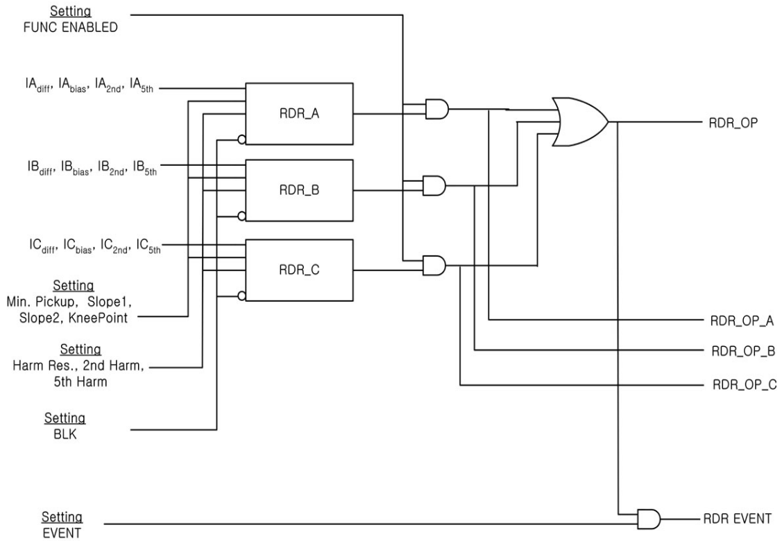
<Figure 3. 비율 차동 요소 Logic Diagram>
