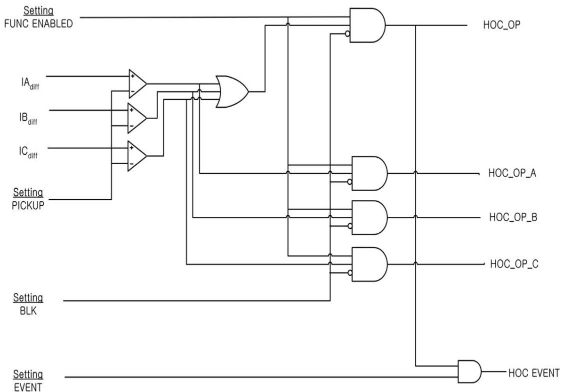
<Figure 1. 순시 차동 요소 Logic Diagram>
