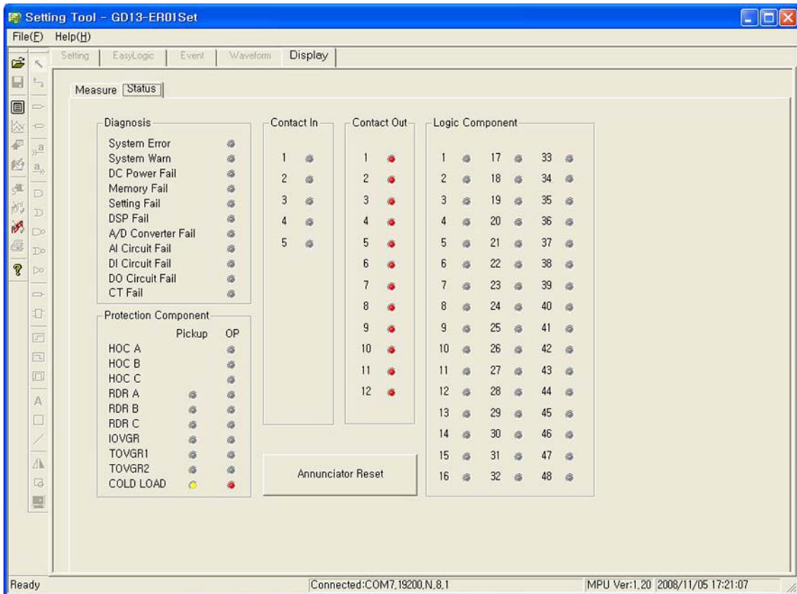
<Figure 21. Display ▶ Status 화면 표시>
