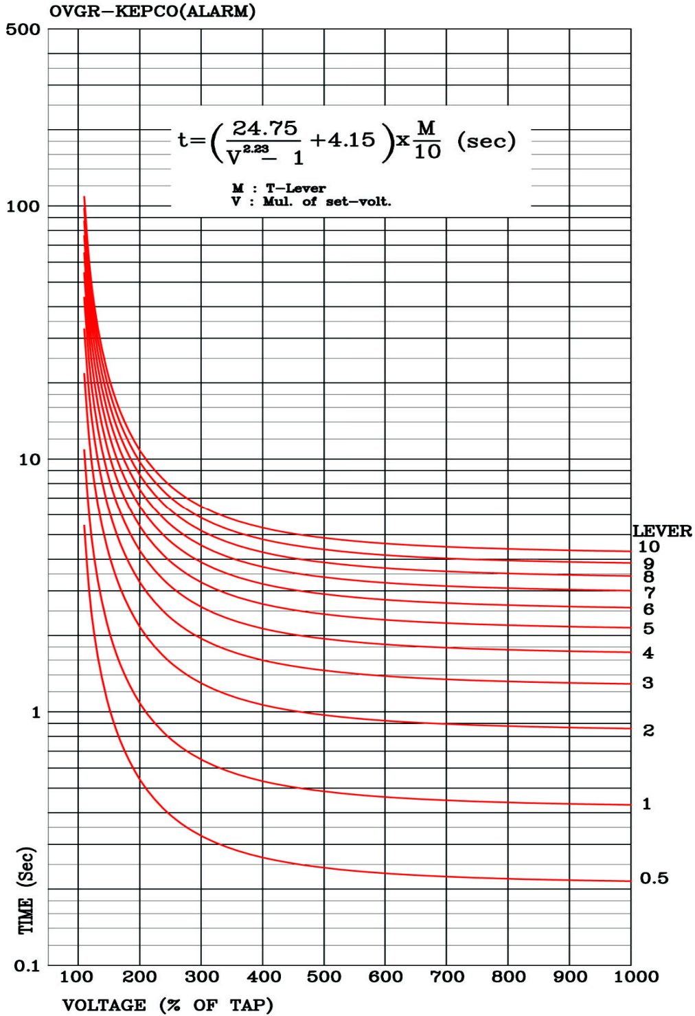
<부도 4.3 Alarm용 한시 지락과전압 반한시 특성 곡선>
