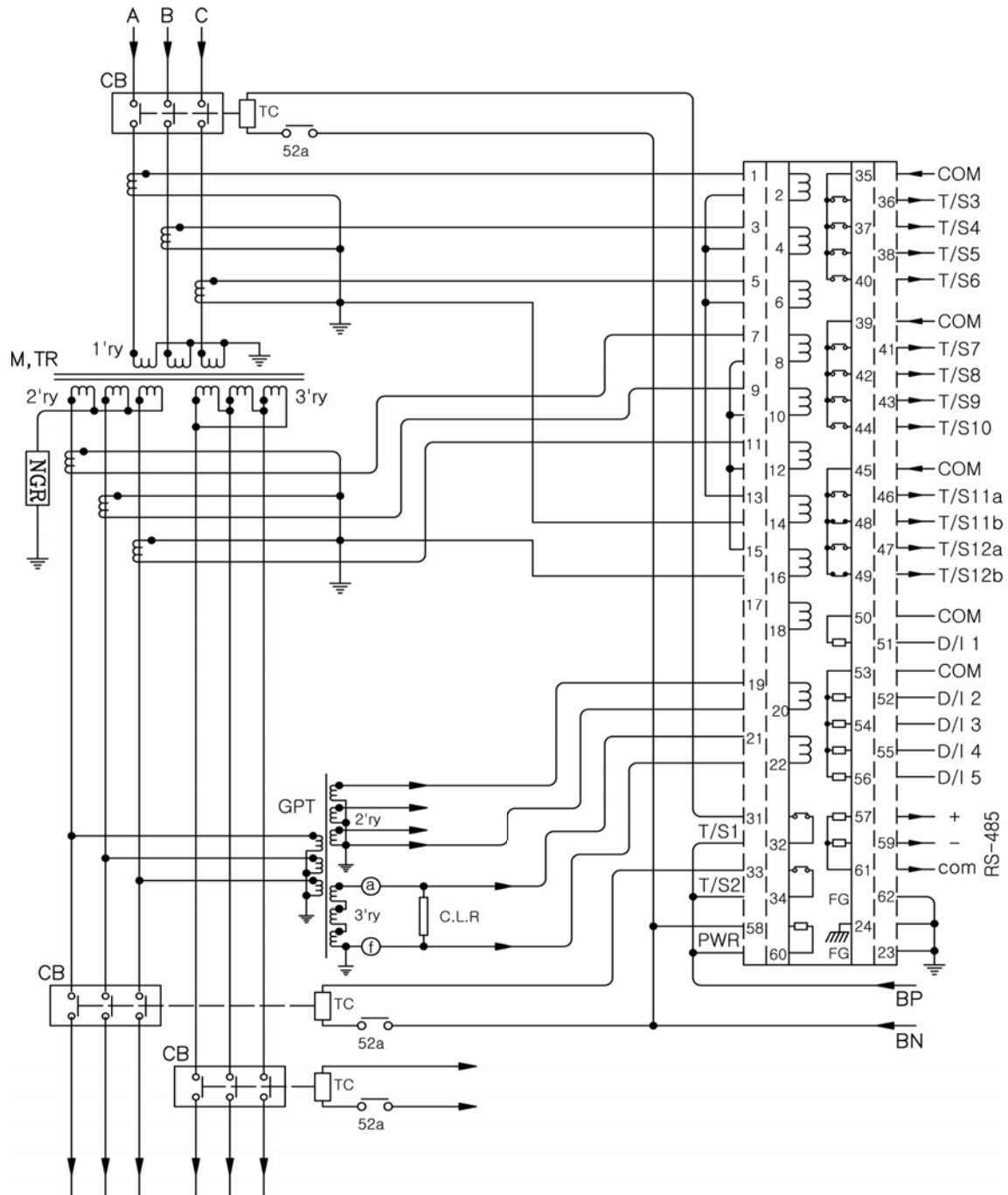
<부도 3.3 계전기 CT Fail Block을 사용 할 경우 외부 결선도>
