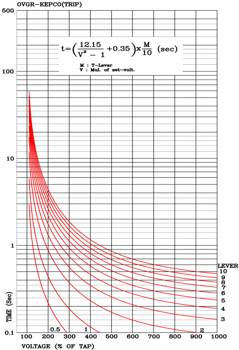
<부도 4.2 Trip용 한시 지락과전압 반한시 특성 곡선>
