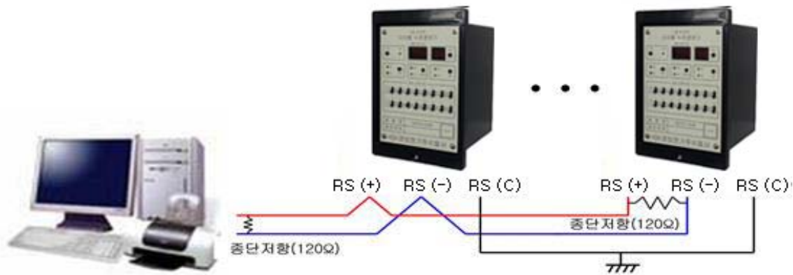
【Figure 1. RS-485 결선도】
