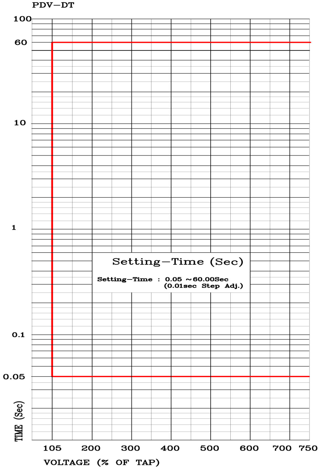
<부도 5.3 PDV 정한시 특성 곡선>
