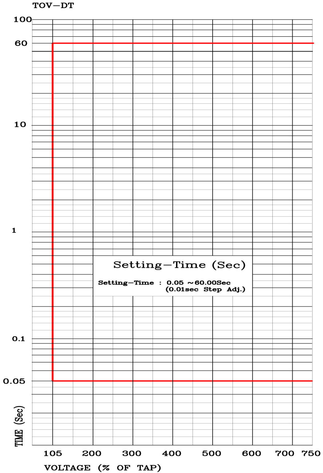
<부도 5.5 TOV 정한시 특성 곡선>
