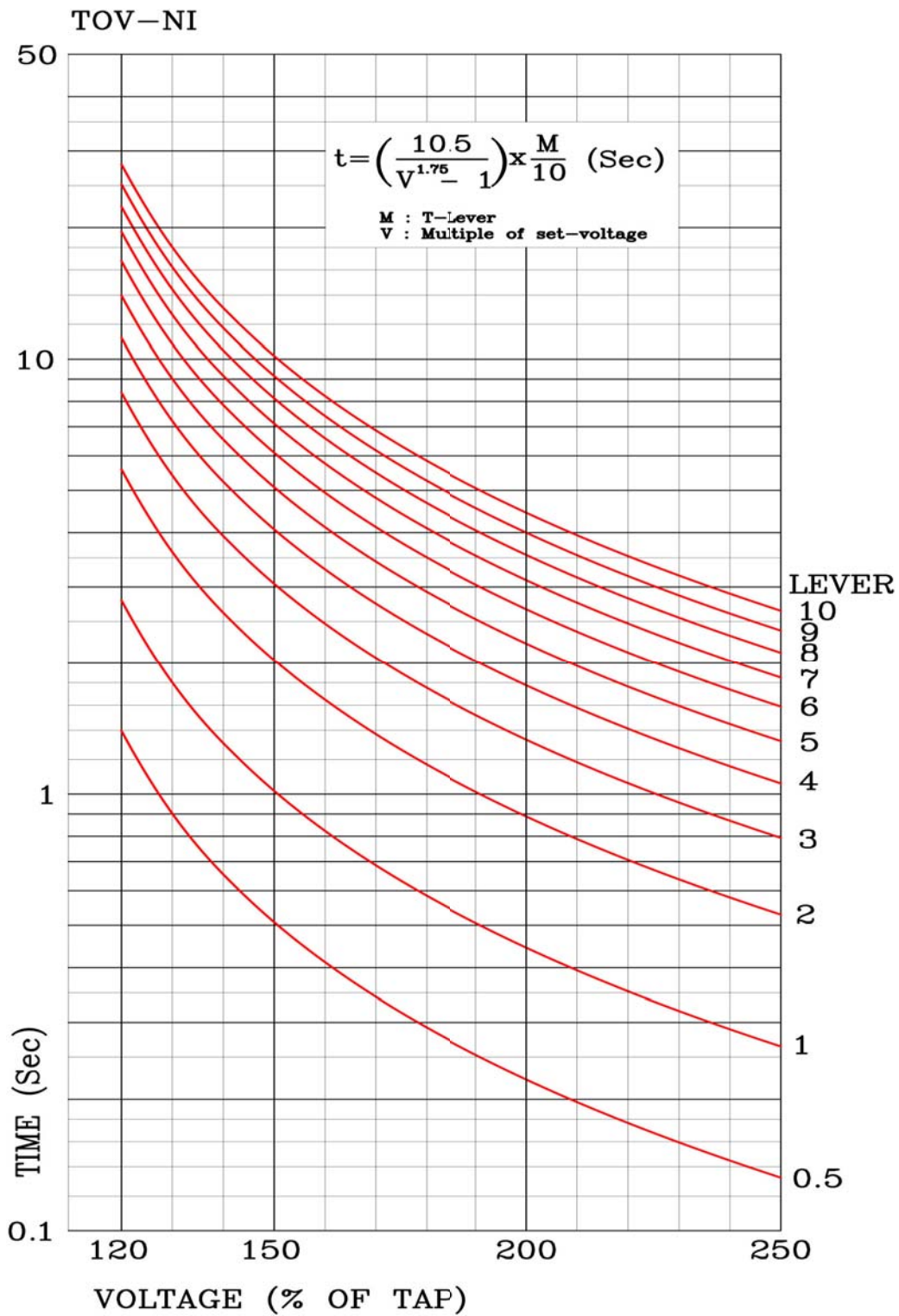
<부도 5.4 TOV 반한시 특성 곡선>
