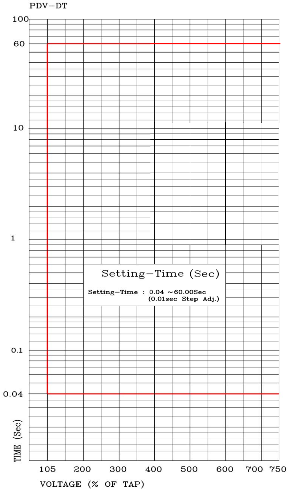
<부도 5.3 PDV 정한시 특성 곡선>
