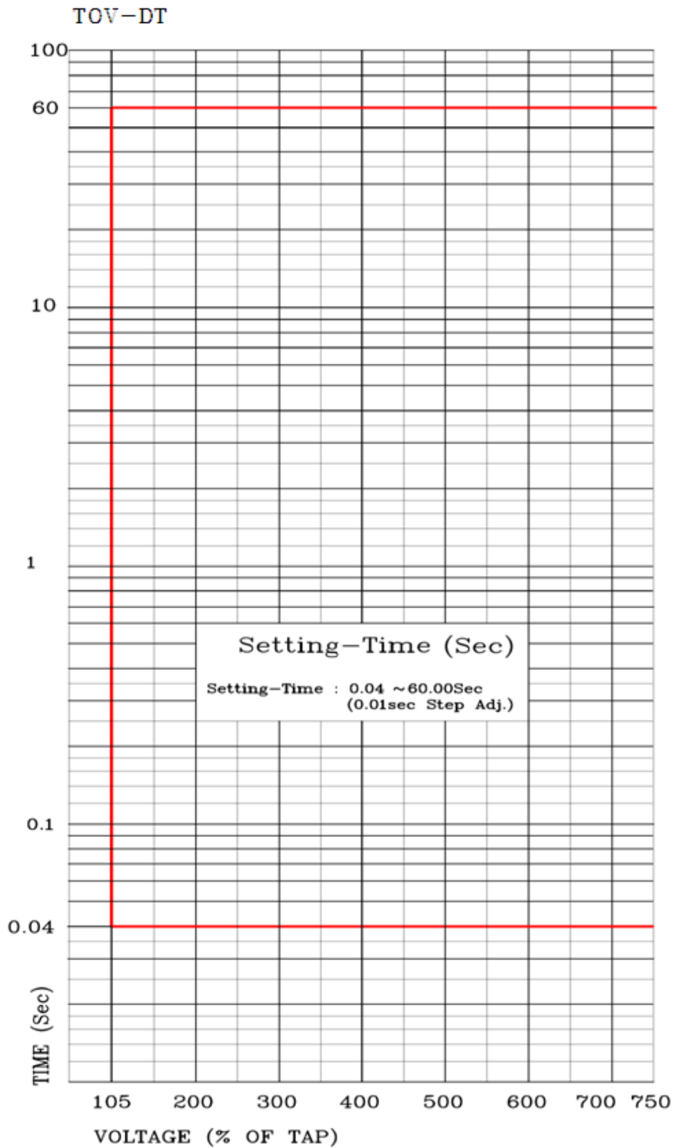
<부도 5.5 TOV 정한시 특성 곡선>
