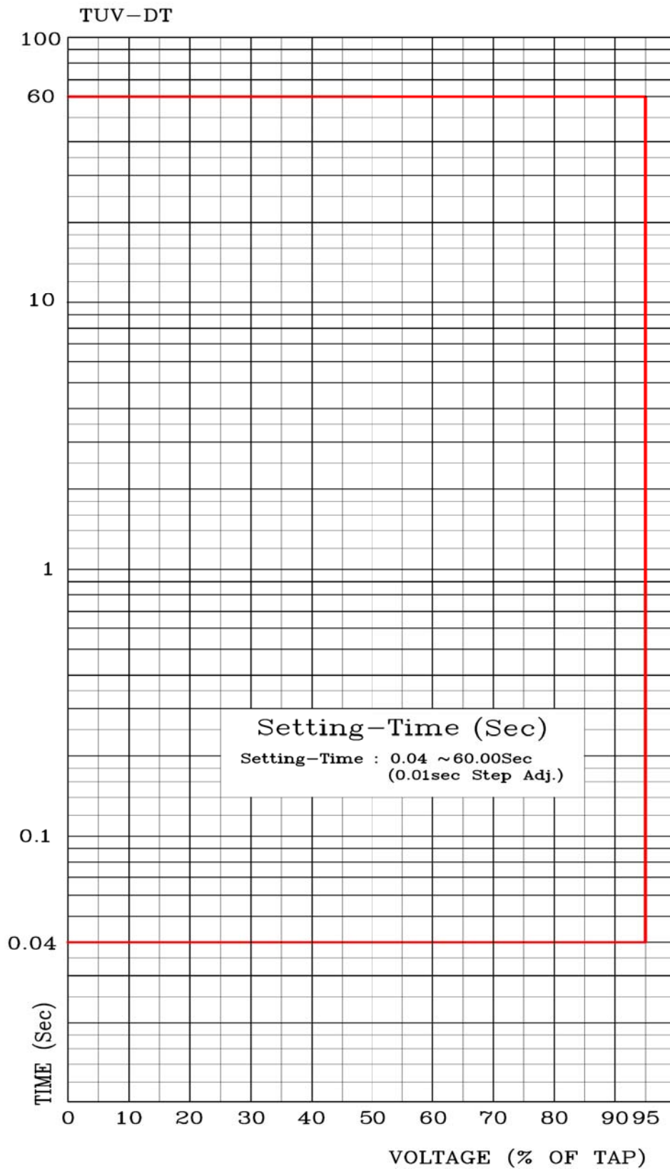
<부도 5.7 TUV 정한시 특성 곡선>
