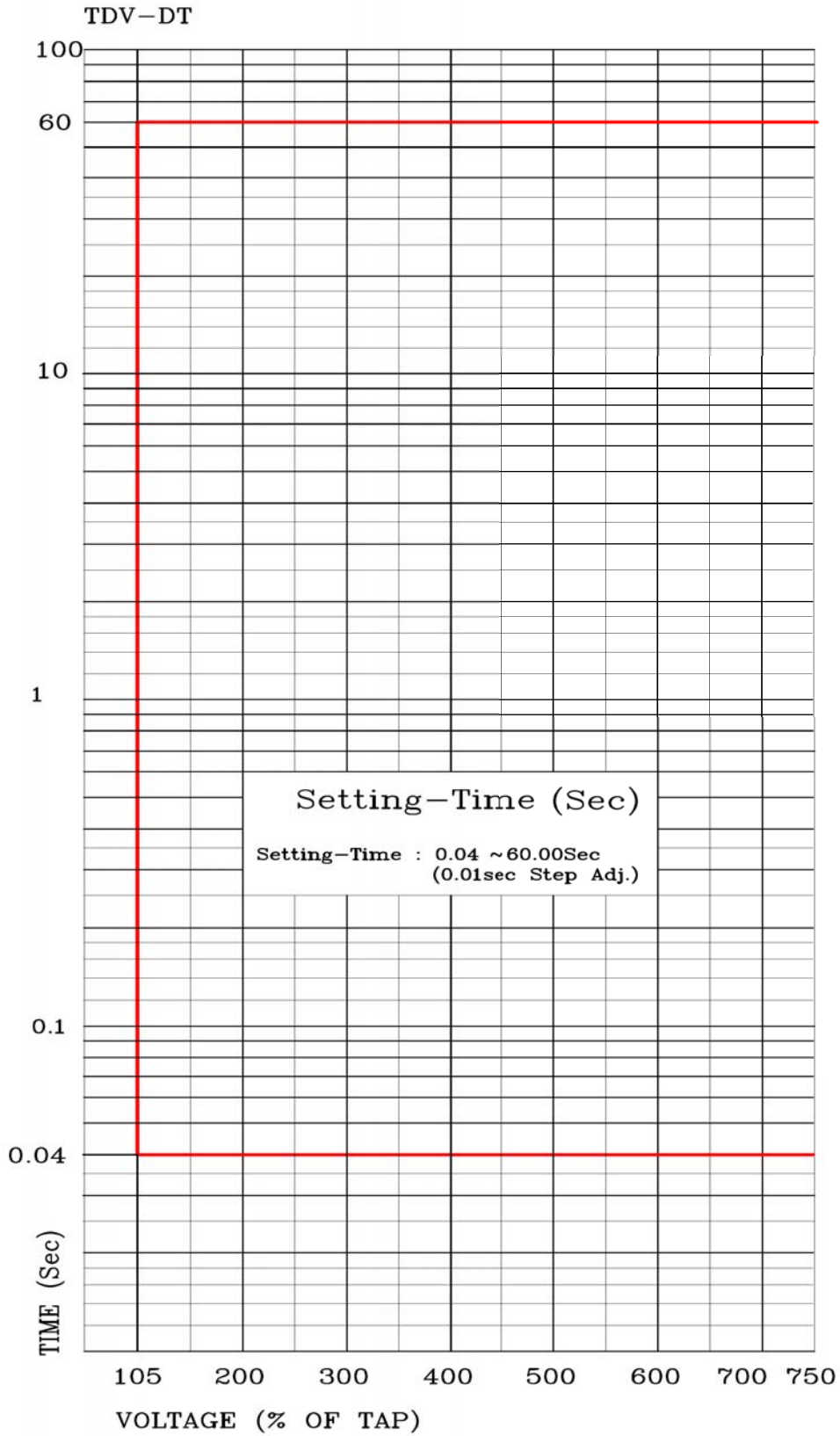
<부도 5.2 TDV 정한시 특성 곡선>
