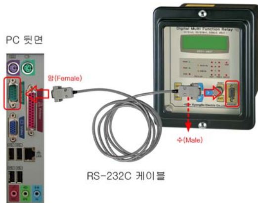
<Figure 4. RS-232C 연결>
