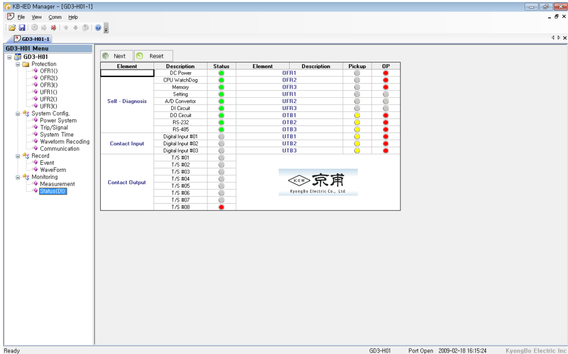
<Figure 17. GD3-H01 Status(DI)>
