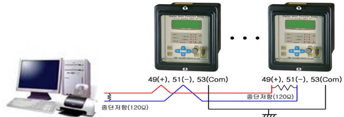
<Figure 5. RS-485C 결선도>
