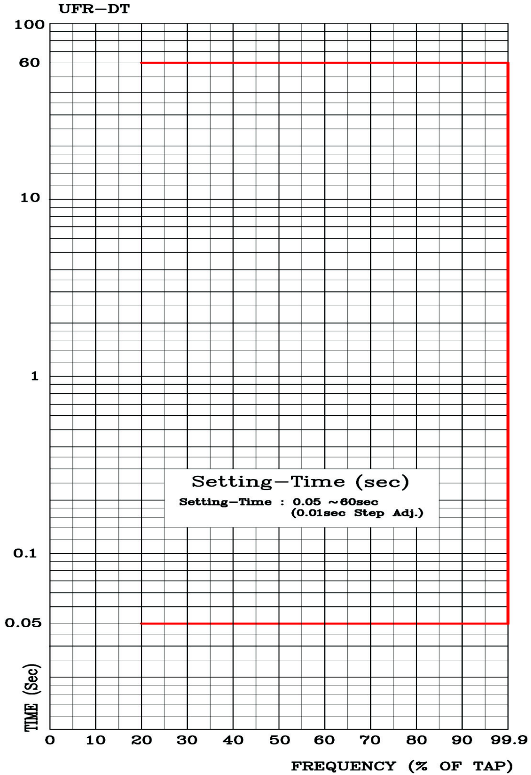
<부도 5.2 UFR 정한시 특성 곡선>
