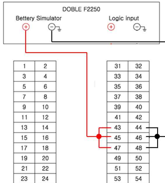
<그림 10. 계전기 Test 장비와 GD3-H11 결선도>
