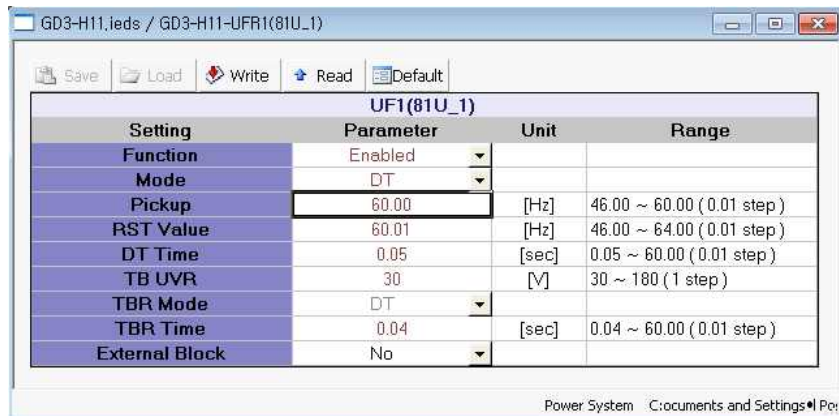
<그림 4. UFR 동작시간(최소) 설정>
