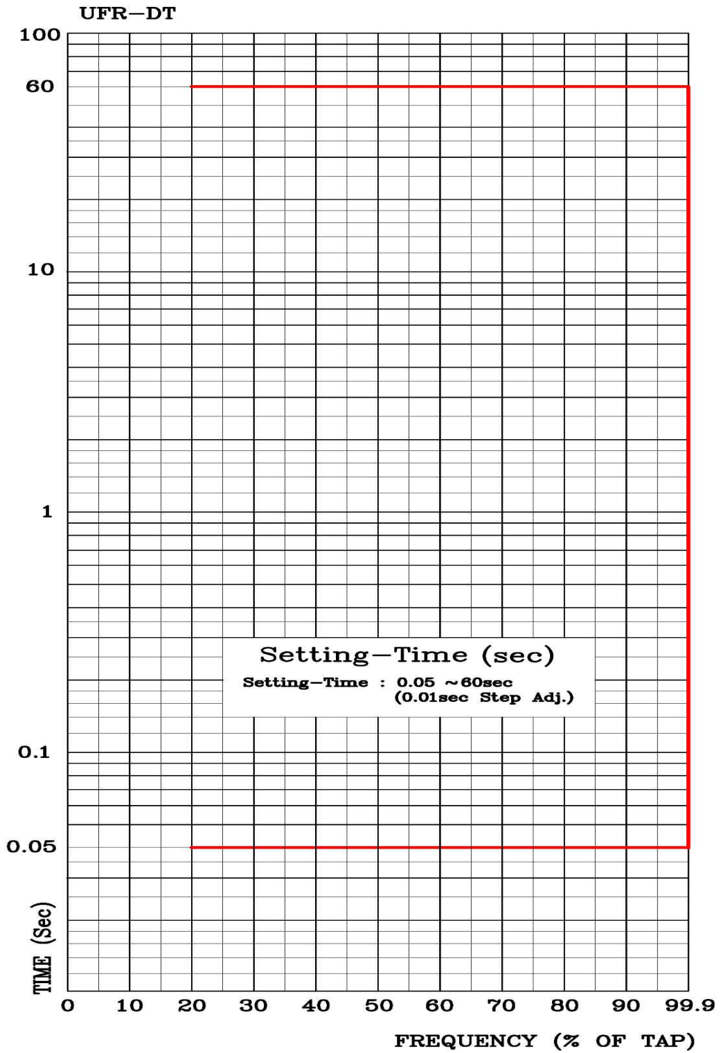
<부도 4.2 UFR 정한시 특성 곡선>
