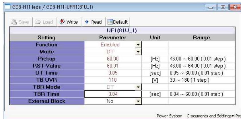
<그림 8. 저전압 Blocking 복귀시간 순시 설정>
