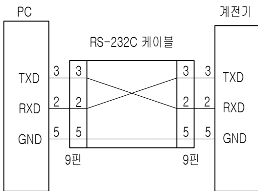
<Figure 3. RS-232C 회로도>
