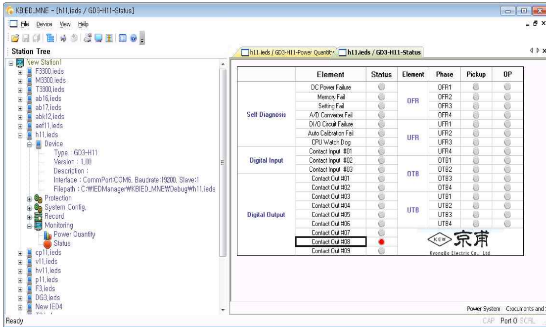
<Figure 26. Status>
