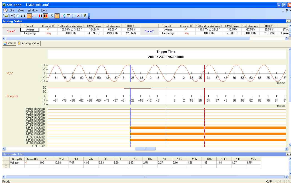
<Figure 29. KBCanes>
