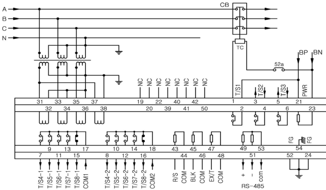
<부도 4. External Connection Diagram>
