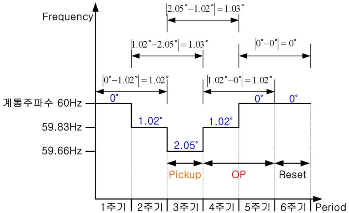
<Figure 5. VSR 동작, 복귀특성>
