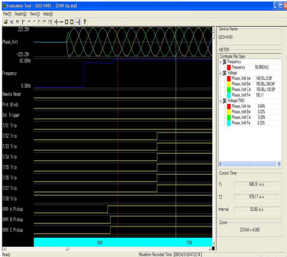
<Figure 21. GD3-HV01 Evaluation Tool>
