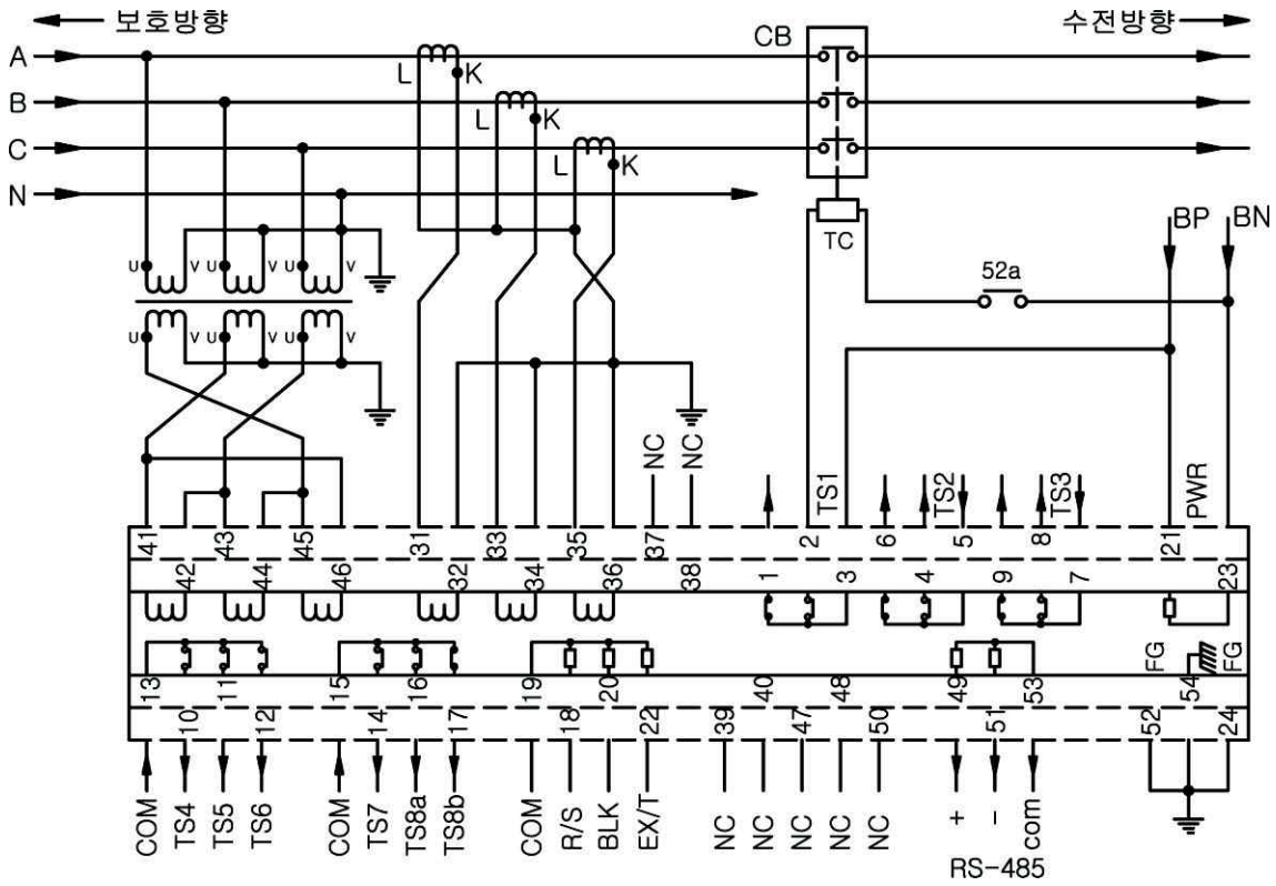
<부도 3.6 3상 4선식 External Connection Diagram>
