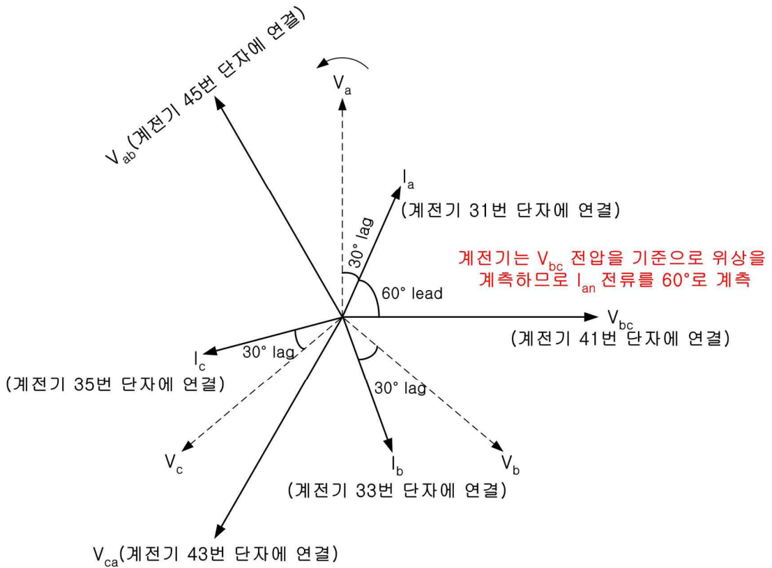
<Figure B.2.1 선간전압 입력 시 계전기 계측 표시 방법>
