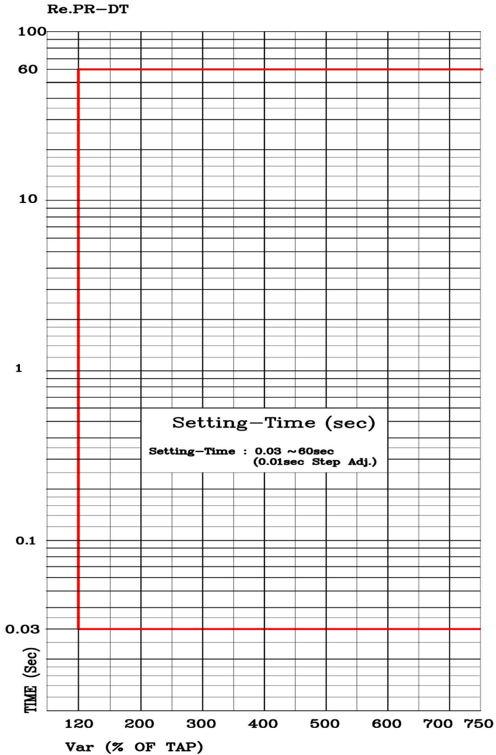
<부도 4.7 무효전력 요소 정한시 특성 곡선>
