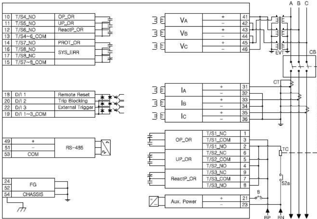
<부도 4.6 3상 4선식 External Connection Diagram>
