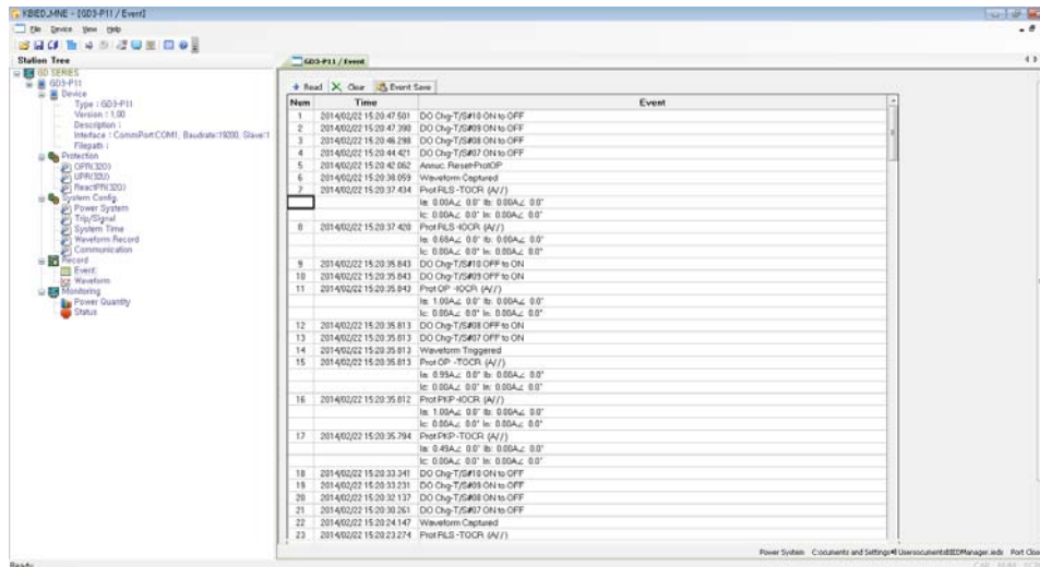
<Figure 27. Event>
