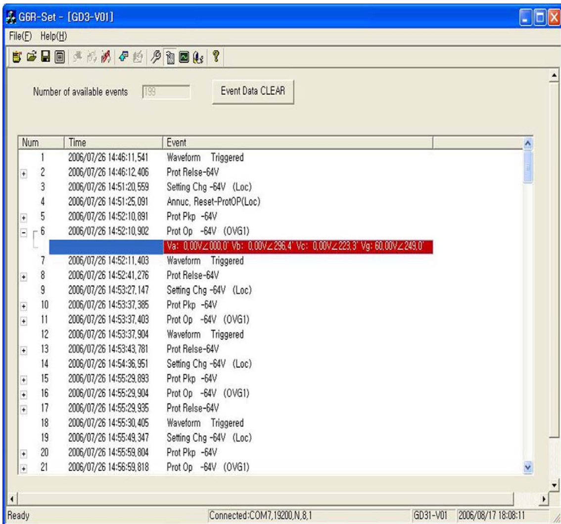
<Figure 17. GD3-V01 Event>
