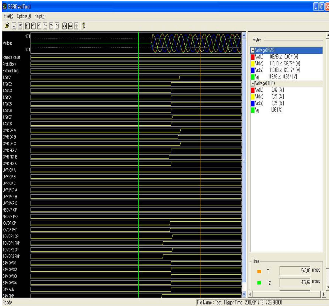
<Figure 20. GD3-V01 Fault Evaluation Tool>
