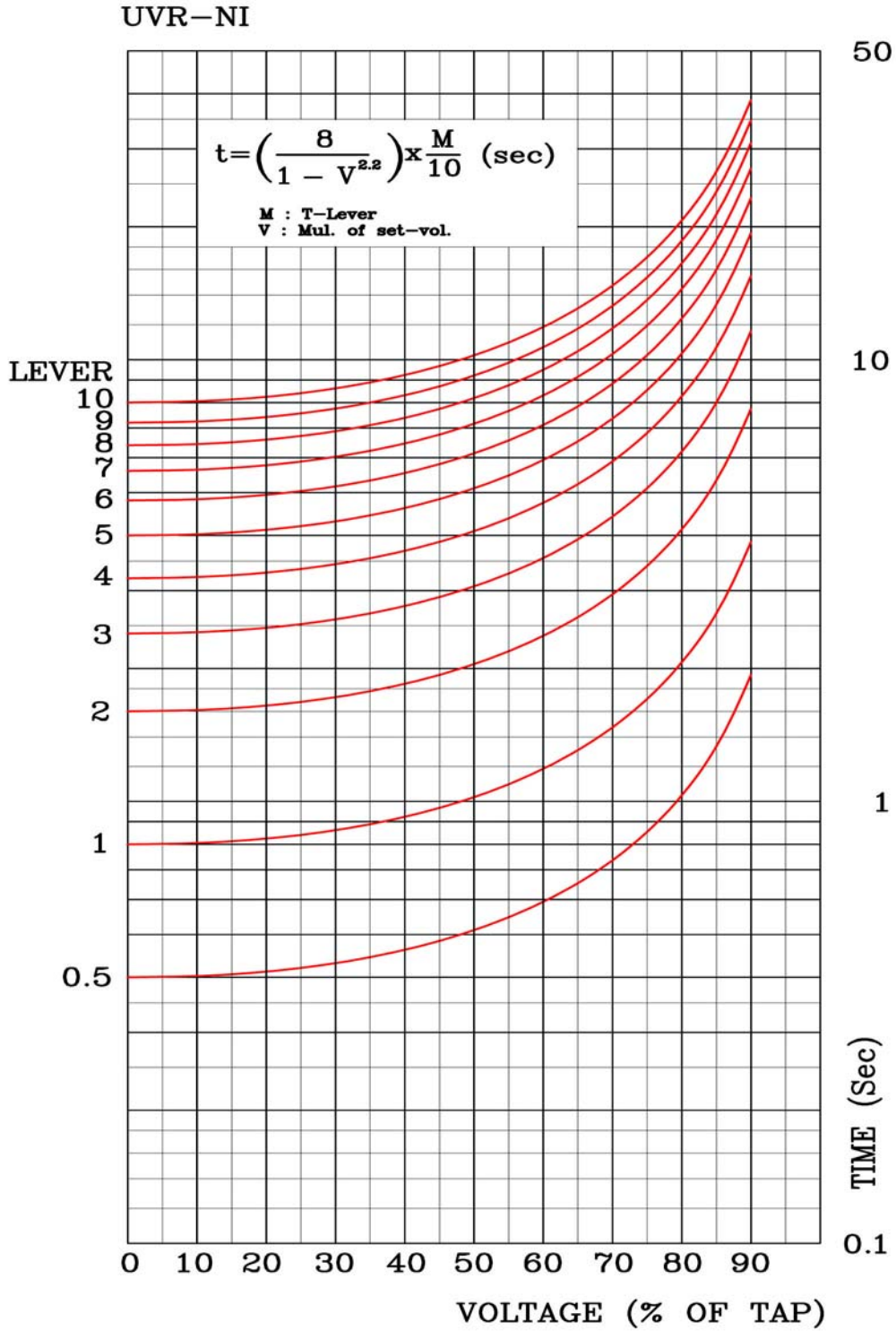
<부도 5.3 UVR 역반한시 특성 곡선>
