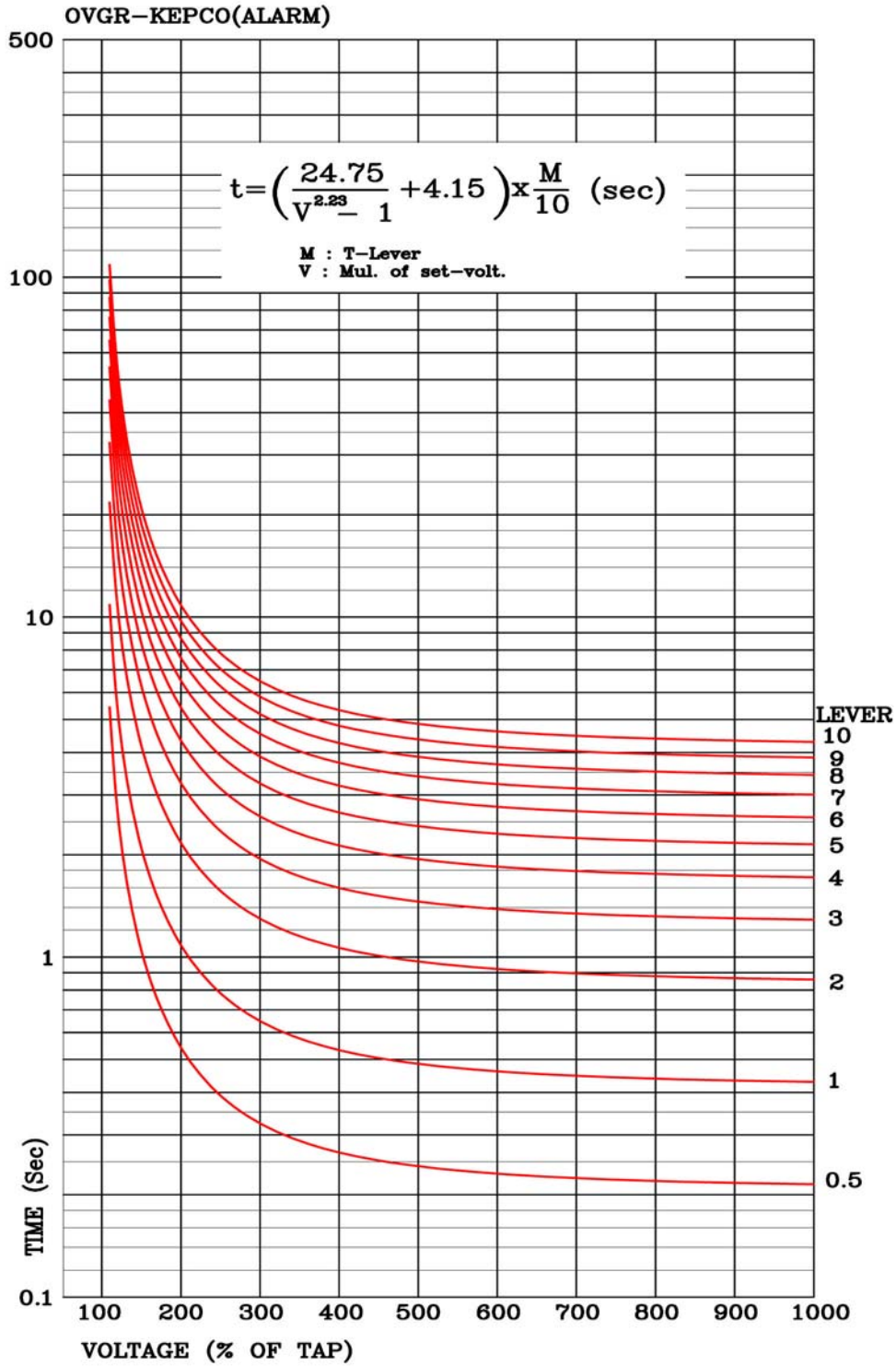
<부도 5.7 OVGR Alarm용 반한시 특성 곡선>
