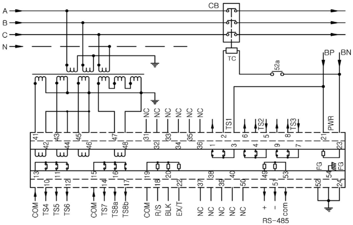
<부도 4.1 GPT 사용 시 외부 결선도>
