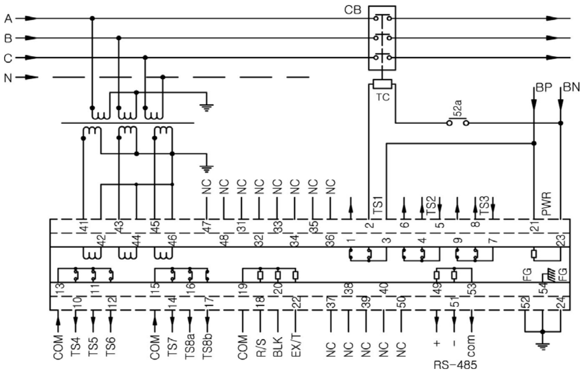
<부도 4.2 GPT 미사용 시 외부 결선도>
