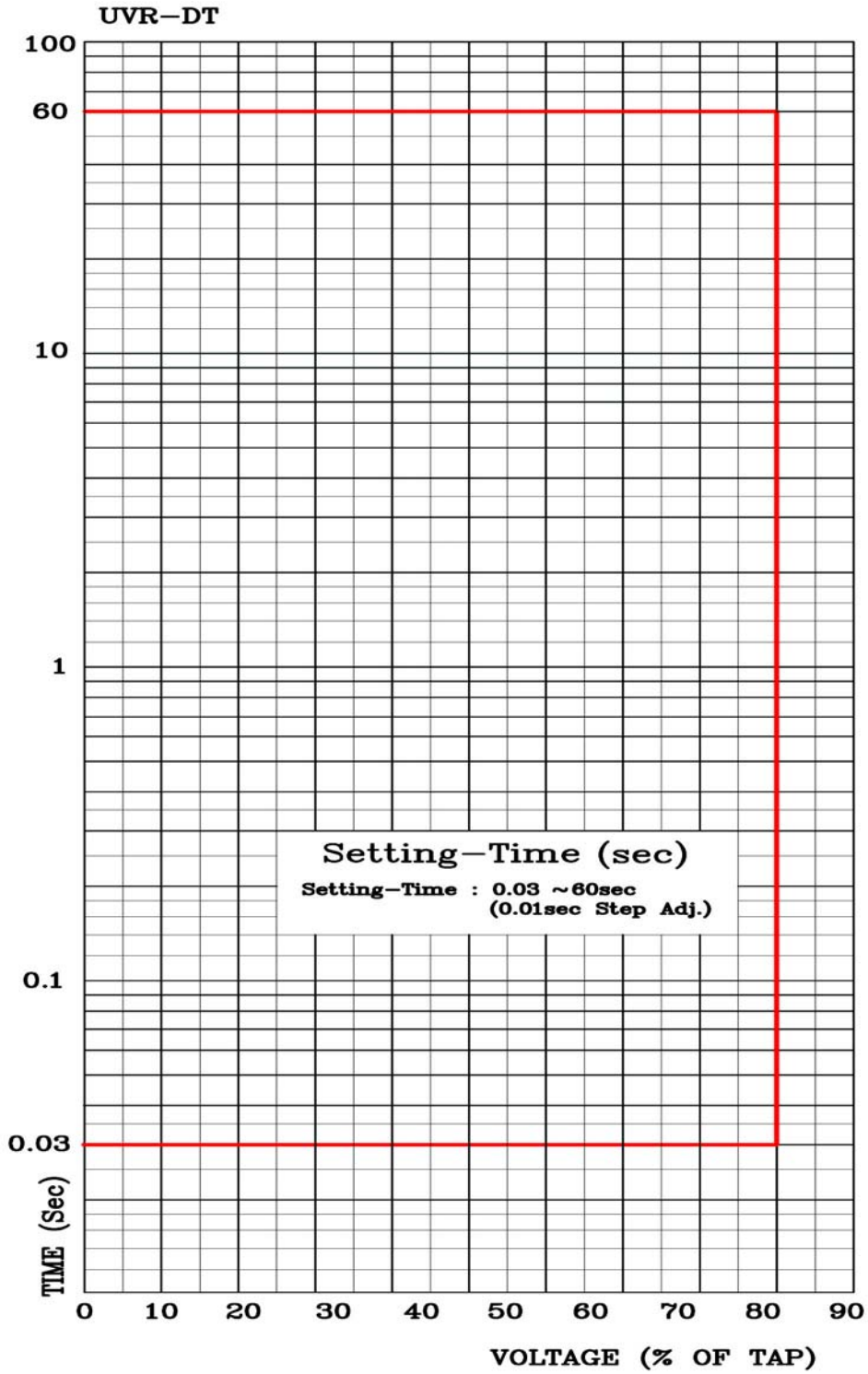
<부도 5.4 UVR 정한시 특성 곡선>
