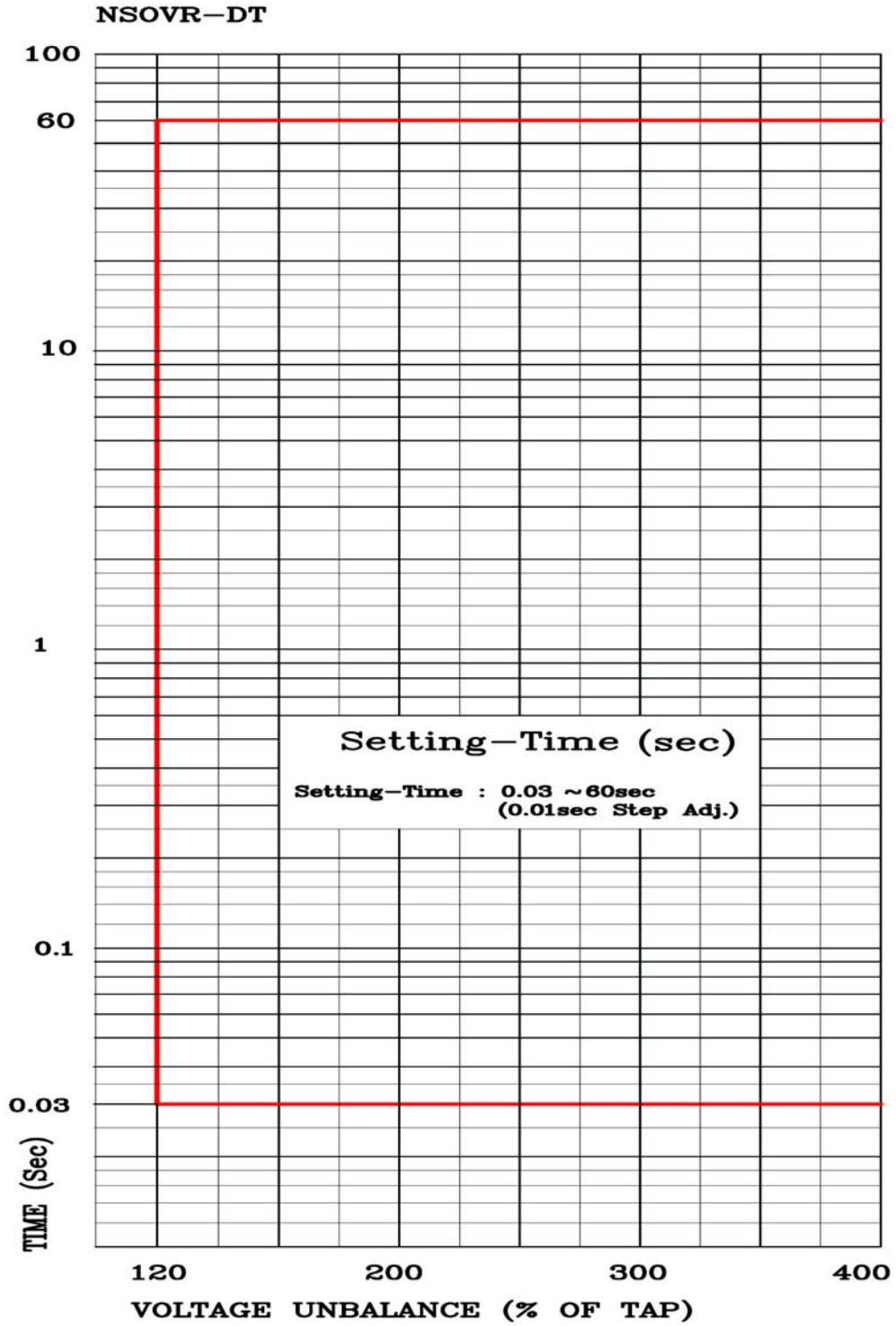
<부도 5.5 NSOVR 정한시 특성 곡선>
