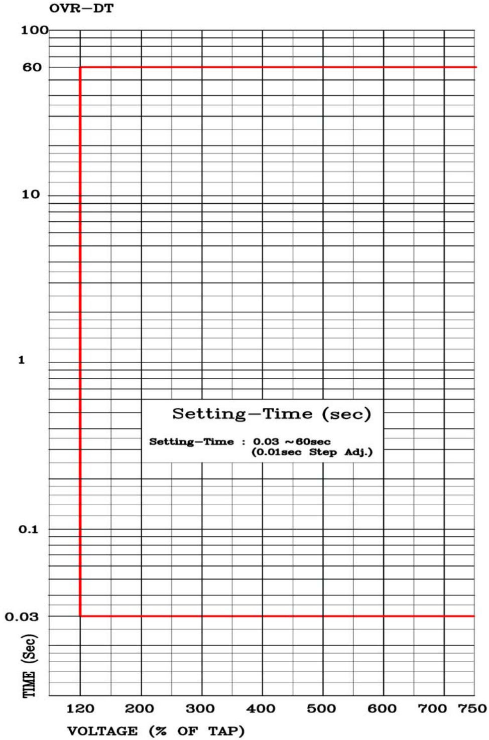
<부도 5.2 OVR 정한시 특성 곡선>
