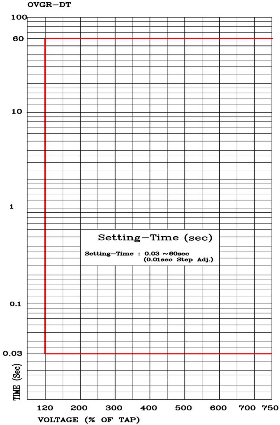
<부도 5.8 OVGR, 64V(OVG) 정한시 특성 곡선>
