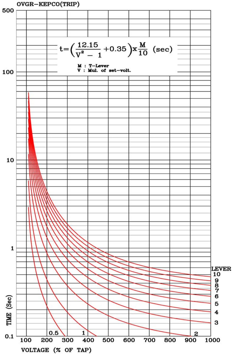
<부도 5.6 OVGR Trip용 반한시 특성 곡선>
