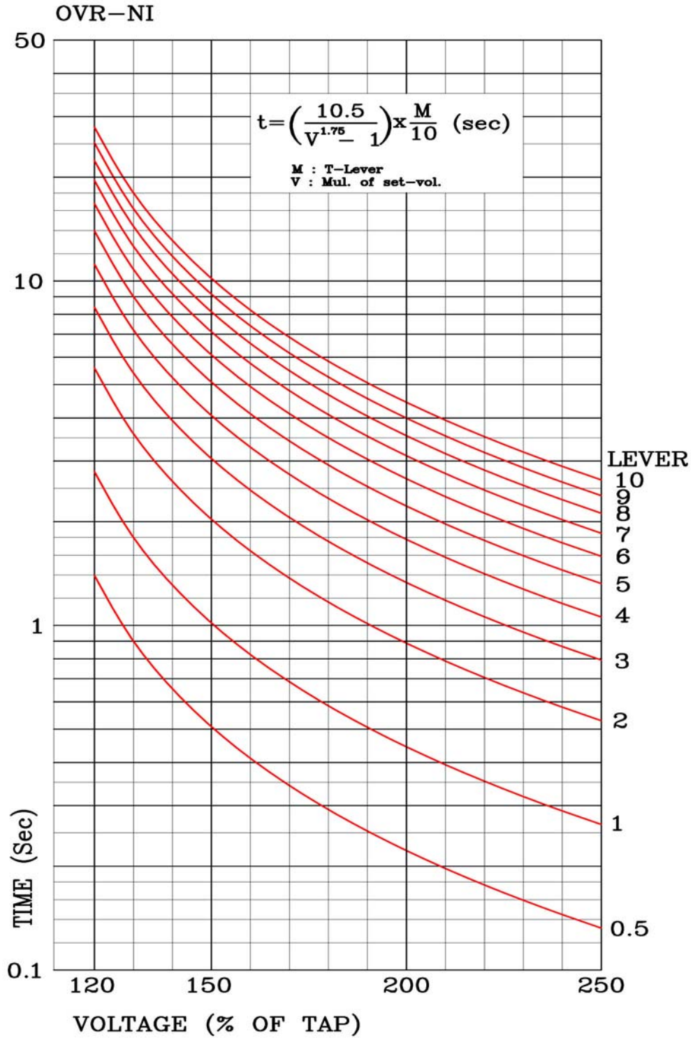
<부도 5.1 OVR 반한시 특성 곡선>
