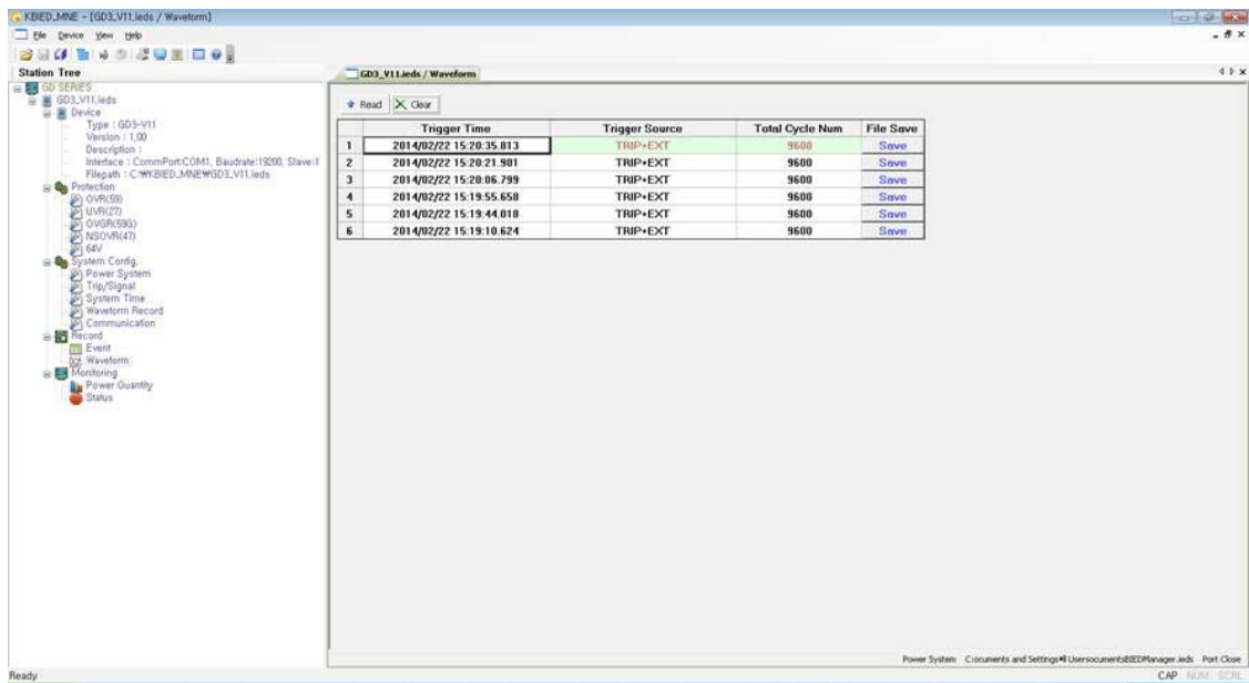
<Figure 28. WaveForm>
