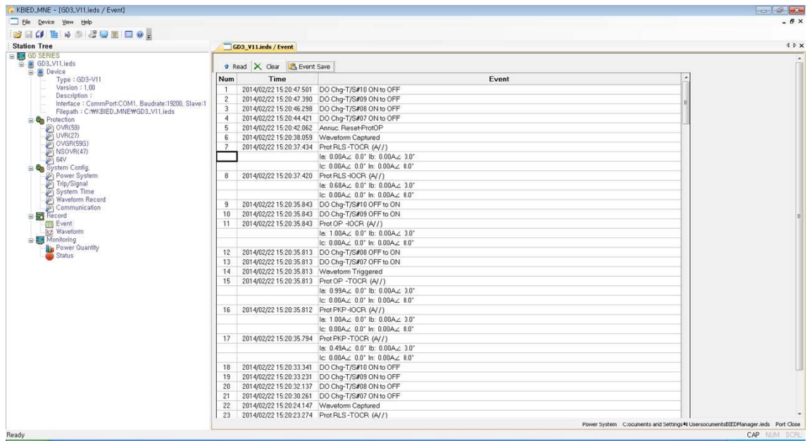
<Figure 27. Event>
