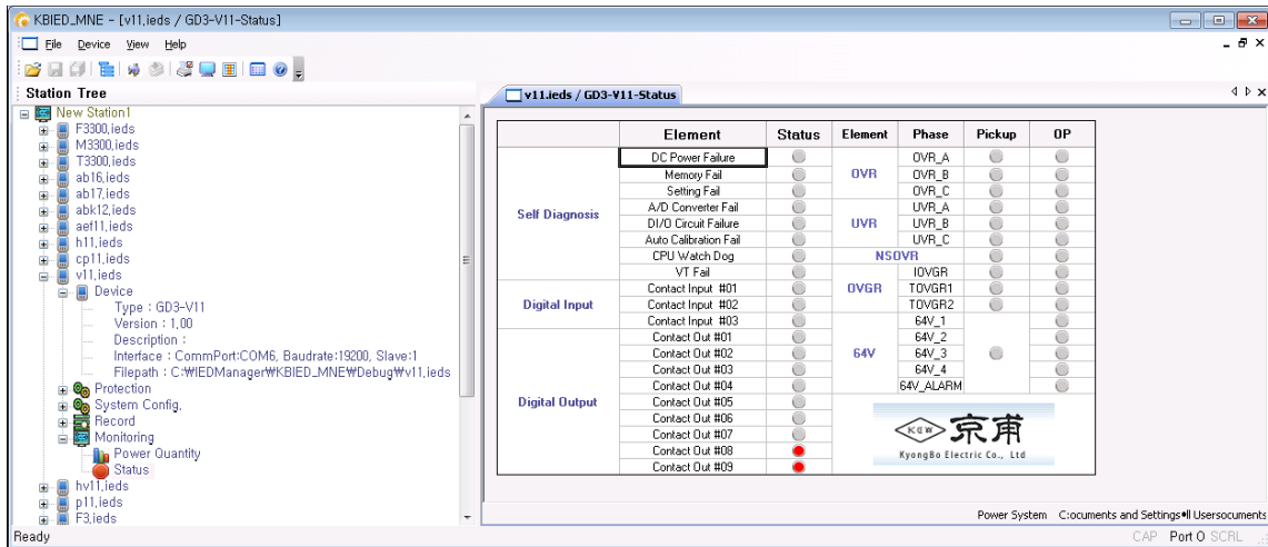
<Figure 30. Status>
