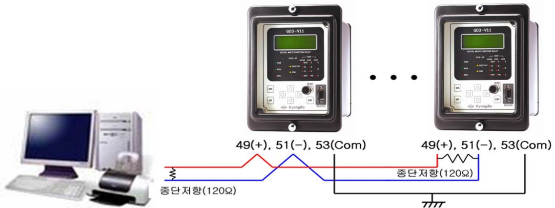
<Figure 9. RS-485 결선도>
