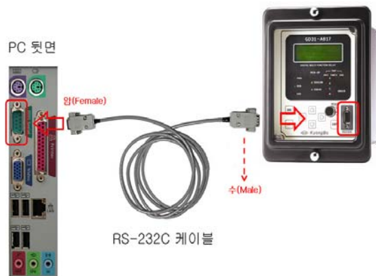
<Figure 8. RS-232C 연결>
