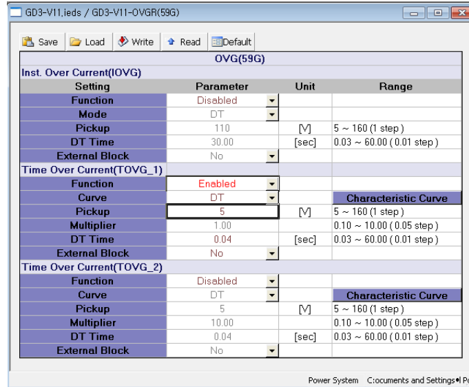
<그림 8. TOVGR1 동작치(최소) 설정>
