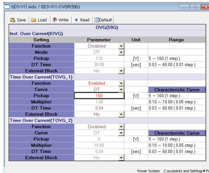
<그림 9. TOVGR1 동작치(최대) 설정>
