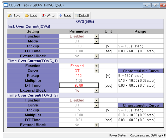
<그림 11. TOVGR1 정한시(최대) 설정>
