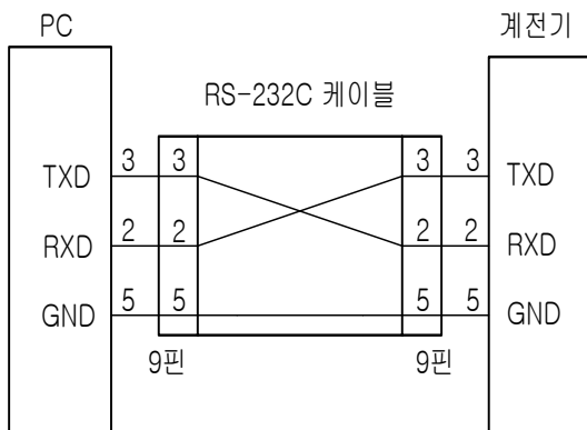
<Figure 7. RS-232C 회로도>
