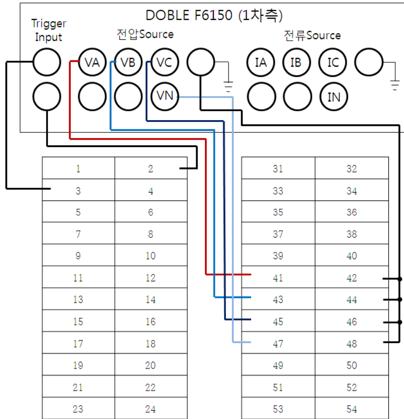
<그림 1. 계전기 Test 장비와 GD3-V11 결선도>
