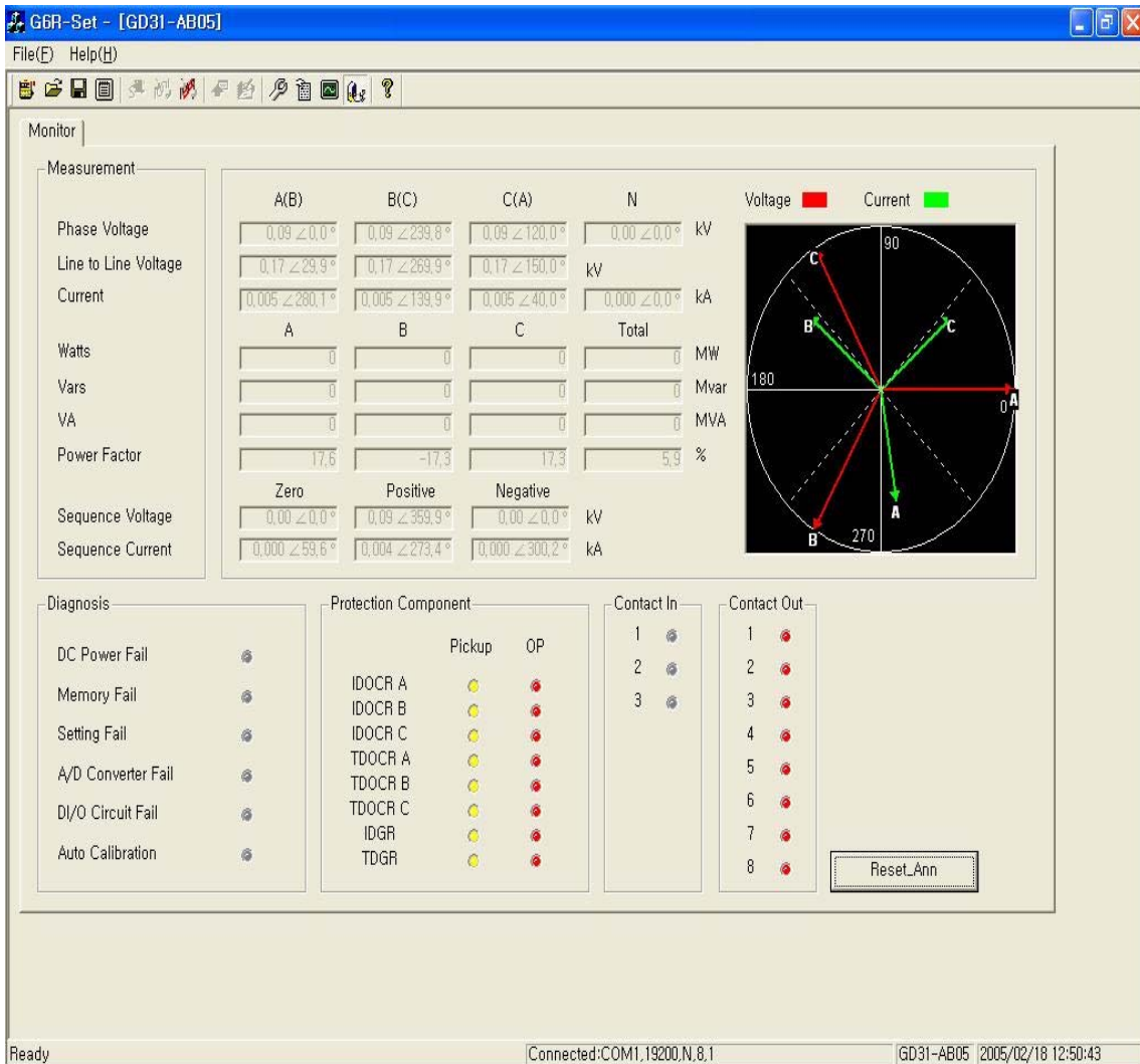
<Figure 20. GD31-AB05 Monitor>
