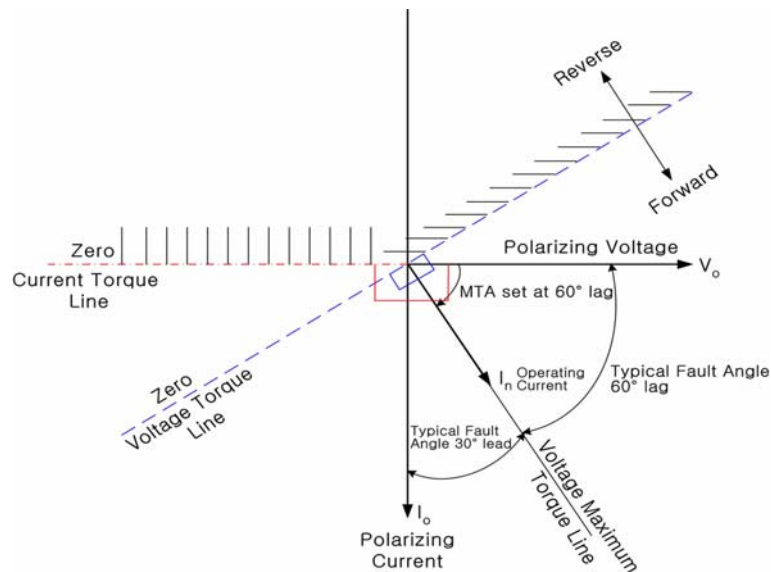
<Figure 5. 기준 극성을 Dual로 하였을 때의 동작 특성>
