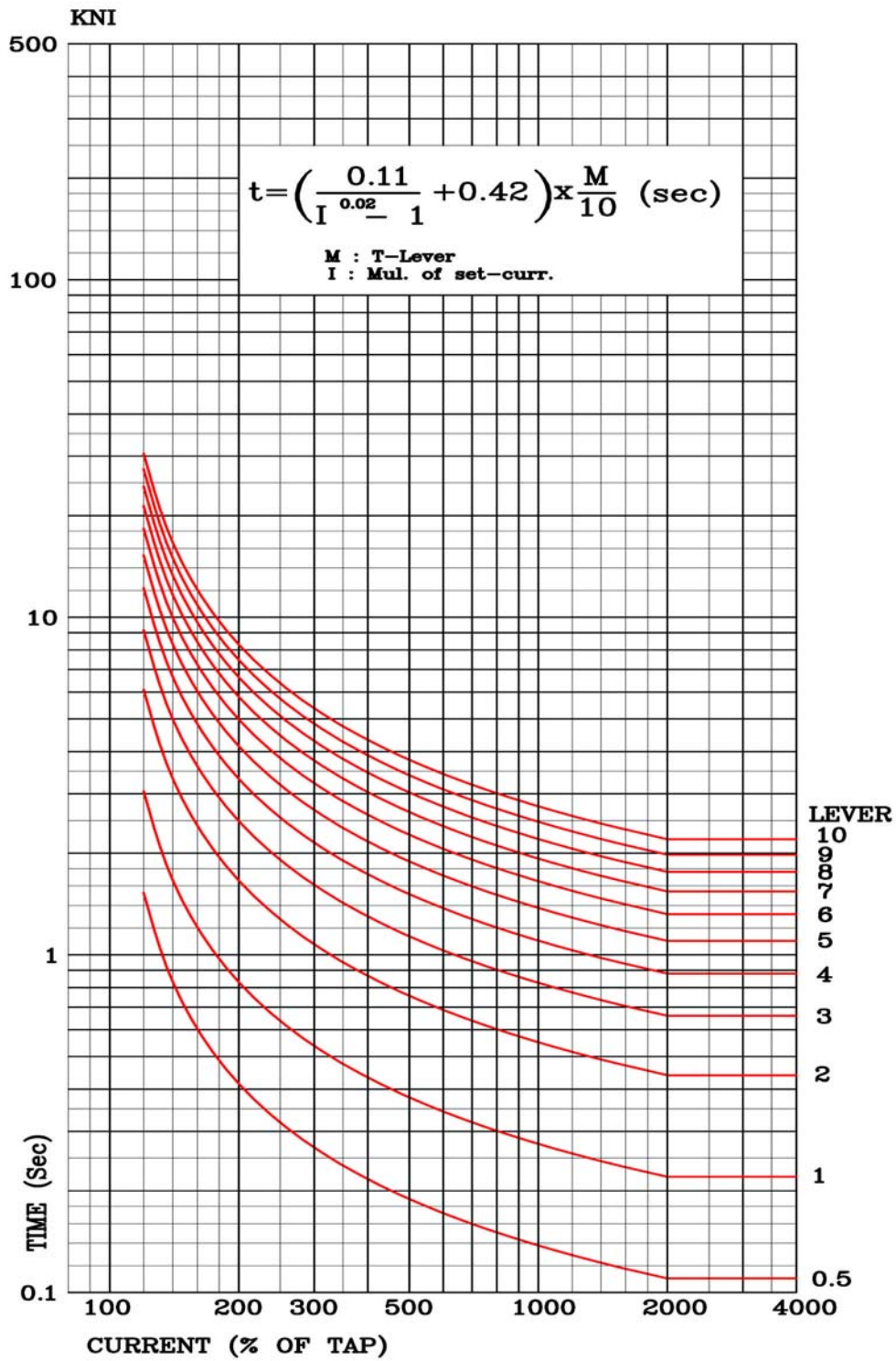
<부도 5.5 경보유도형 (KEPCO형) 반한시 특성 곡선>
