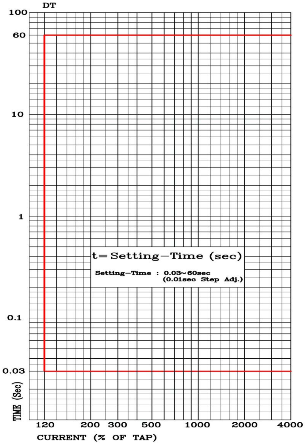
<부도 5.8 정한시 특성 곡선>
