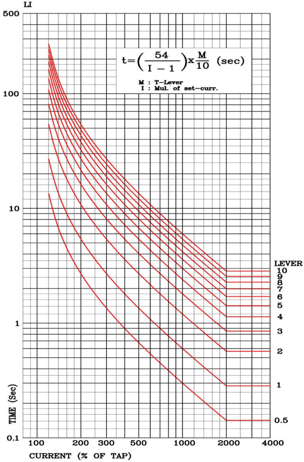
<부도 5.3 장반한시 특성 곡선>
