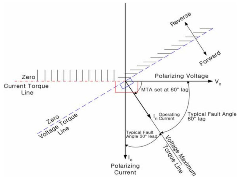
<Figure 5. 기준 Polarizing을 Dual로 하였을 때의 동작 특성>
