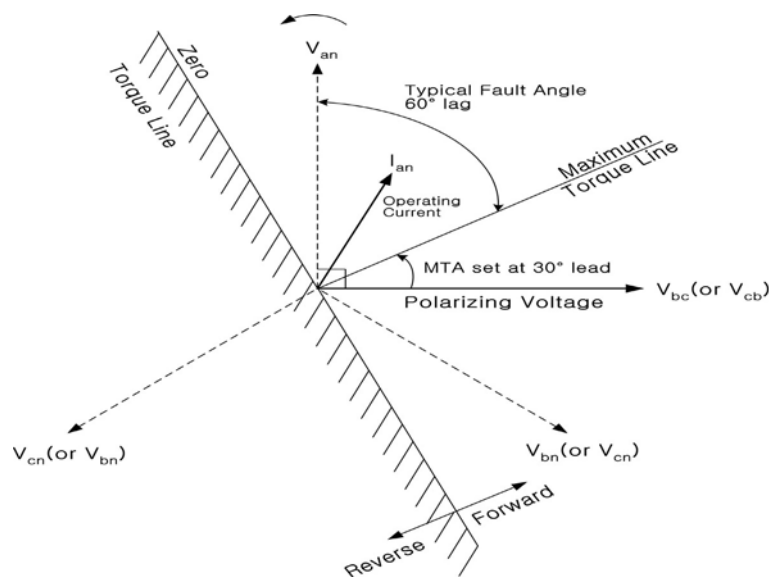
<Figure 2. A상 전류의 동작 특성>
