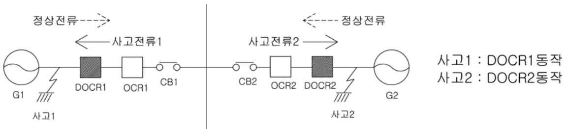
<Figure 1. DOCR 설치 위치>
