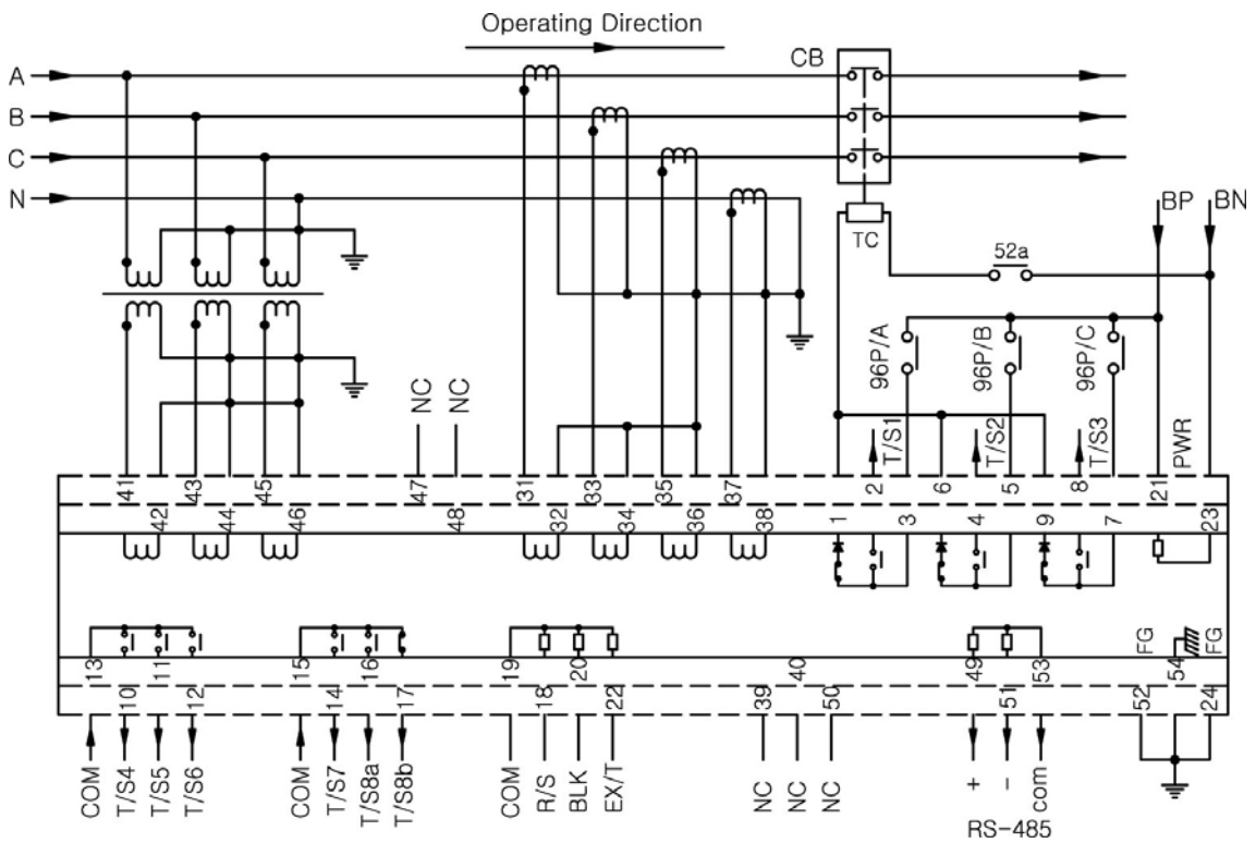
<부도 4.2 GPT 미사용 시 외부 결선도>
