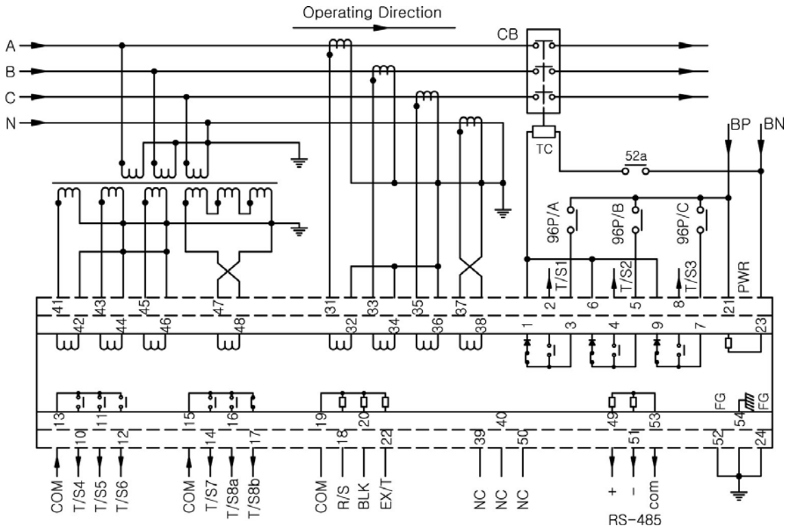
<부도 4.1 GPT 사용 시 외부 결선도>
