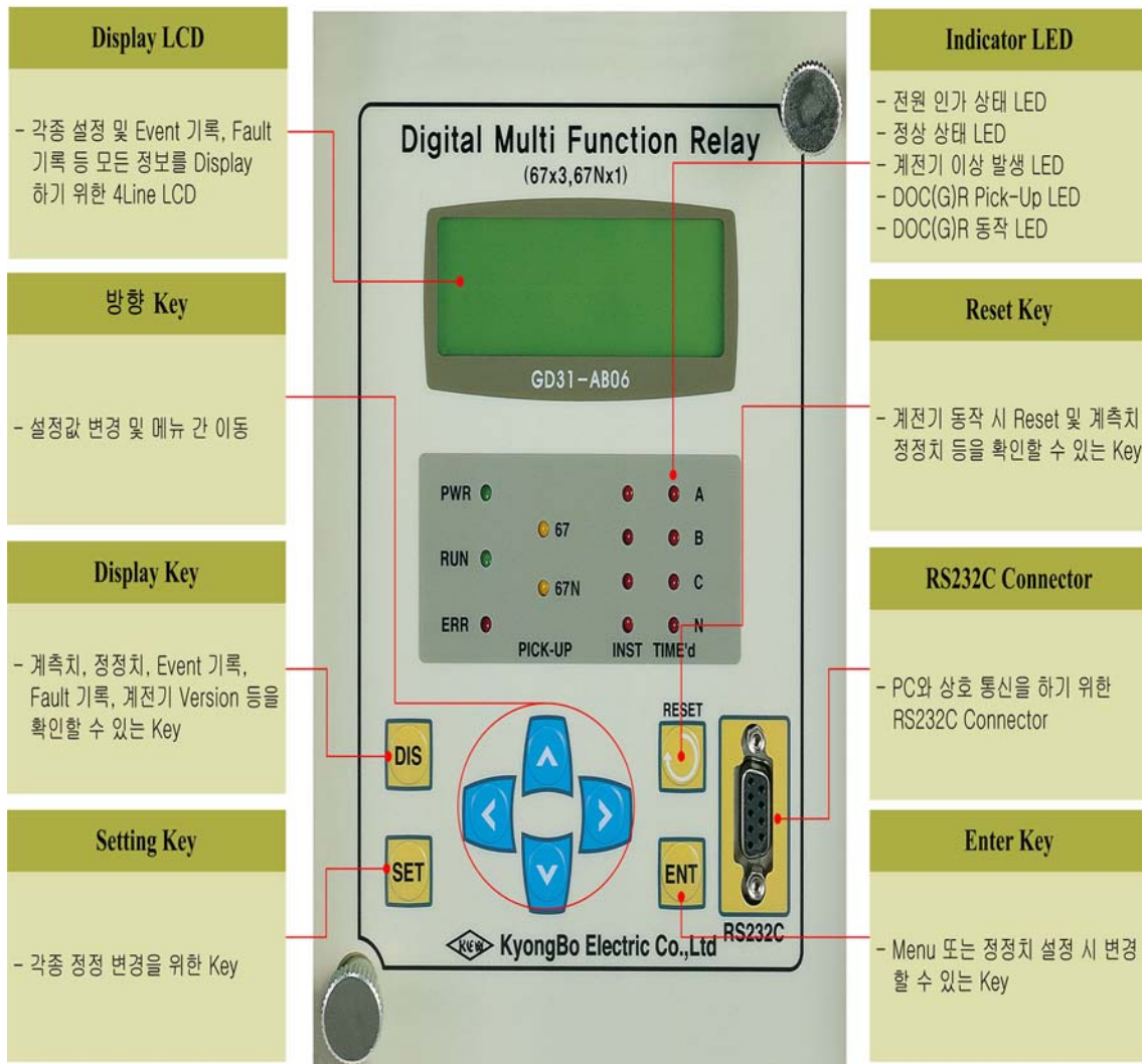
<Figure 8. 전면 표시부>
