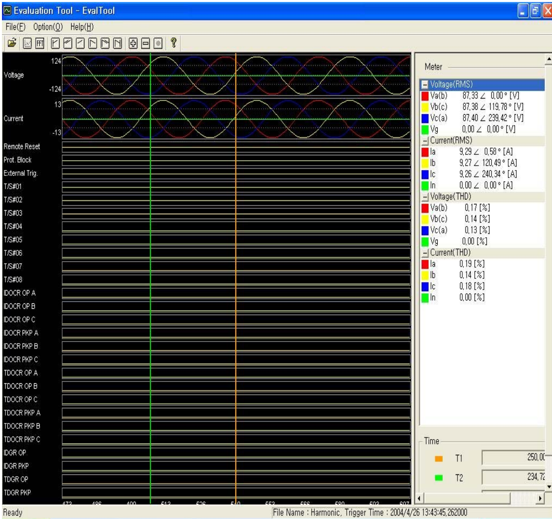
<Figure 18. GD31-AB06 Fault Evaluation Tool>
