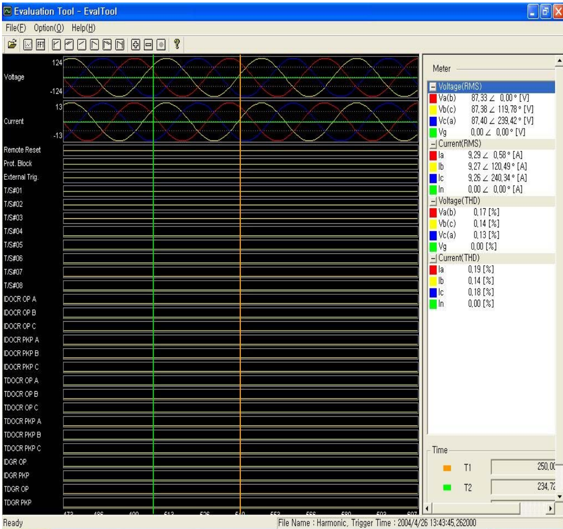
<Figure 21. GD31-AB06 Fault Evaluation Tool>
