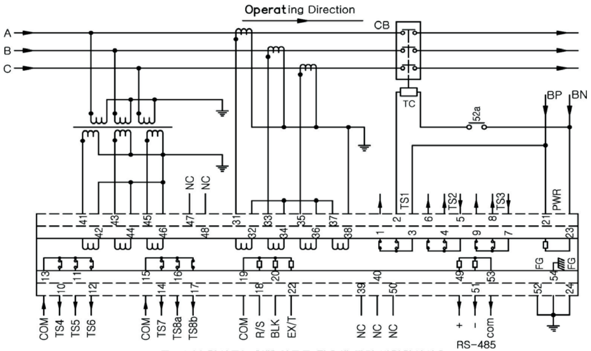
<부도 3.1 GPT 미사용 시 외부 결선도>
