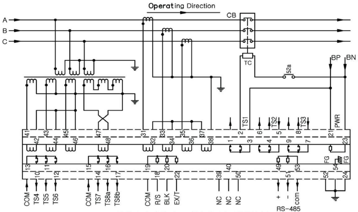
<부도 3.2 GPT 사용 시 외부 결선도>
