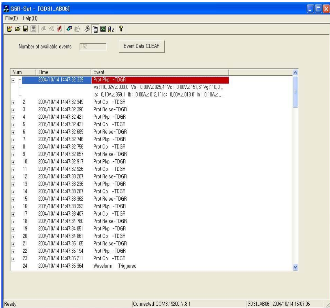
<Figure 18. GD31-AB06 Event>
