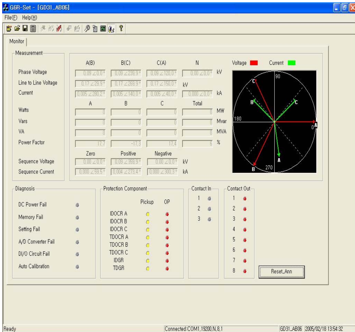
<Figure 20. GD31-AB06 Monitor>
