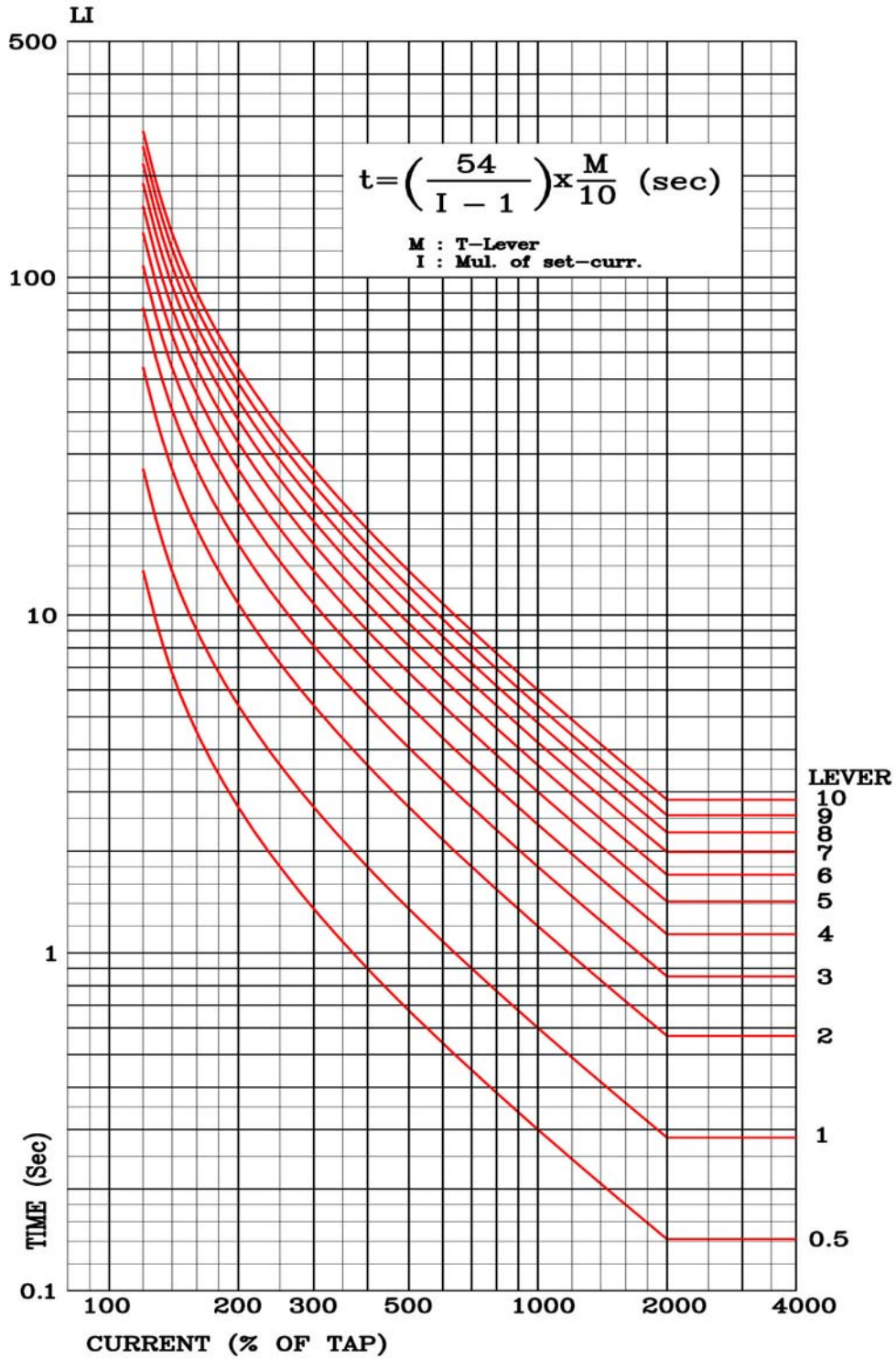
<부도 4.3 장반한시 특성 곡선>
