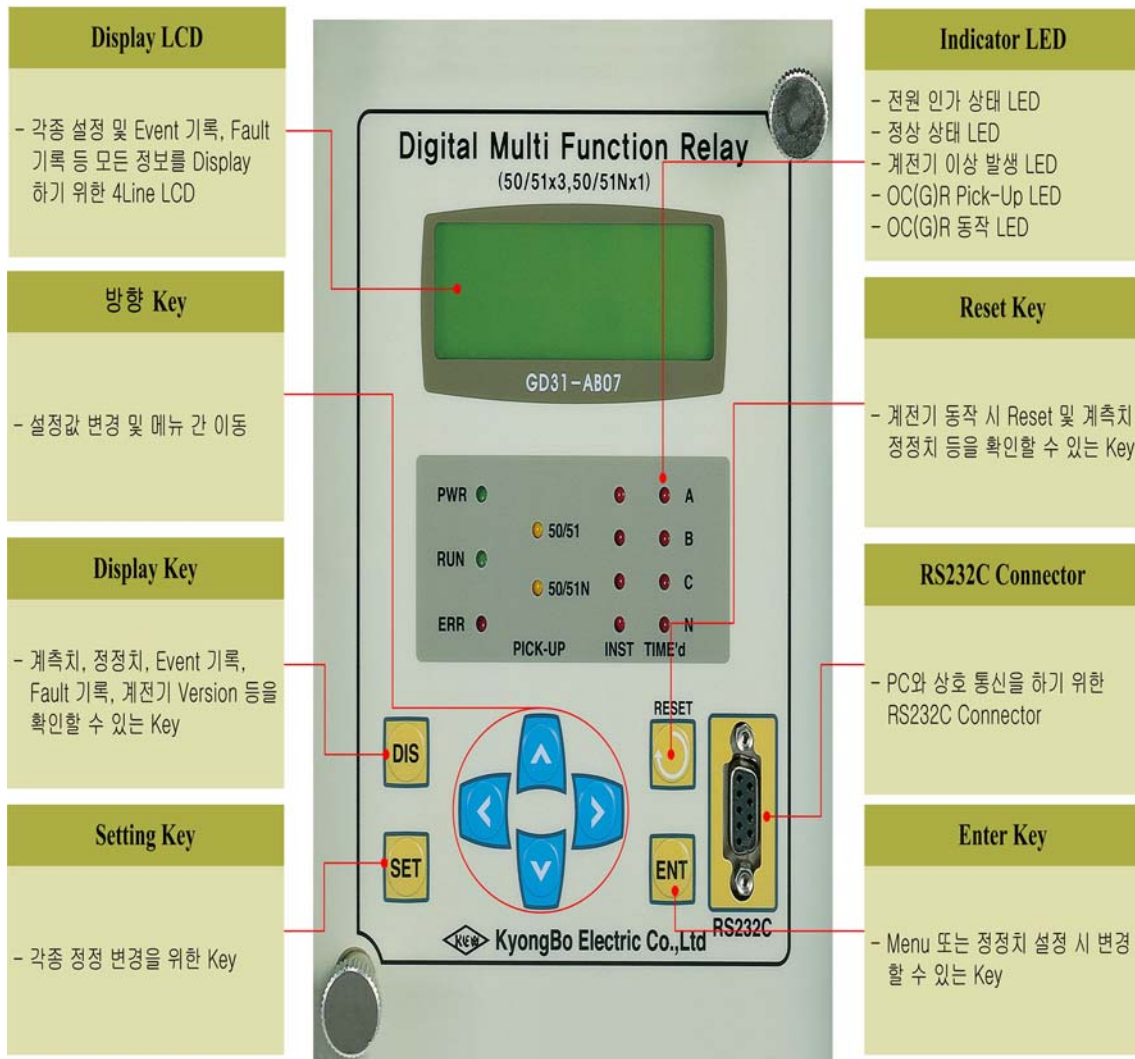
<Figure 5. 전면 표시부>
