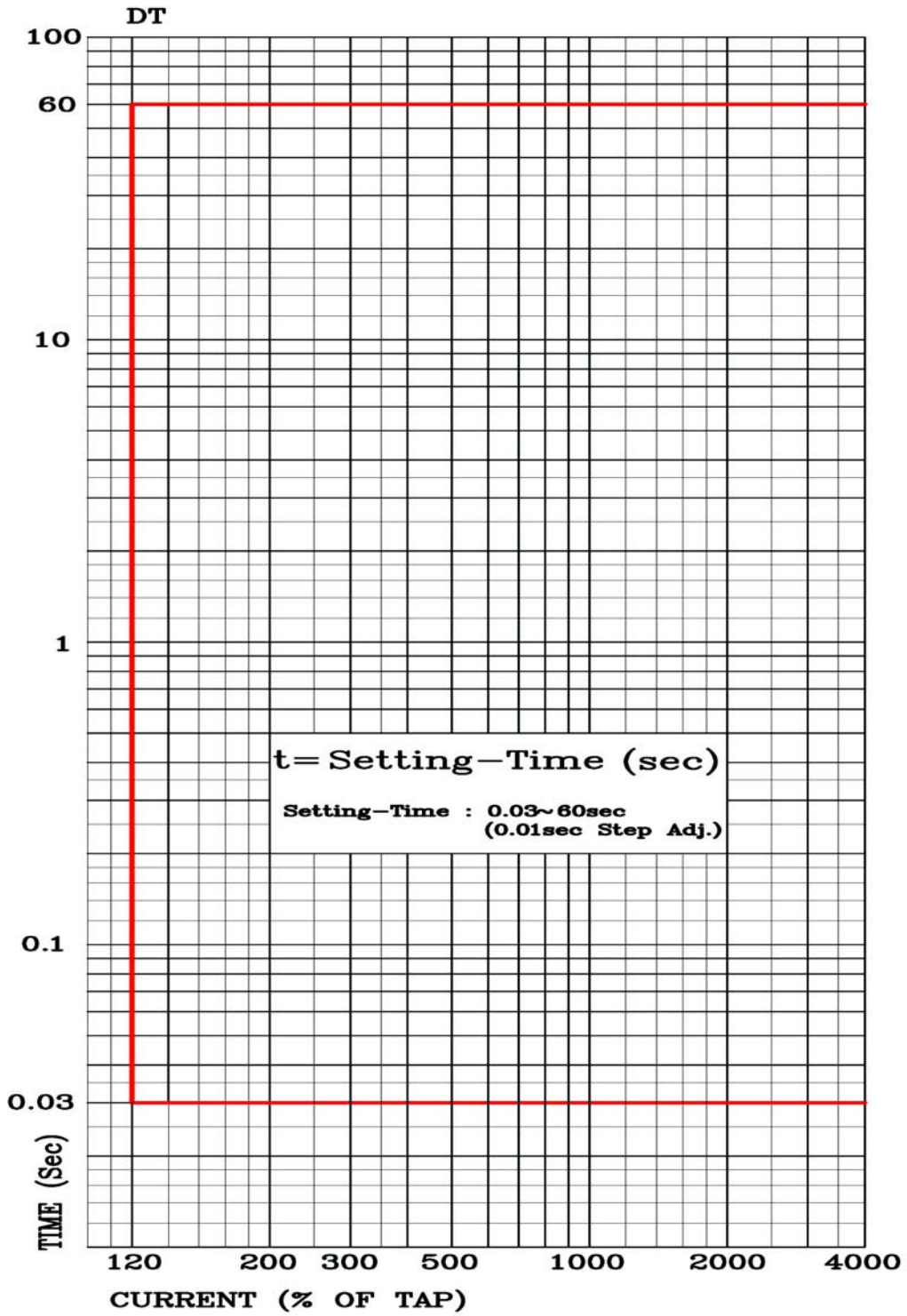
<부도 4.8 정한시 특성 곡선>
