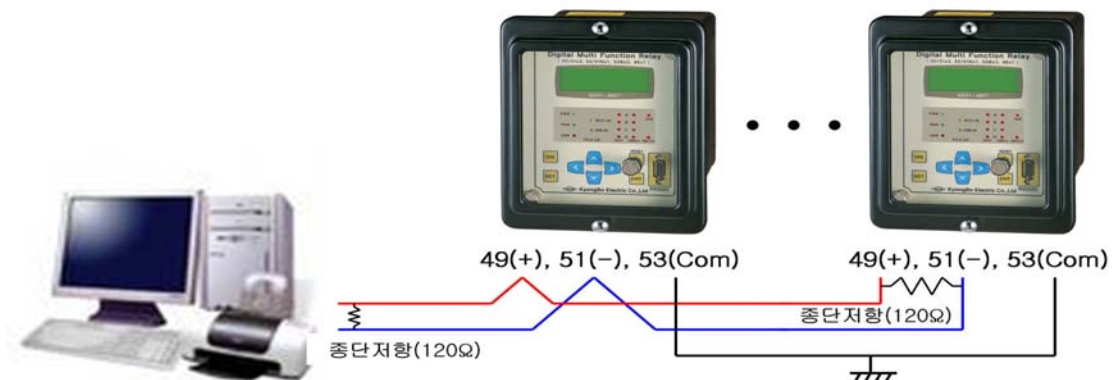
<Figure 8. RS-485C 결선도>
