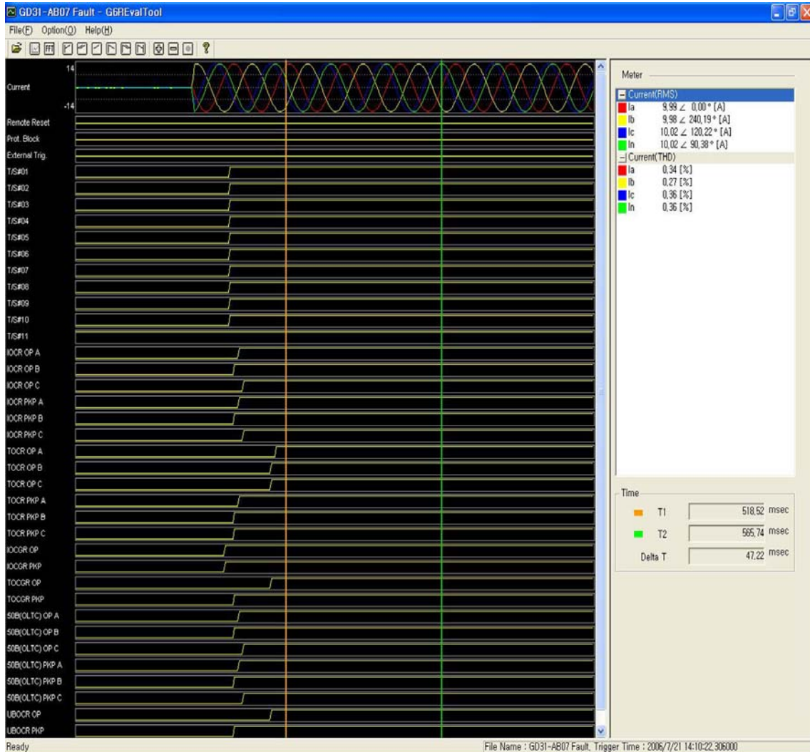
<Figure 19. GD31-AB07 Fault Evaluation Tool>
