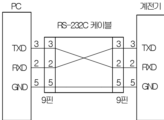
<Figure 7. RS-232C 회로도>
