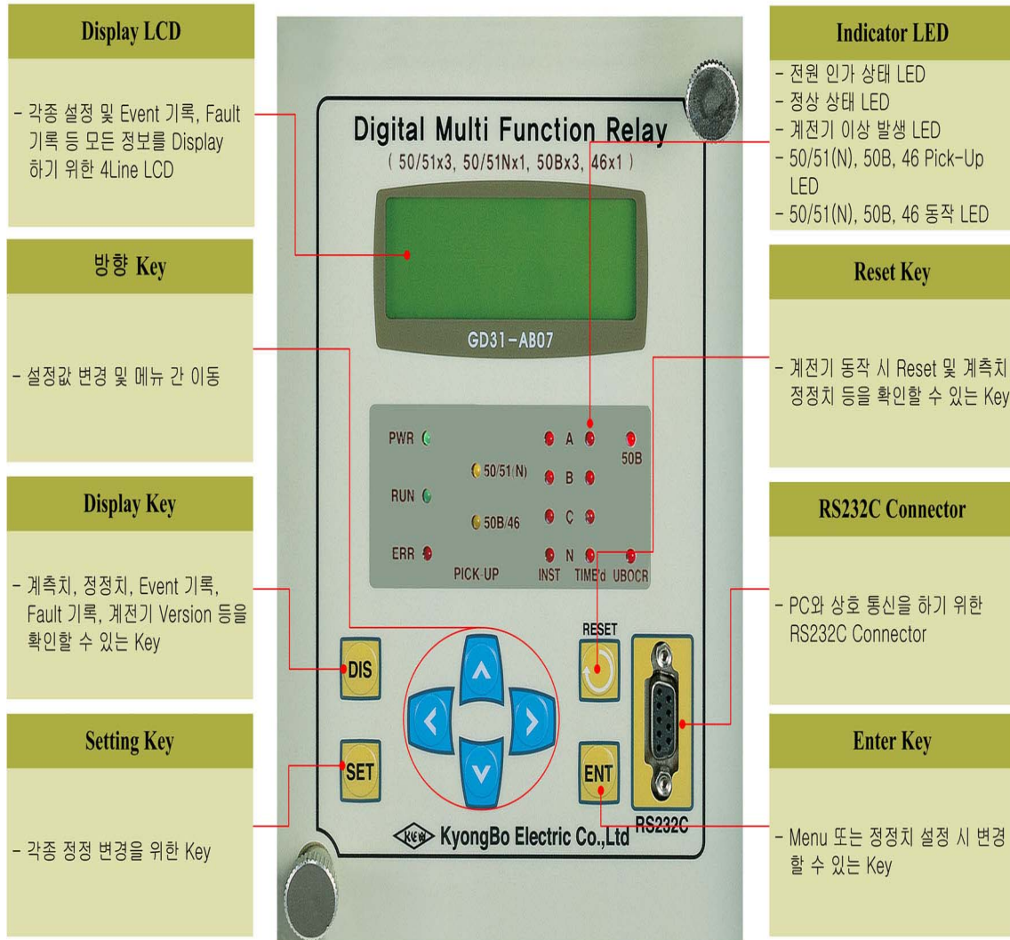
<Figure 10. 전면 표시부>
