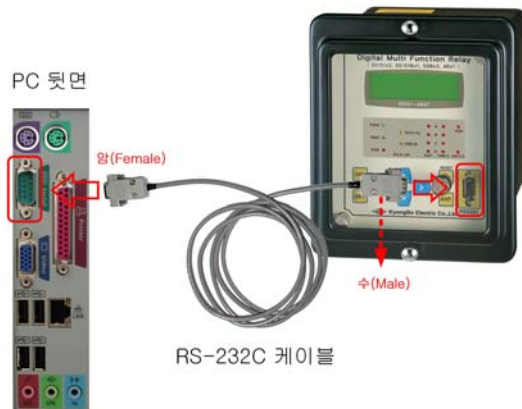
<Figure 8. RS-232C 연결>
