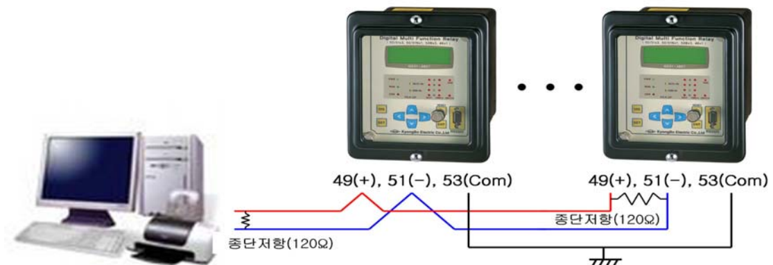
<Figure 9. RS-485C 결선도>
