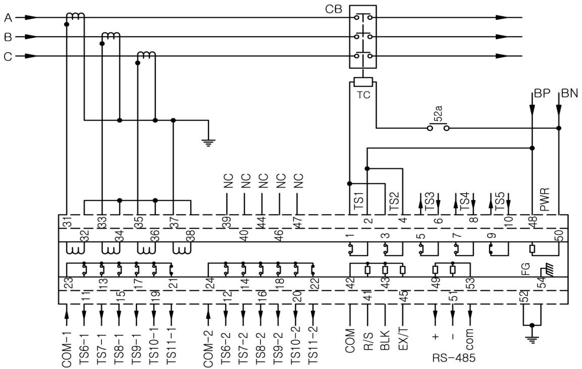
<부도 5. 한전 23kV D/L 보호 외부 결선도>
