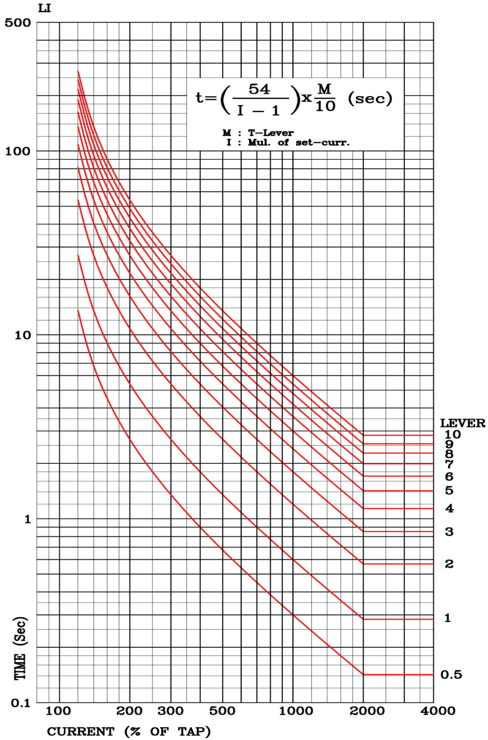
<부도 6.3 장반한시 특성 곡선>
