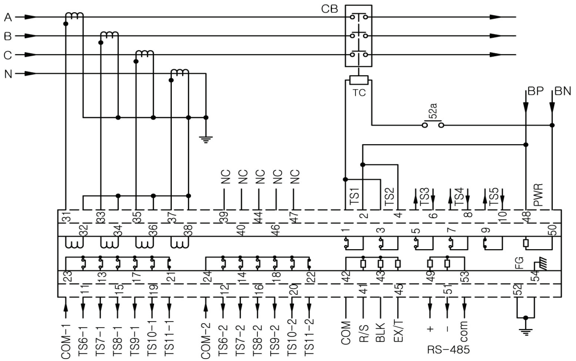
<부도 4. 한전 154kV 변압기 보호 51S 외부 결선도>
