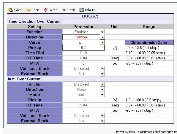
<그림 2. TDOCR 동작치(최소) 설정>
