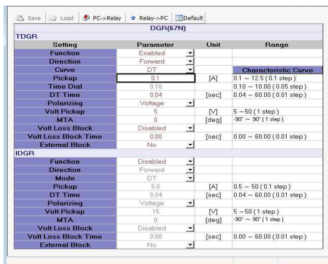
<그림 7. TDGR 동작치 설정>
