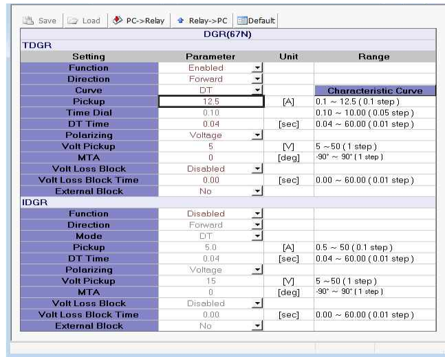
<그림 8. TDGR 동작치 설정>
