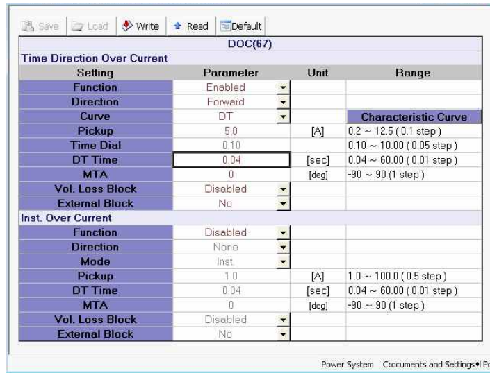
<그림 4. DOCR 정한시(최소) 설정>
