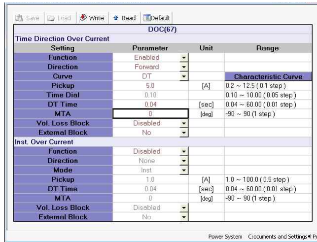
<그림 6. DOCR 동작위상 설정>
