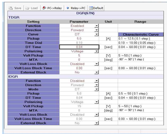
<그림 9. TDGR 동작시간 설정>
