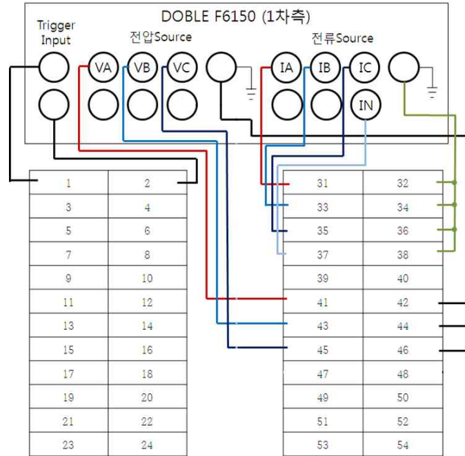
<그림 1. 계전기 Test 장비와 GD31-AB15 결선도>
