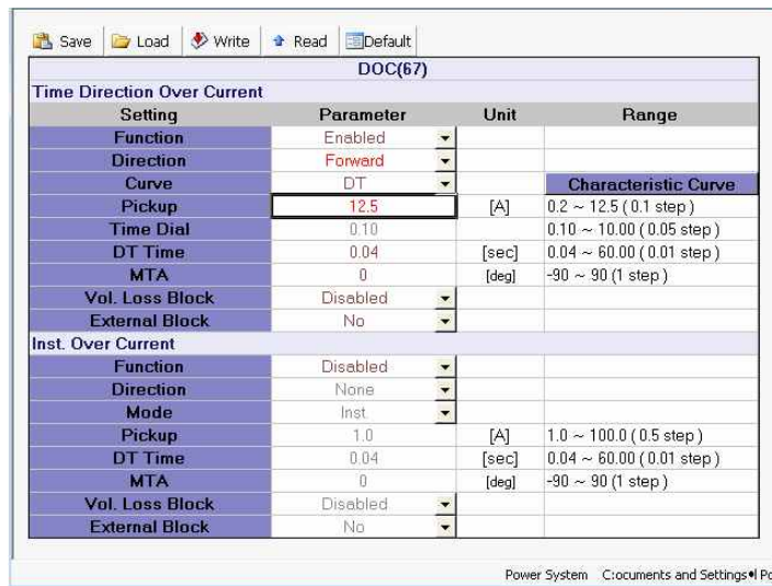
<그림 3. DOCR 동작치(최대) 설정>
