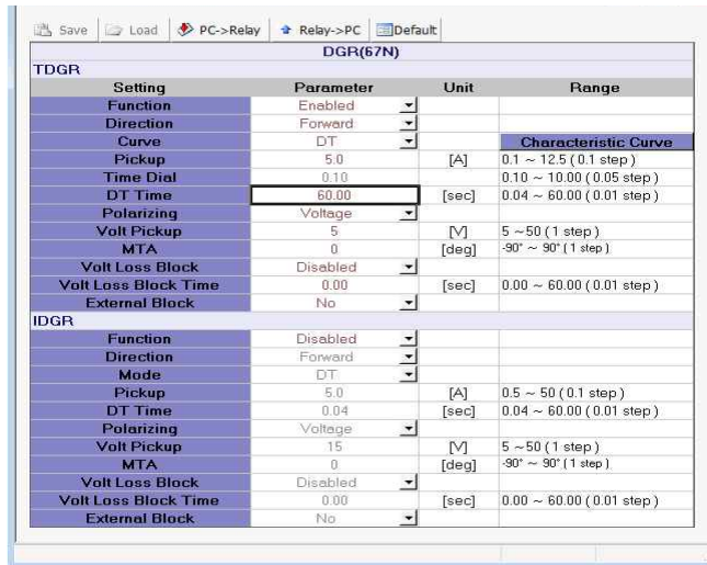
<그림 10. TDGR 동작시간 설정>
