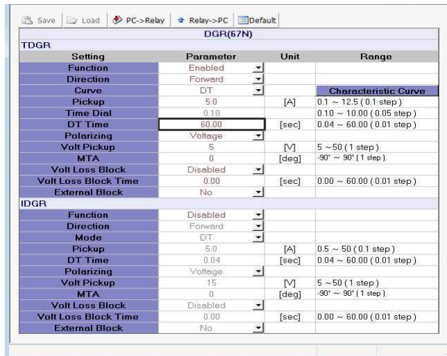
<그림 11. DGR 동작위상 설정>
