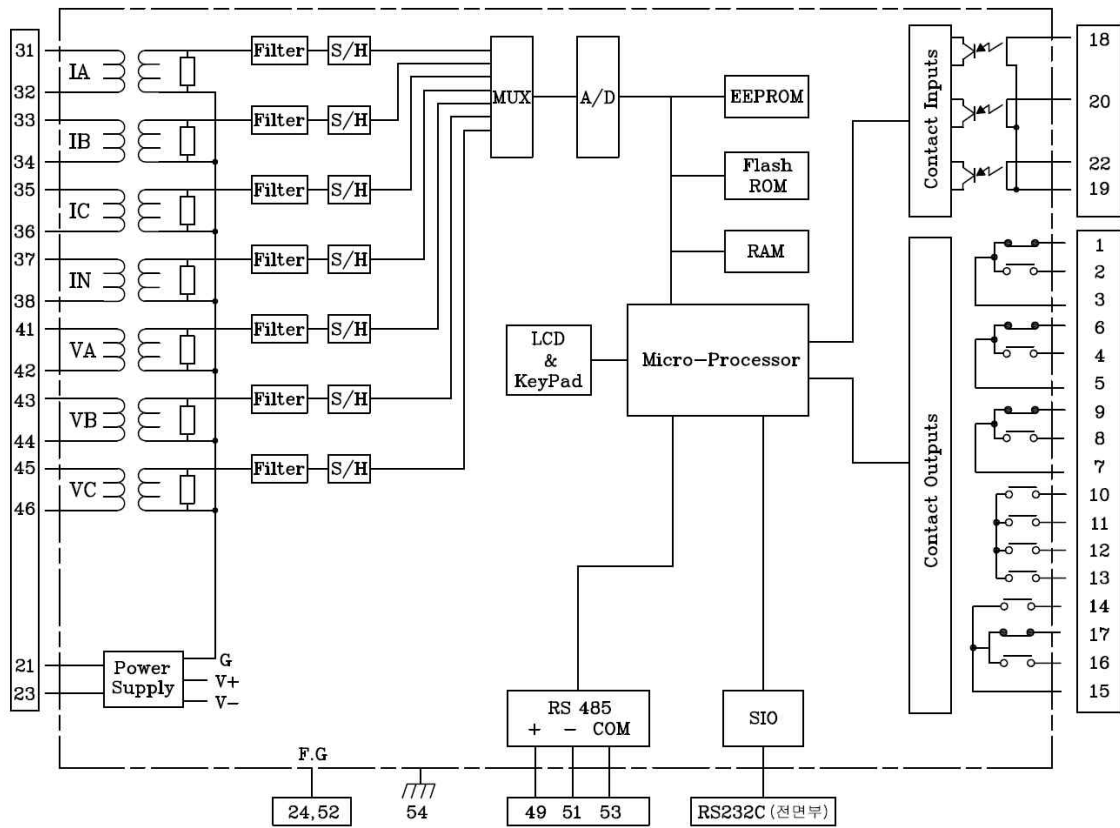
<부도 2. Internal Block Diagram>
