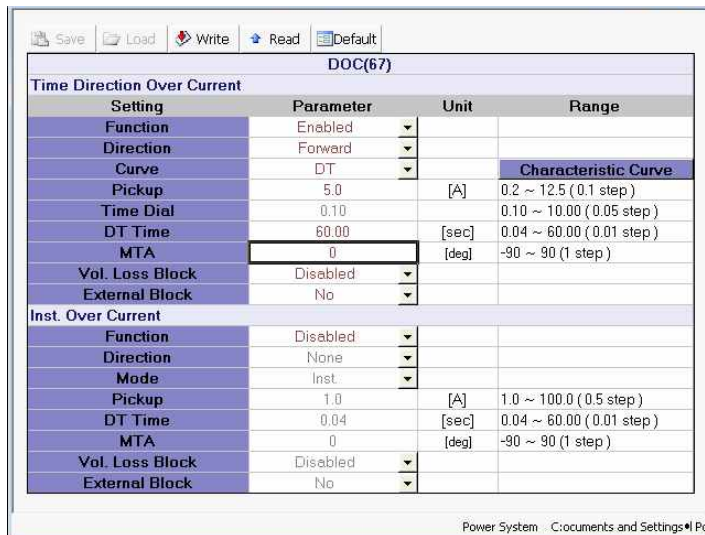
<그림 5. DOCR 정한시(최대) 설정>
