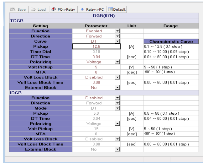
<그림 8. TDGR 동작치 설정>
