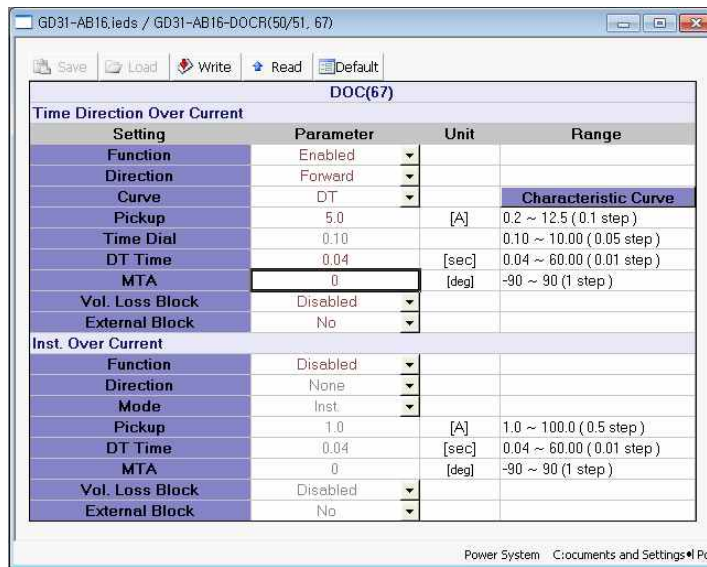
<그림 6. TDOCR 동작위상 설정>
