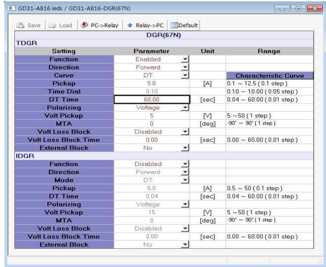
<그림 13. TDGR 동작위상 설정>
