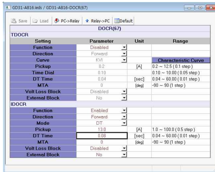
<그림 8. IDOCR 부동작 특성 시험 설정>
