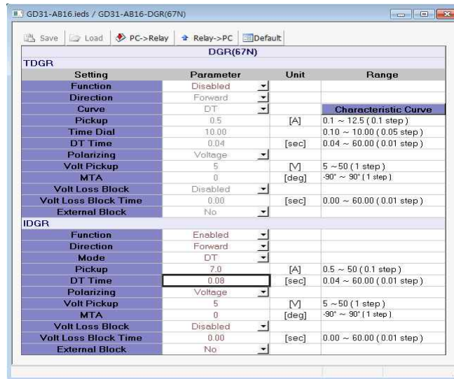
<그림 15. IDGR 부동작 특성 시험 설정>
