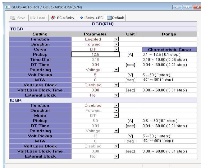
<그림 10. TDGR 동작치 설정>
