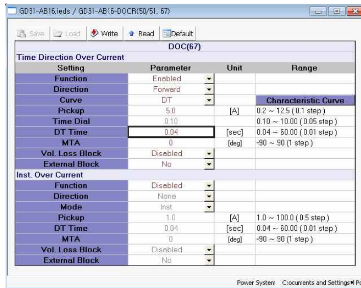
<그림 4. TDOCR 정한시(최소) 설정>
