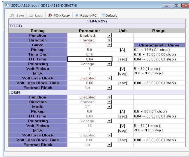
<그림 11. TDGR 동작시간 설정>
