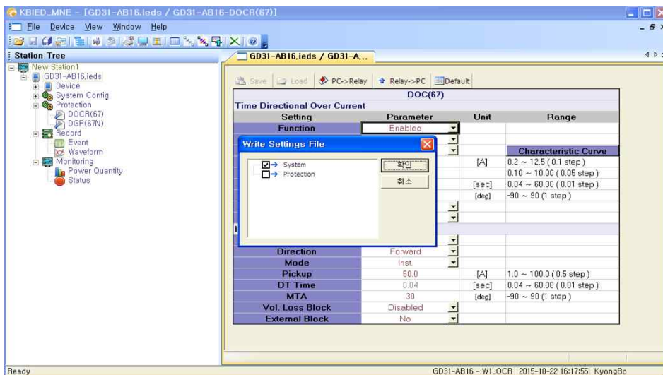
<Figure 22. 저장된 파일을 보호계전기(Device)로 다운로드(PC→Device)>
