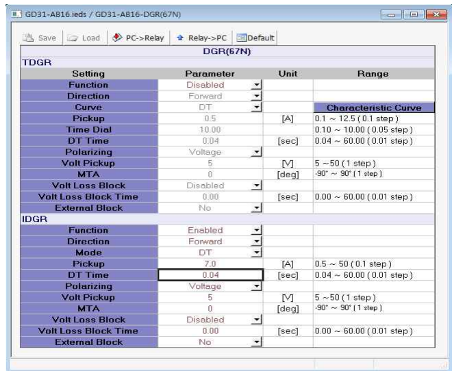
<그림 14. IDGR 부동작 특성 시험 설정>
