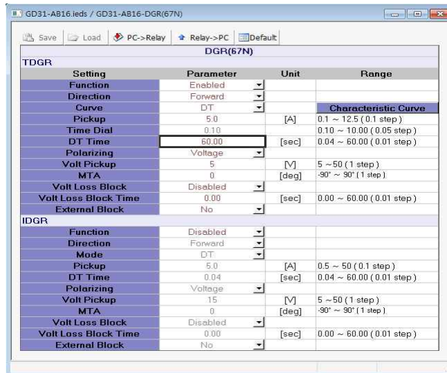
<그림 12. TDGR 동작시간 설정>
