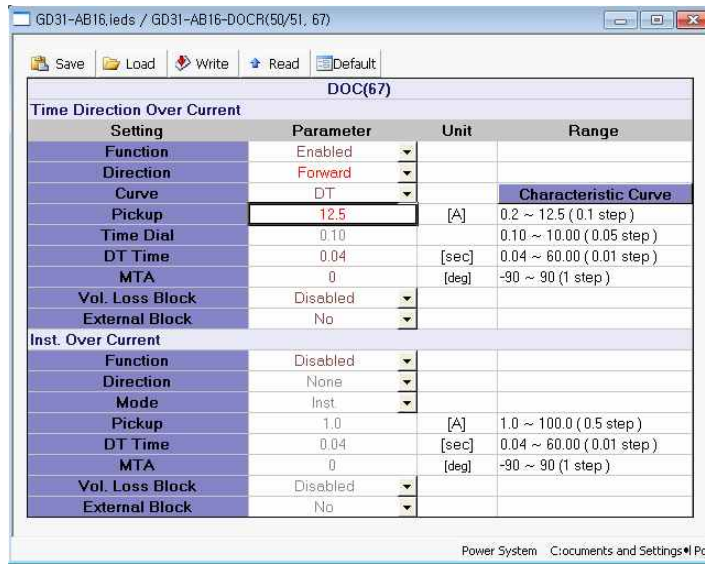
<그림 3. TDOCR 동작치(최대) 설정>
