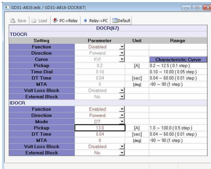
<그림 7. IDOCR 부동작 특성 시험 설정>
