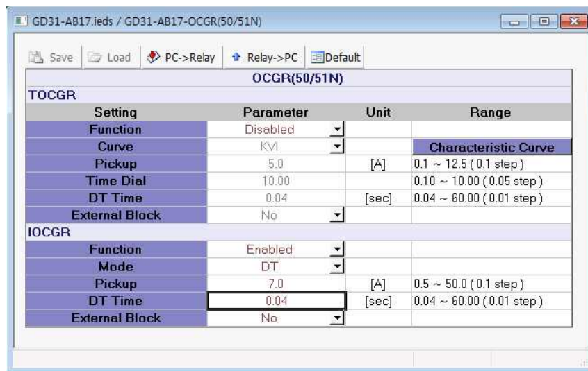
<그림 16. IOCGR 부동작 특성 시험 설정>
