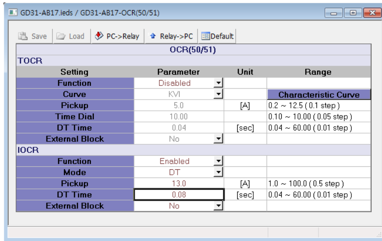
<그림 9. OCR 부동작 특성 시험 설정>
