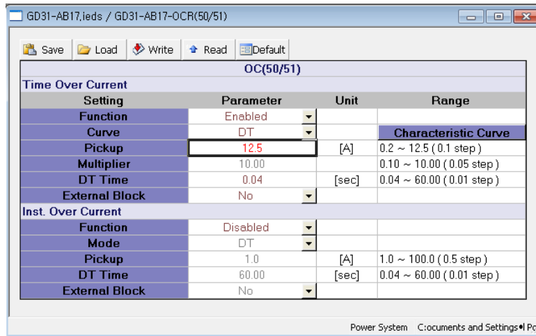
<그림 3. TOCR 동작치(최대) 설정>
