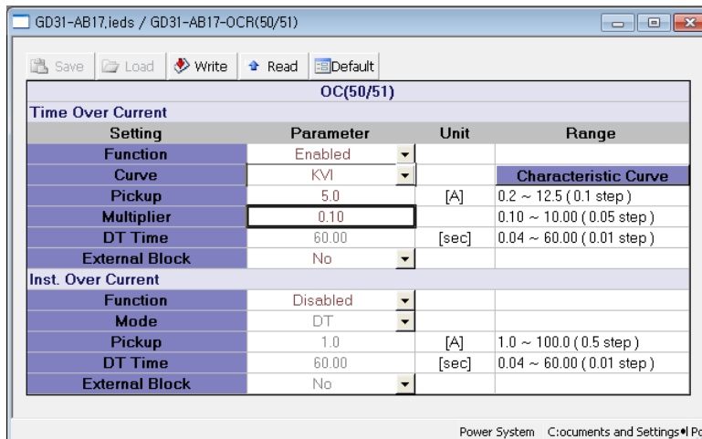
<그림 6. TOCR 반환시(최소) 설정>
