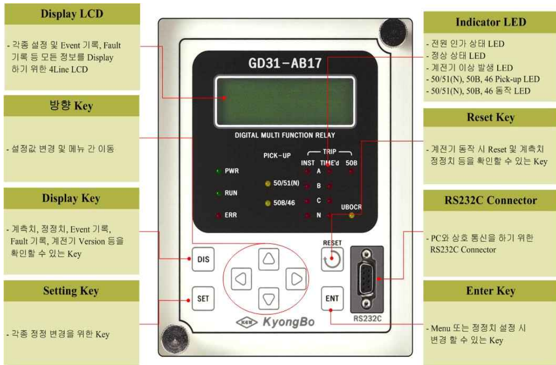
<Figure 10. 전면 표시부>
