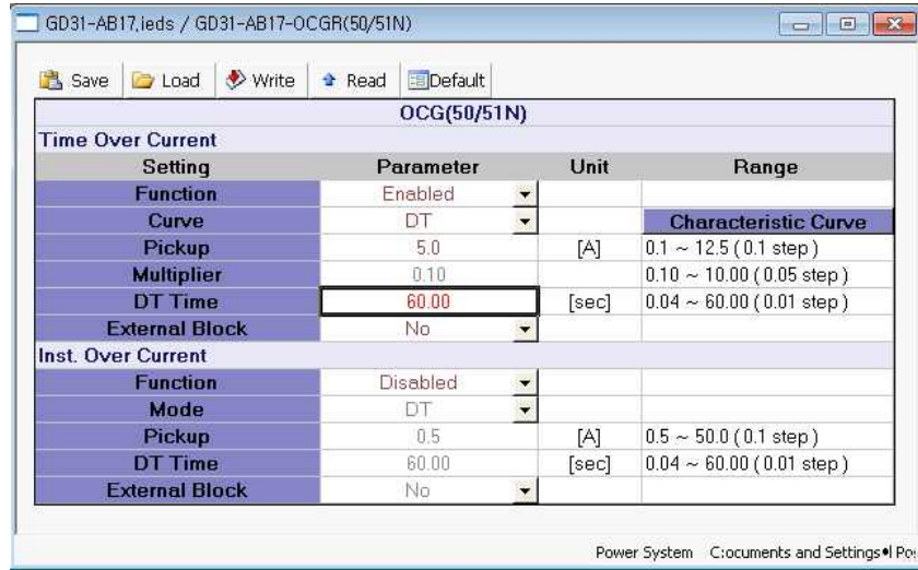
<그림 13. TOCGR 정한시(최대) 설정>
