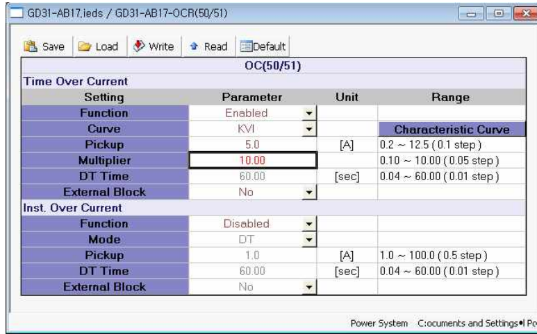
<그림 7. TOCR 반환시(최대) 설정>
