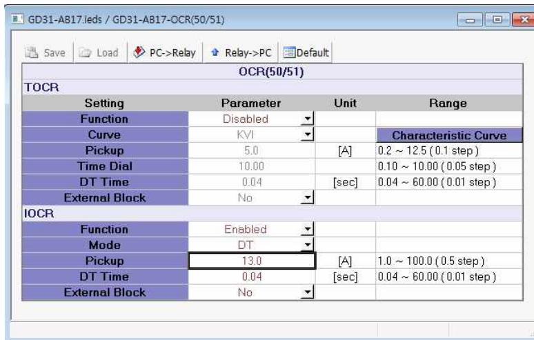
<그림 8. OCR 부동작 특성 시험 설정>
