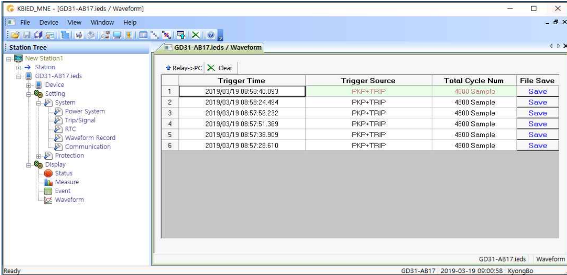
<Figure 27. WaveForm>
