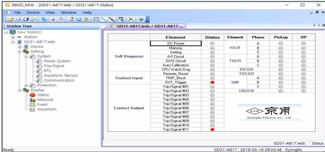
<Figure 29. Status>
