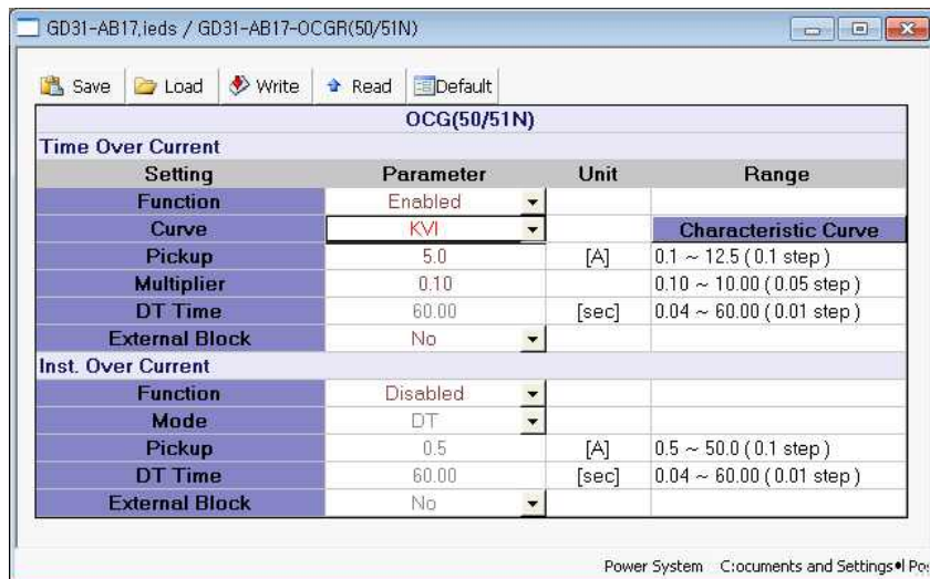
<그림 14. TOCGR 반환시(최소) 설정>
