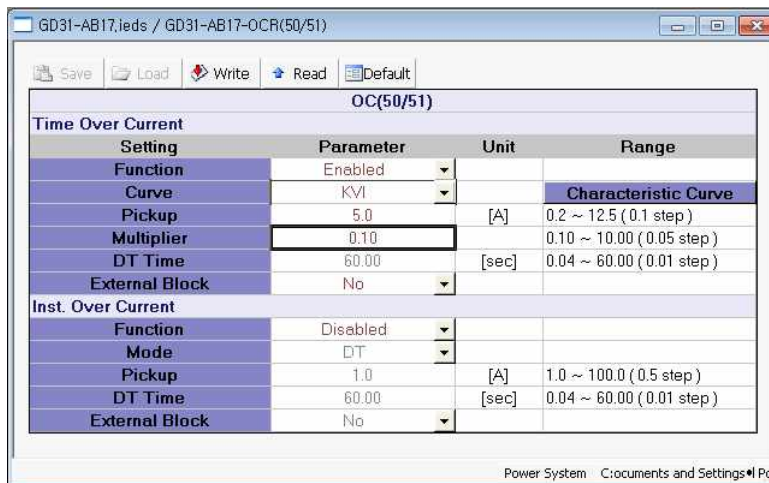
<그림 6. TOCR 반한시(최소) 설정>
