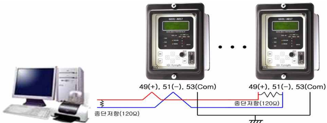
<Figure 9. RS-485 결선도>
