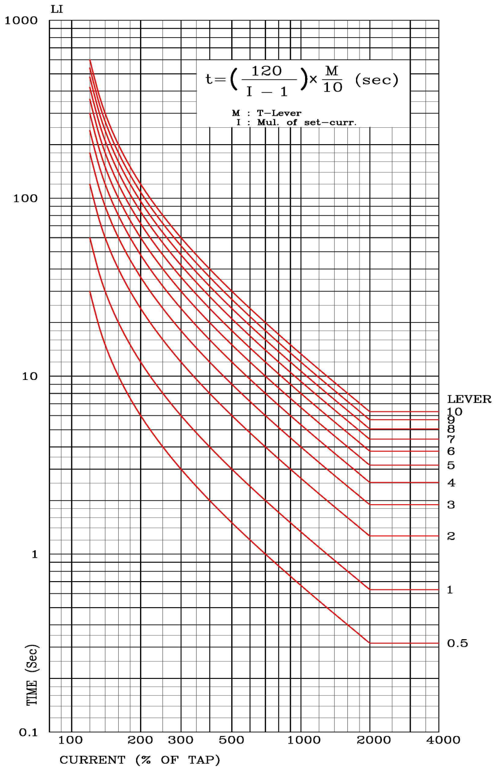
<부도 5.3 장반한시 특성 곡선>
