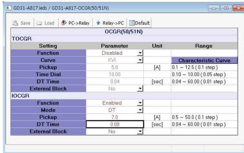
<그림 17. IOCGR 부동작 특성 시험 설정>
