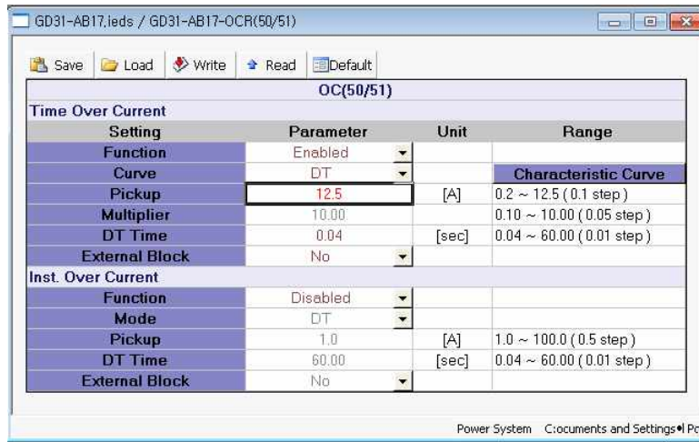
<그림 3. TOCR 동작치(최대) 설정>
