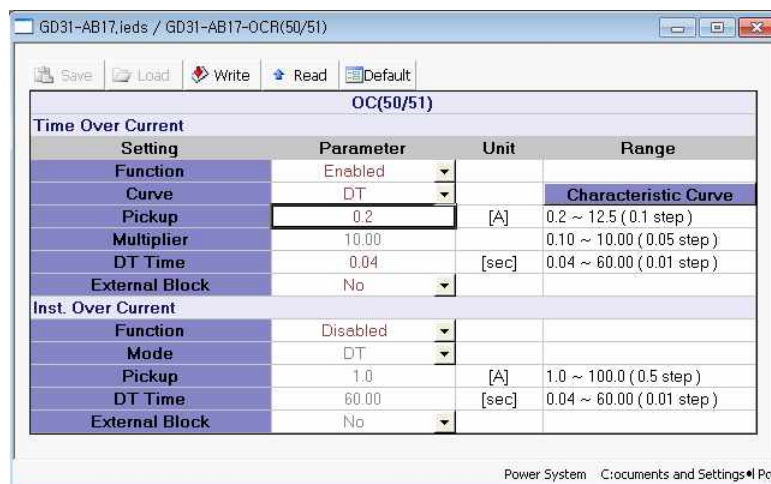
<그림 2. TOCR 동작치(최소) 설정>
