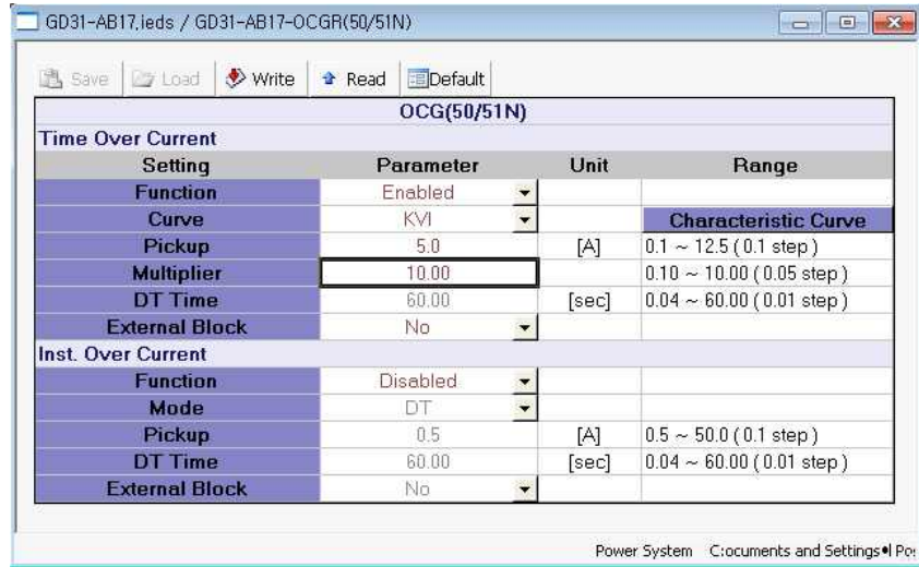
<그림 15. TOCGR 반한시(최대) 설정>
