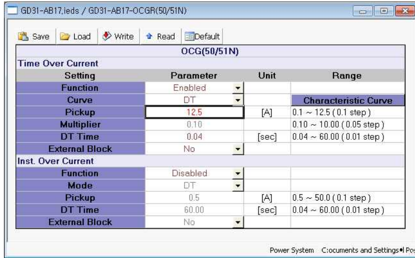
<그림 11. TOCGR 동작치(최대) 설정>
