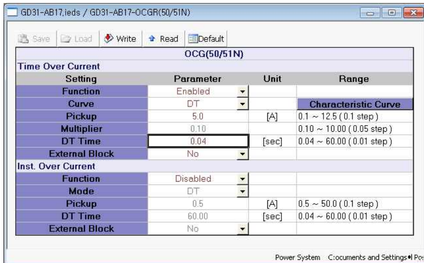
<그림 12. TOCGR 정한시(최소) 설정>
