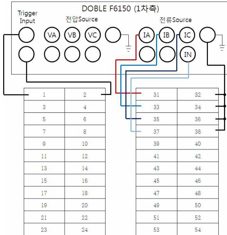
<그림 1. 계전기 Test 장비와 GD31-AB17 결선도>
