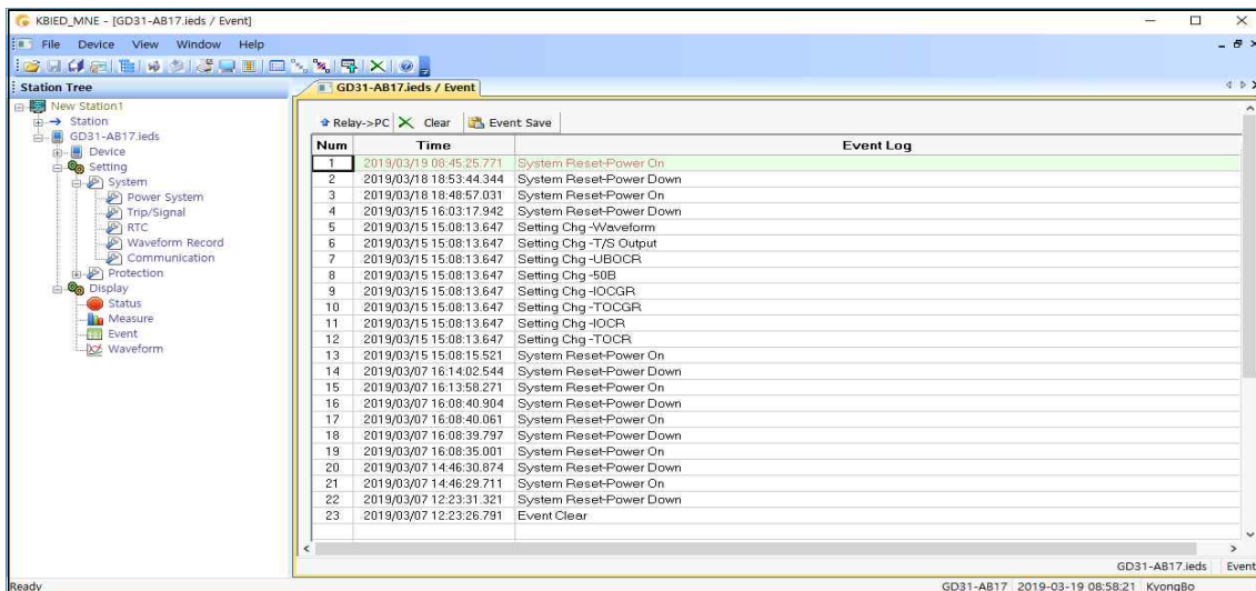
<Figure 26. Event>
