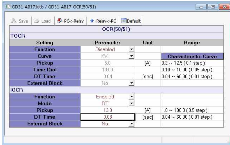
<그림 9. OCR 부동작 특성 시험 설정>
