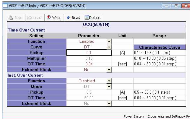
<그림 10. TOCGR 동작치(최소) 설정>
