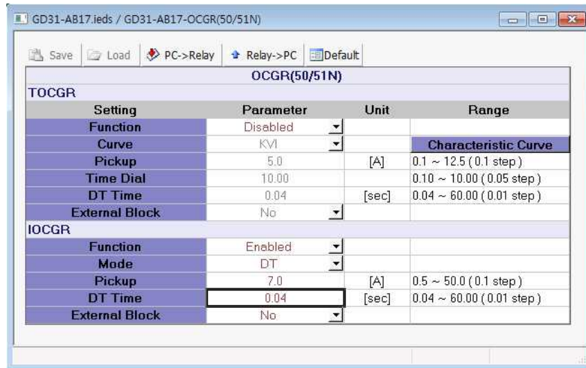
<그림 16. IOCGR 부동작 특성 시험 설정>
