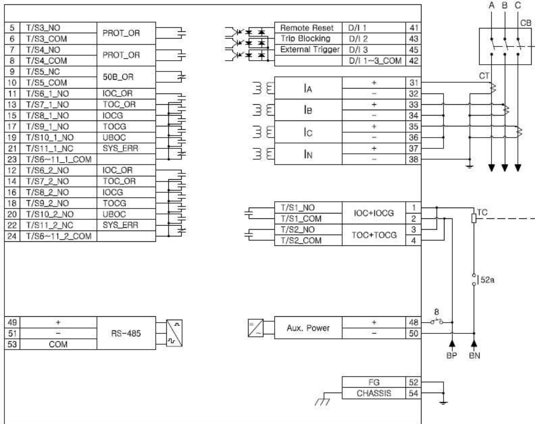
<부도 4. 한전 23kV D/L 보호 외부 결선도>
