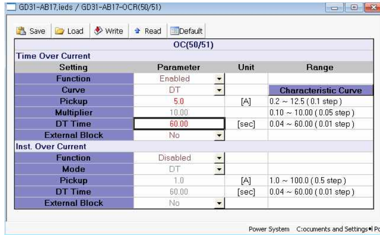
<그림 5. TOCR 정한시(최대) 설정>
