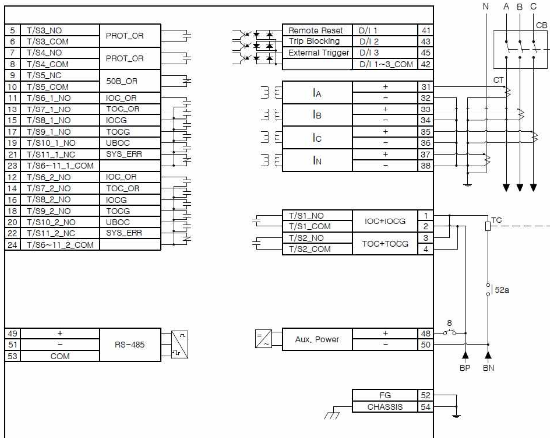
<부도 3. 한전 154kV 변압기 보호 51S 외부 결선도>
