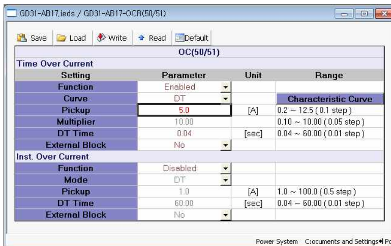
<그림 4. TOCR 정한시(최소) 설정>
