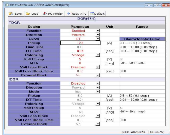
<그림 10. TDGR 동작치 설정>
