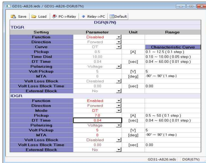
<그림 14. IDGR 부동작 특성 시험 설정>
