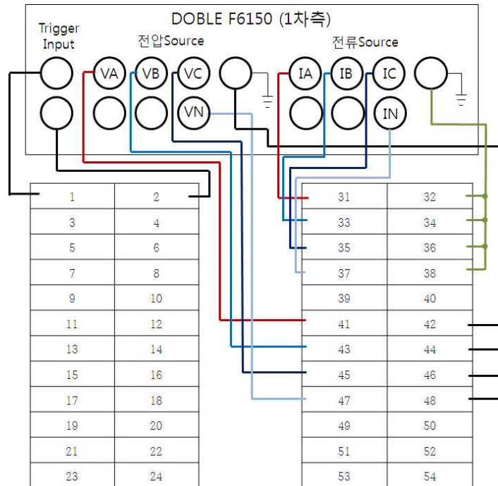
<그림 1. 계전기 Test 장비와 GD31-AB26 결선도>
