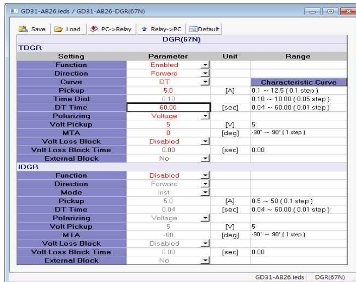
<그림 12. TDGR 동작시간 설정>
