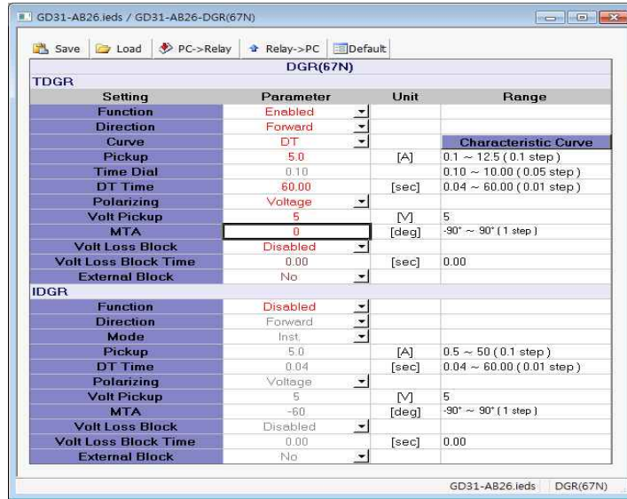
<그림 13. TDGR 동작위상 설정>
