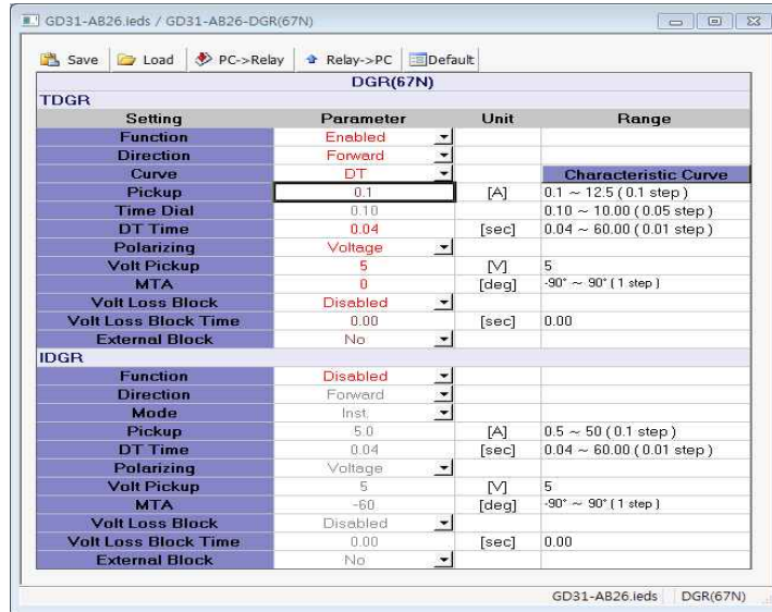
<그림 9. TDGR 동작치 설정>
