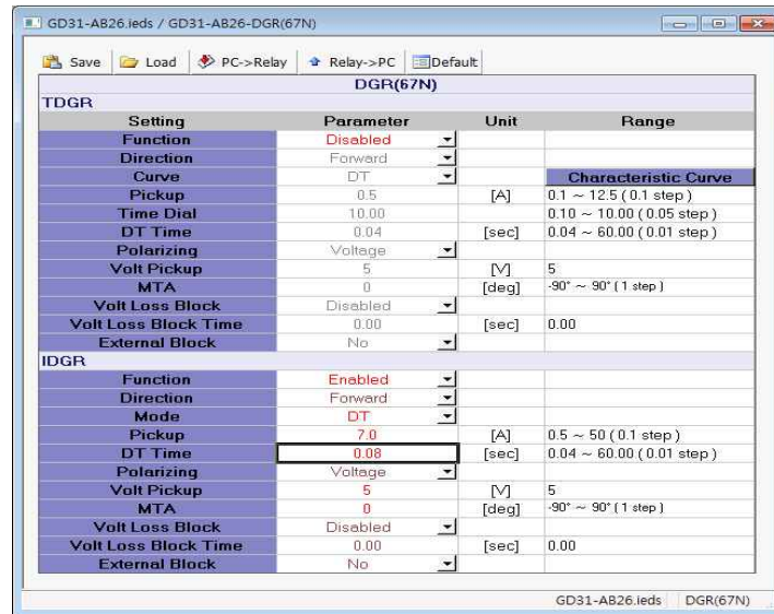
<그림 15. IDGR 부동작 특성 시험 설정>
