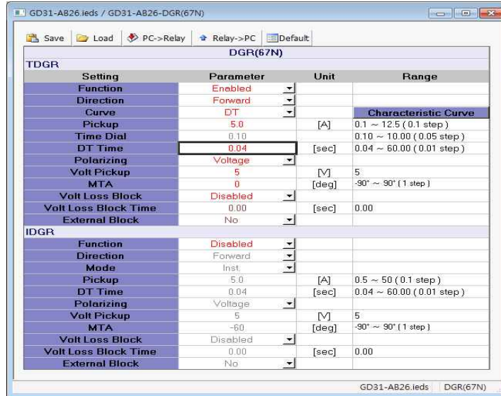
<그림 11. TDGR 동작시간 설정>
