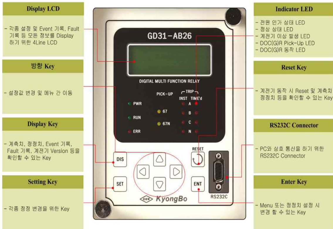
<Figure 11. 전면 표시부>
