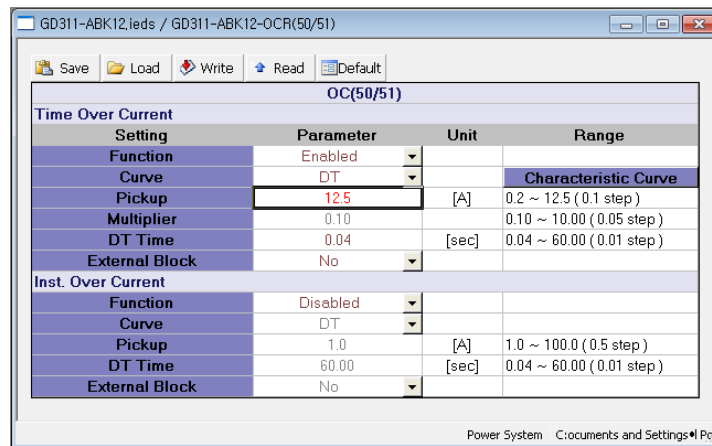
<그림 3. TOCR 동작치(최대) 설정>
