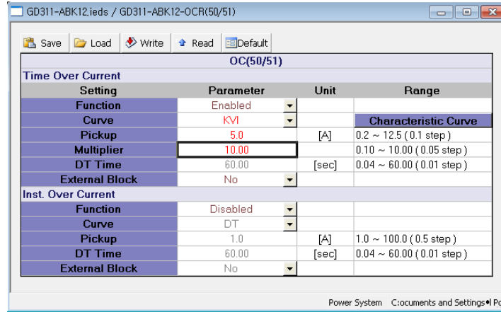
<그림 7. TOCR 반한시(최대) 설정>
