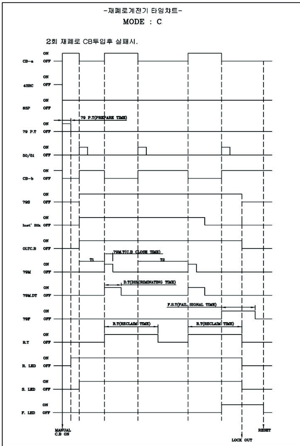
<부도 4.13 C Mode 2회 재폐로 실패 시>
