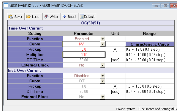
<그림 6. TOCR 반한시(최소) 설정>
