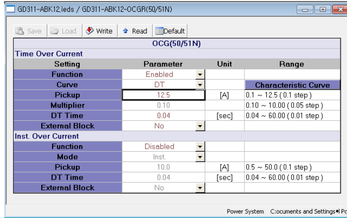
<그림 9. TOCGR 동작치(최대) 설정>
