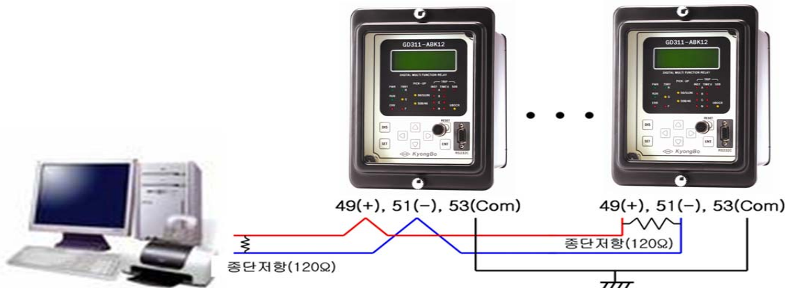
<Figure 10. RS-485 결선도>
