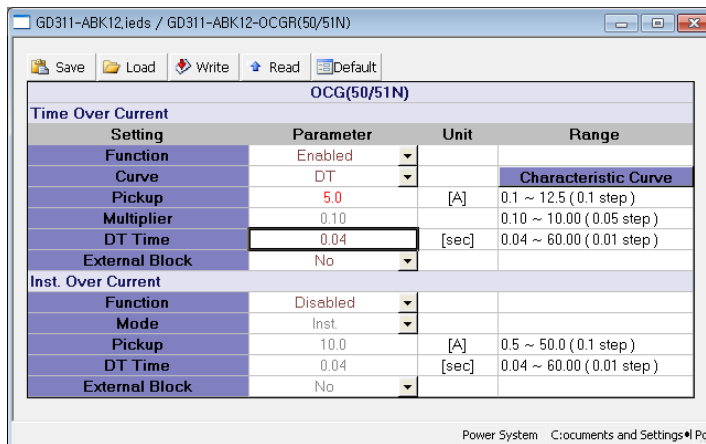
<그림 10. TOCGR 정한시(최소) 설정>
