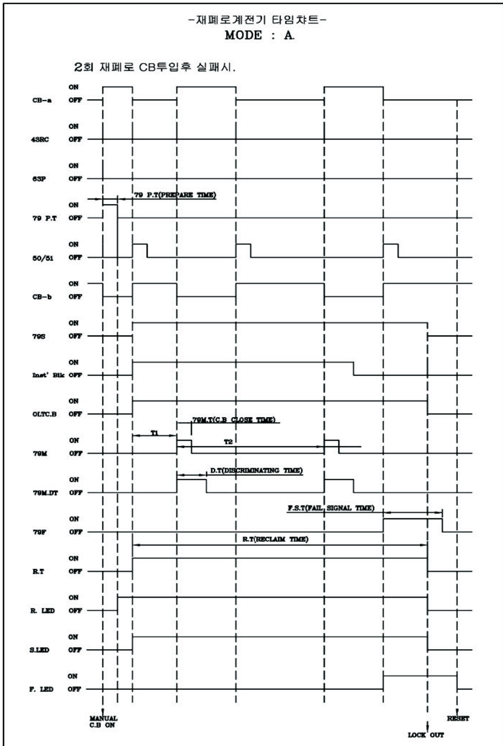
<부도 4.10 A Mode 2회 재폐로 실패 시>
