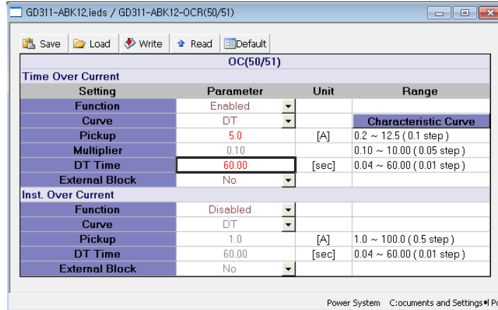
<그림 5. TOCR 정한시(최대) 설정>
