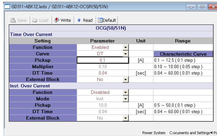
<그림 8. TOCGR 동작치(최소) 설정>
