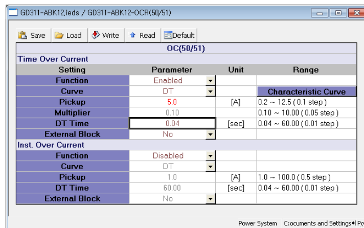
<그림 4. TOCR 정한시(최소) 설정>
