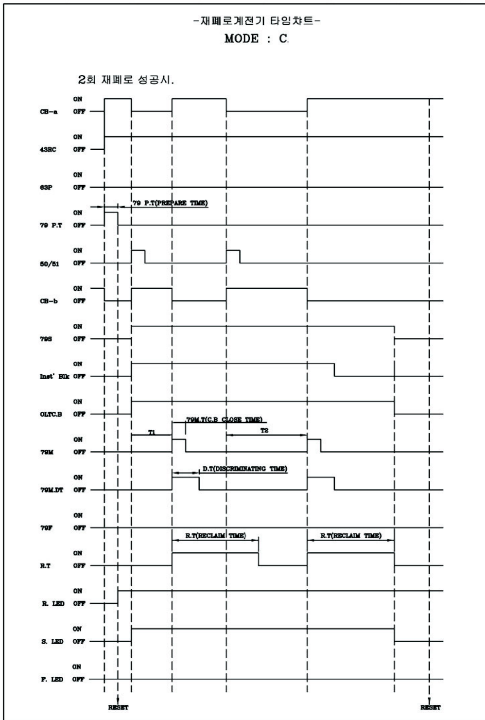
<부도 4.12 C Mode 2회 재폐로 성공 시>
