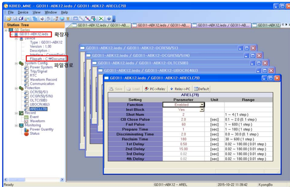
<Figure 18. Project 저장 화면>
