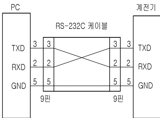
<Figure 8. RS-232C 회로도>
