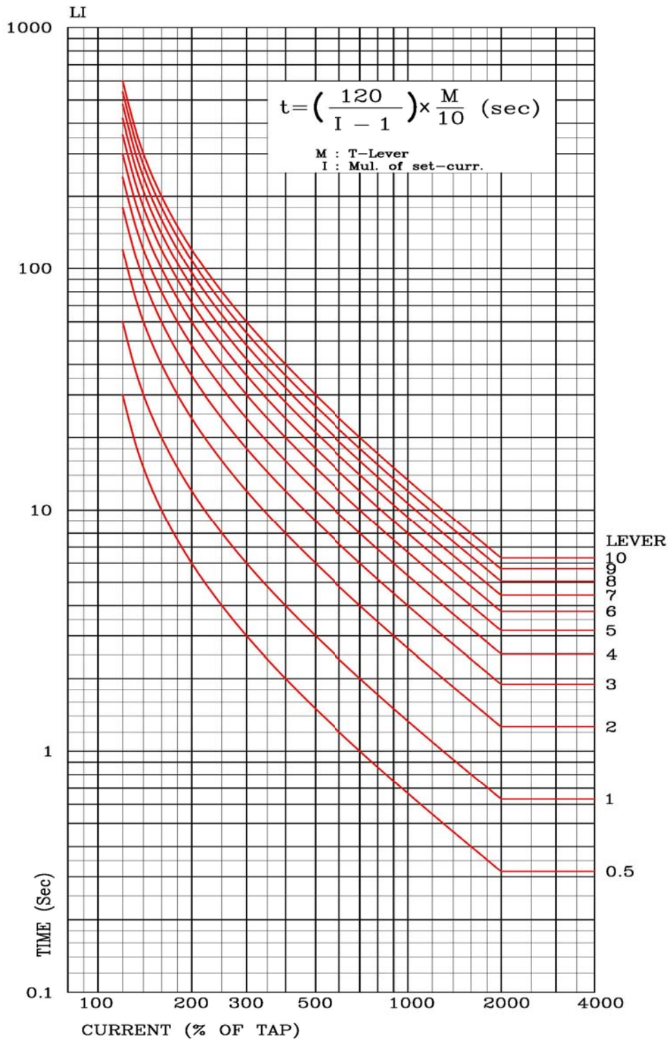
<부도 4.3 장만한시 특성 곡선>
