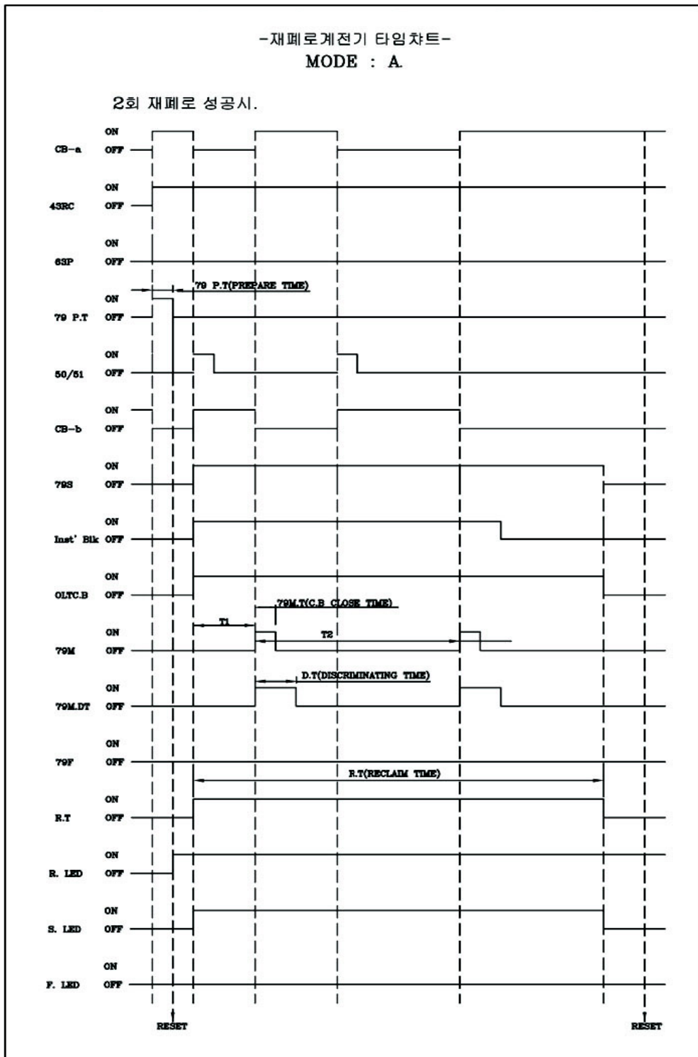
<부도 4.9 A Mode 2회 재폐로 성공 시>
