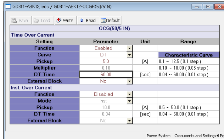
<그림 11. TOCGR 정한시(최대) 설정>
