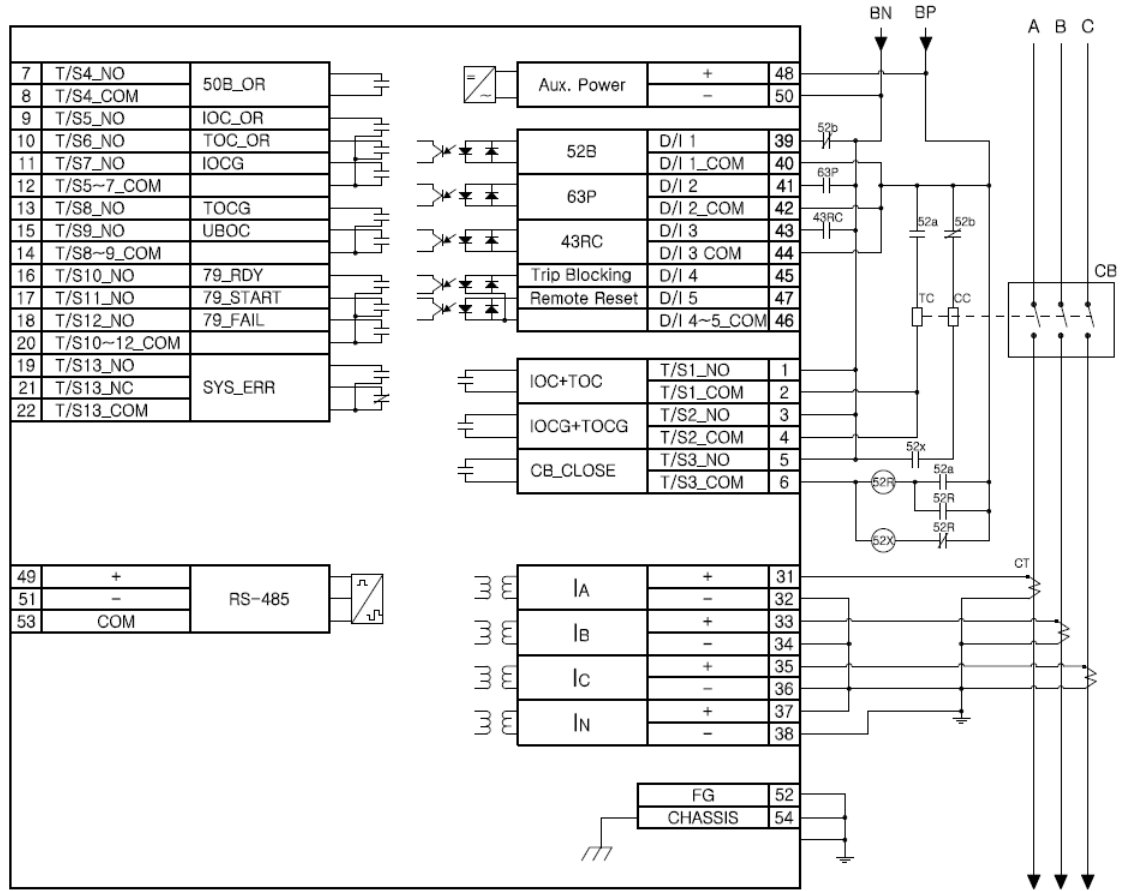
<부도 3. 외부 결선도>
