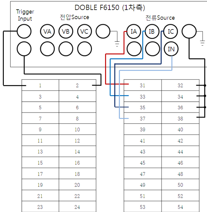
<그림 1. 계전기 Test 장비와 GD311-ABK12 결선도>
