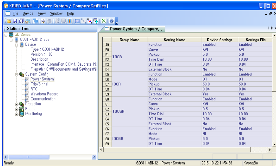
<Figure 25. 정정치 비교 화면>
