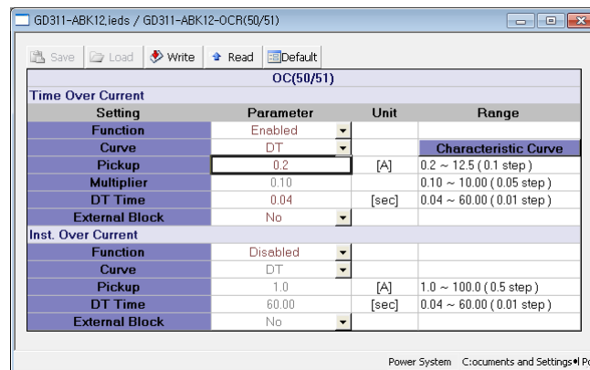
<그림 2. TOCR 동작치(최소) 설정>
