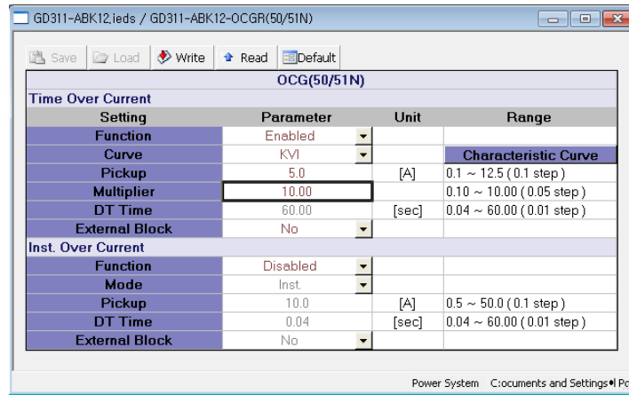
<그림 13. TOCGR 반한시(최대) 설정>
