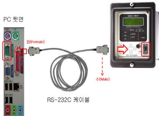
<Figure 9. RS-232C 연결>
