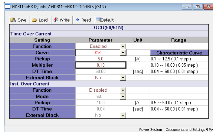
<그림 12. TOCGR 반환시(최소) 설정>
