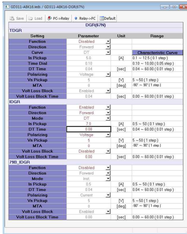
<Figure 부록 D-15. IDGR 부동작 특성 시험 설정>
