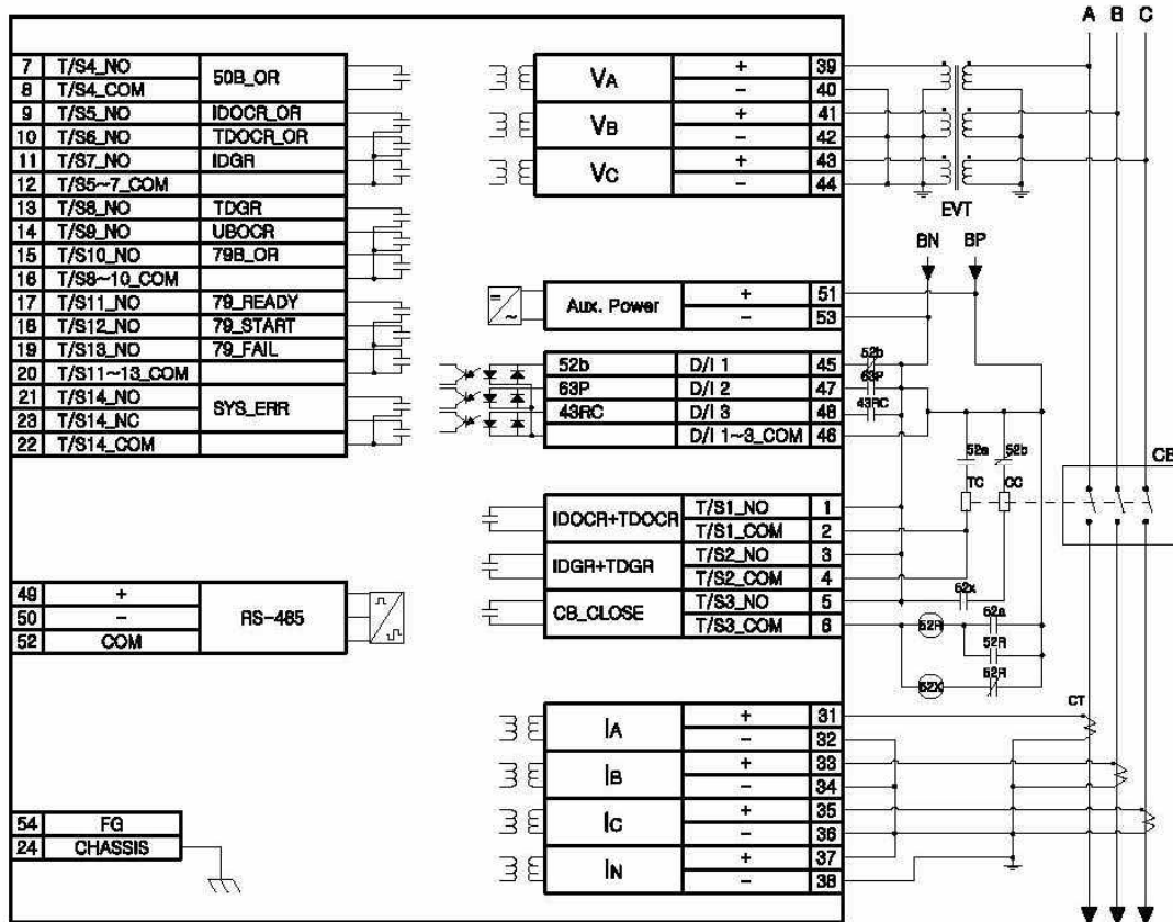
<부도 3. 외부 결선도>
