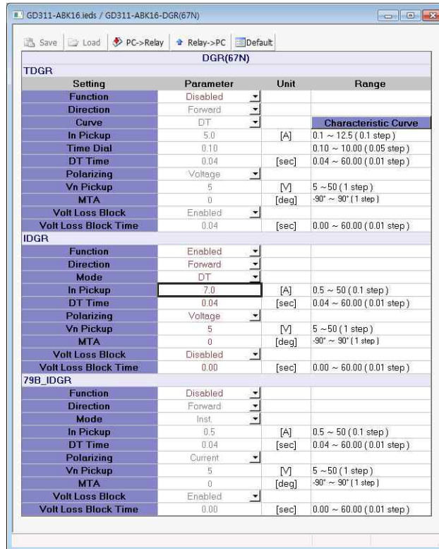
<Figure 부록 D-14. IDGR 부동작 특성 시험 설정>
