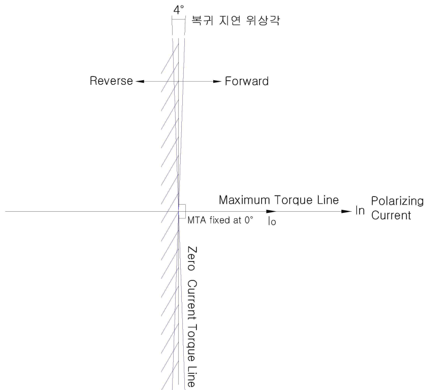
<Figure 6.2 기준 Polarizing을 Current 로 하였을 때의 동작 특성>
