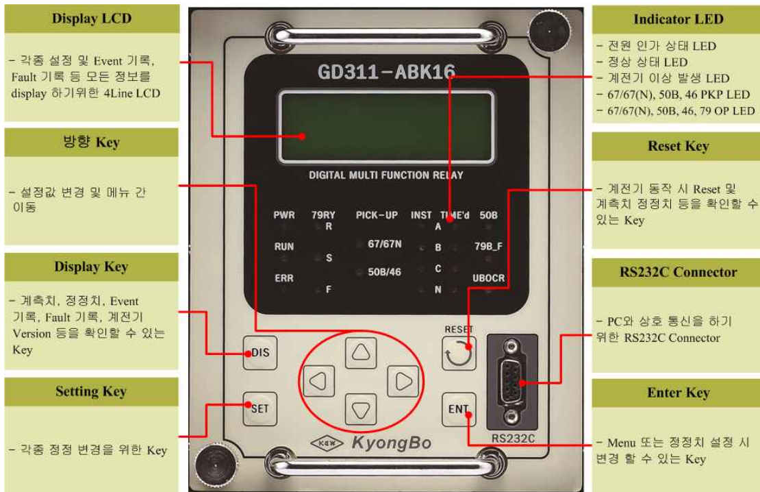
<Figure 16. 전면 표시부>
