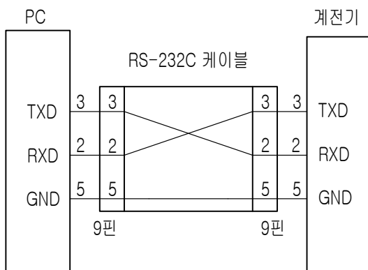
<Figure 13. RS-232C 회로도>
