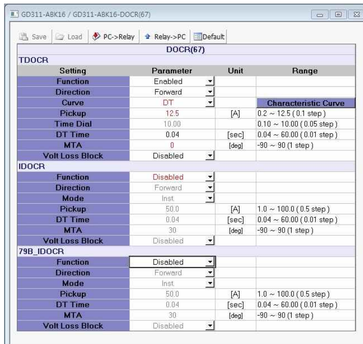
<Figure 부록 D-3. DOCR 동작치(최대) 설정>
