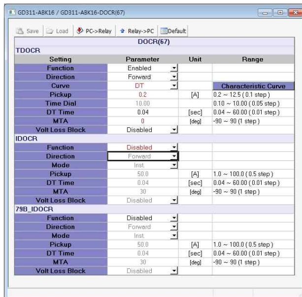
<Figure 부록 D-2. TDOCR 동작치(최소) 설정>
