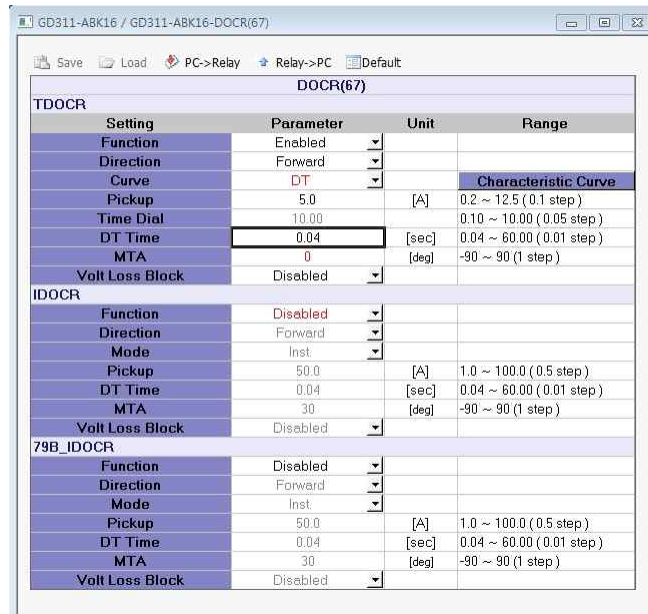
<Figure 부록 D-4. DOCR 정한시(최소) 설정>
