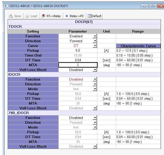
<Figure 부록 D-6. DOCR 동작위상 설정>
