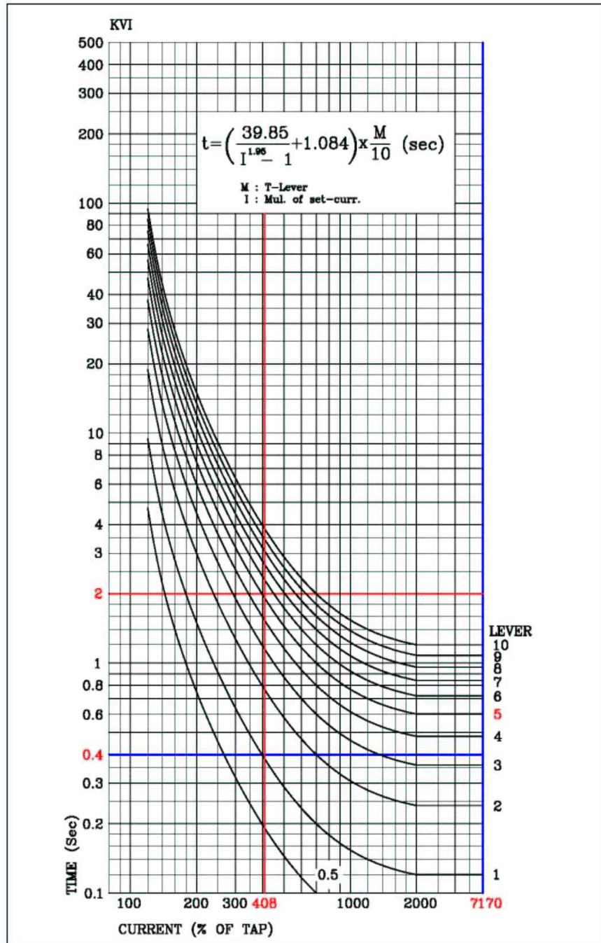
<Figure 부록 B-2 한시 지락 과전류 동작시간 설정>
