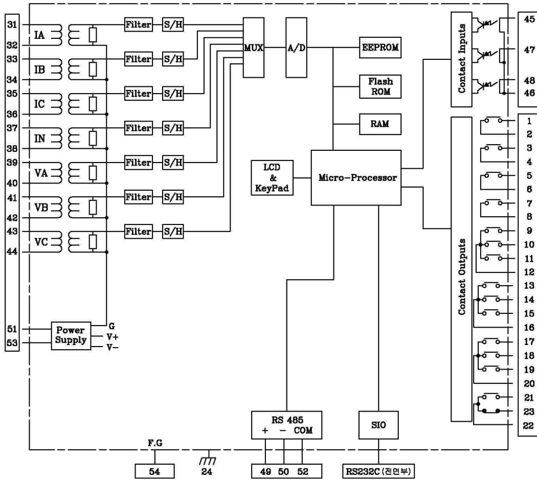
<부도 2. Internal Block Diagram>
