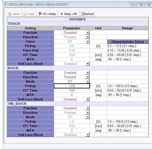
<Figure 부록 D-7. IDOCR 부동작 특성 시험 설정>
