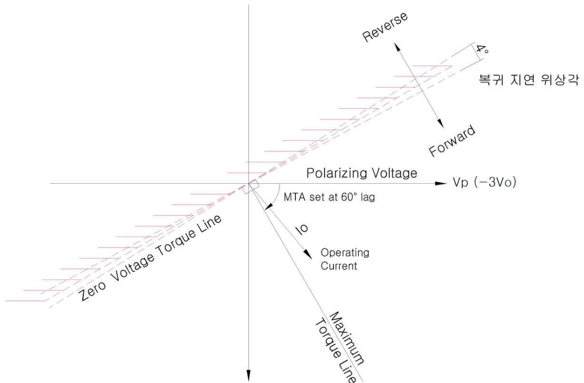
<Figure 6.1 기준 Polarizing을 Voltage 로 하였을 때의 동작 특성>
