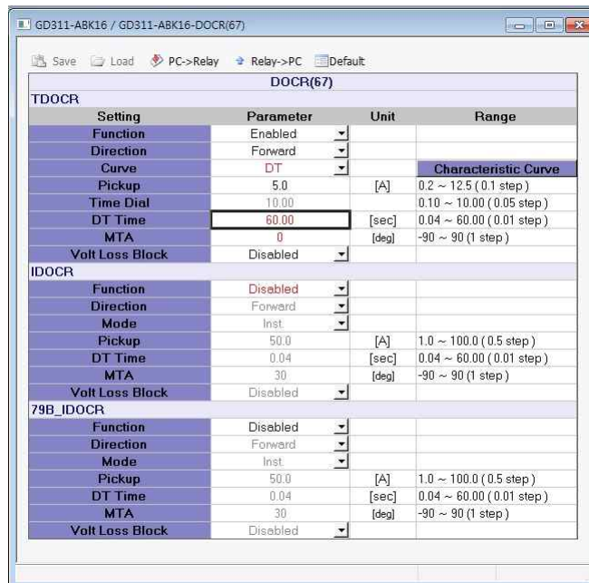
<Figure 부록 D-5. DOCR 정한시(최대) 설정>
