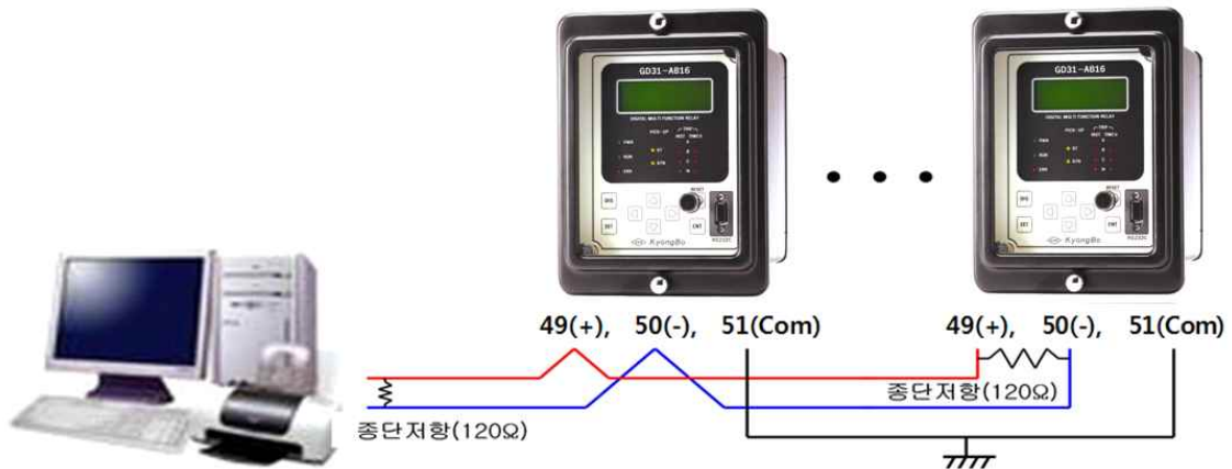
<Figure 15. RS-485 결선도>
