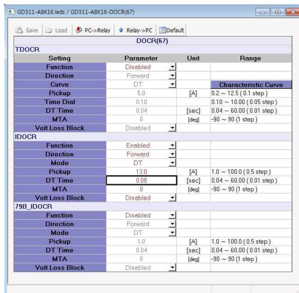
<Figure 부록 D-8. IDOCR 부동작 특성 시험 설정>
