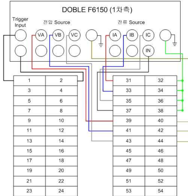
<Figure 부록 D-1. 계전기 Test 장비와 결선도>
