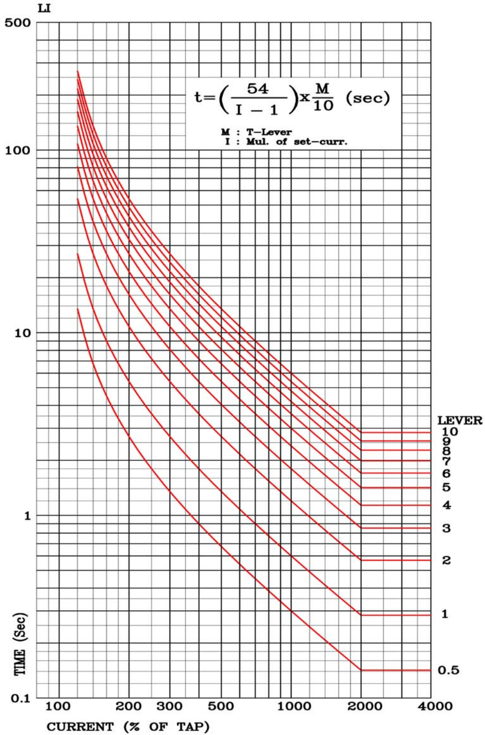
<부도 5.3 OCR 장반한시 특성 곡선>
