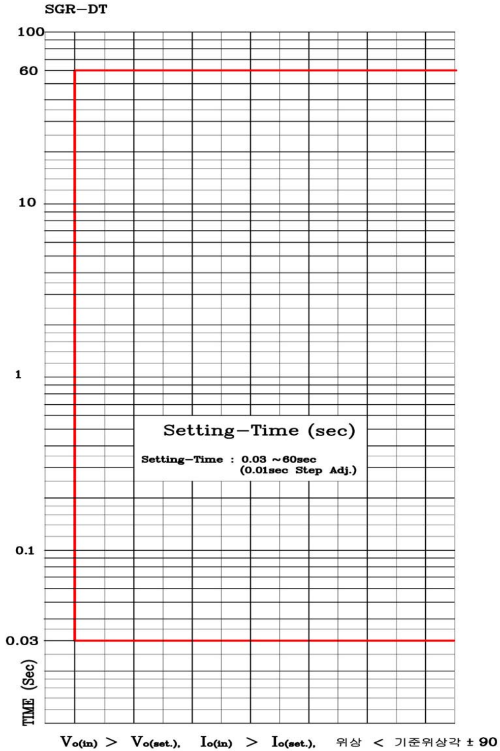
<부도 5.12 SGR 정한시 특성 곡선>
