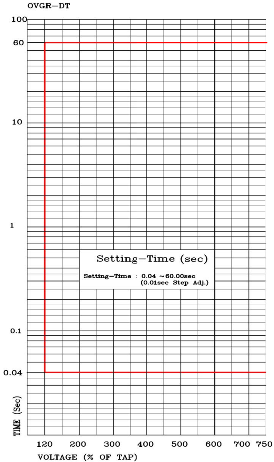
<부도 5.11 OVGR 정한시 특성 곡선>
