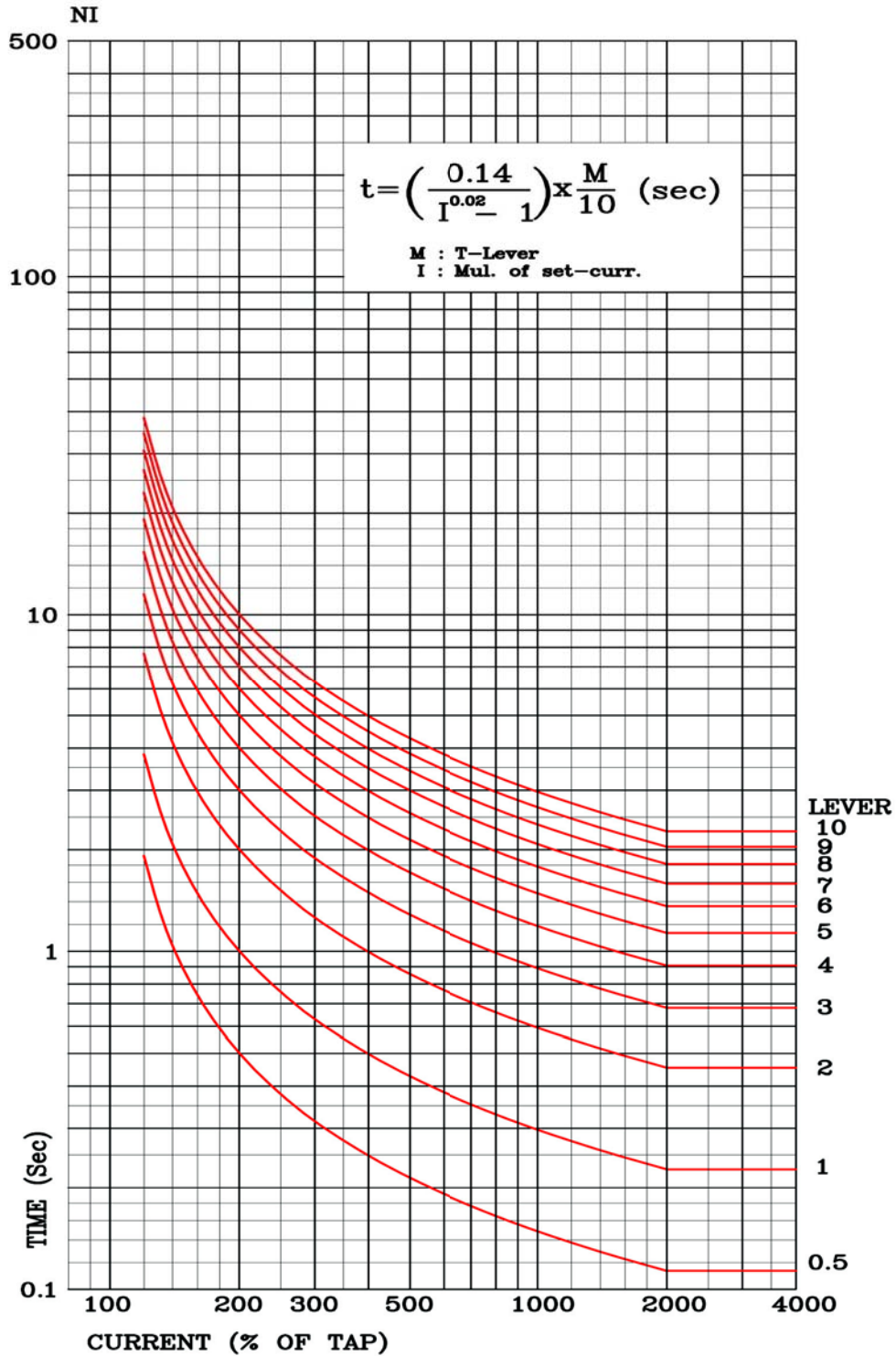
<부도 5.1 OCR 반한시 특성 곡선>
