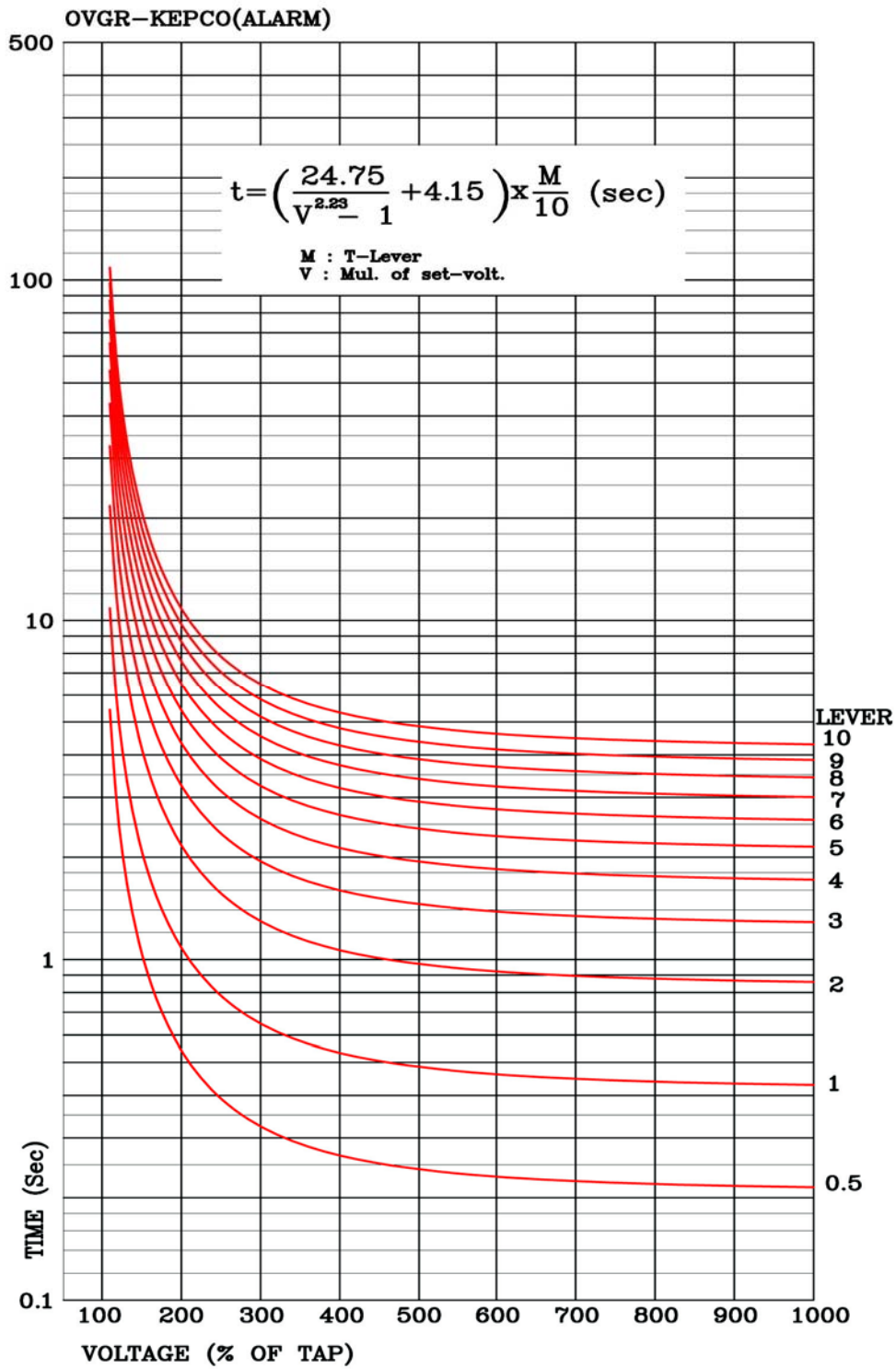
<부도 5.10 OVGR Alarm용 반한시 특성 곡선>
