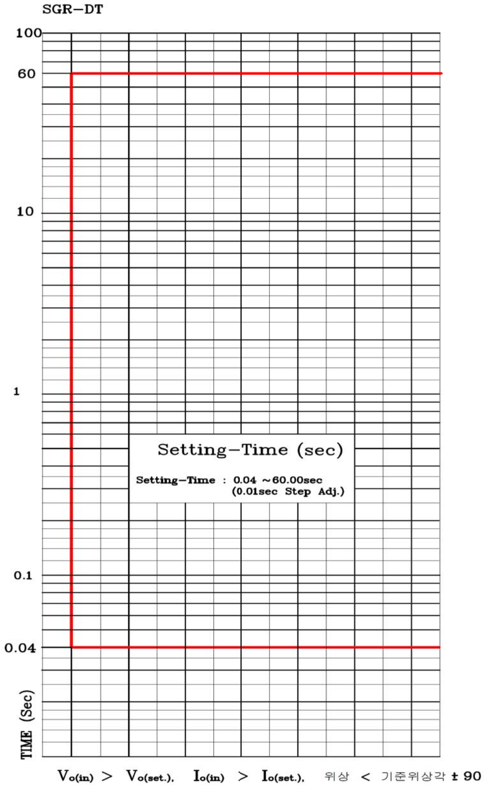
<부도 5.12 SGR 정한시 특성 곡선>
