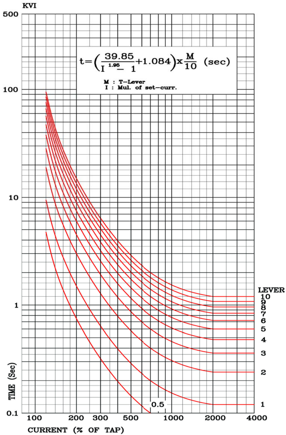
<부도 5.6 OCR 경보유도형 (KEPCO형) 강반한시 특성 곡선>
