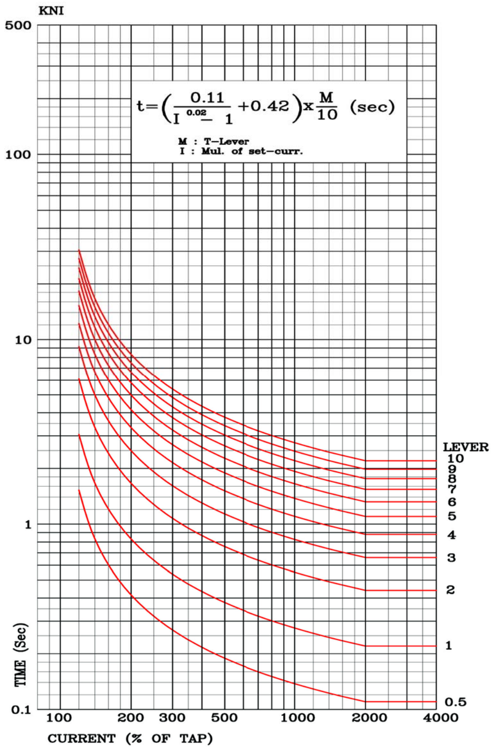
<부도 5.5 OCR 경보유도형 (KEPCO형) 반한시 특성 곡선>
