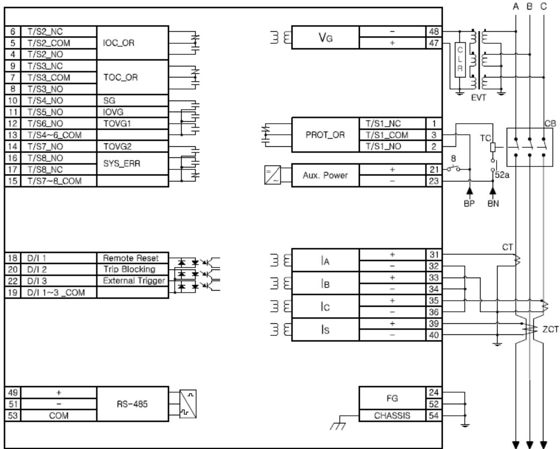
<부도 4. External Connection Diagram>
