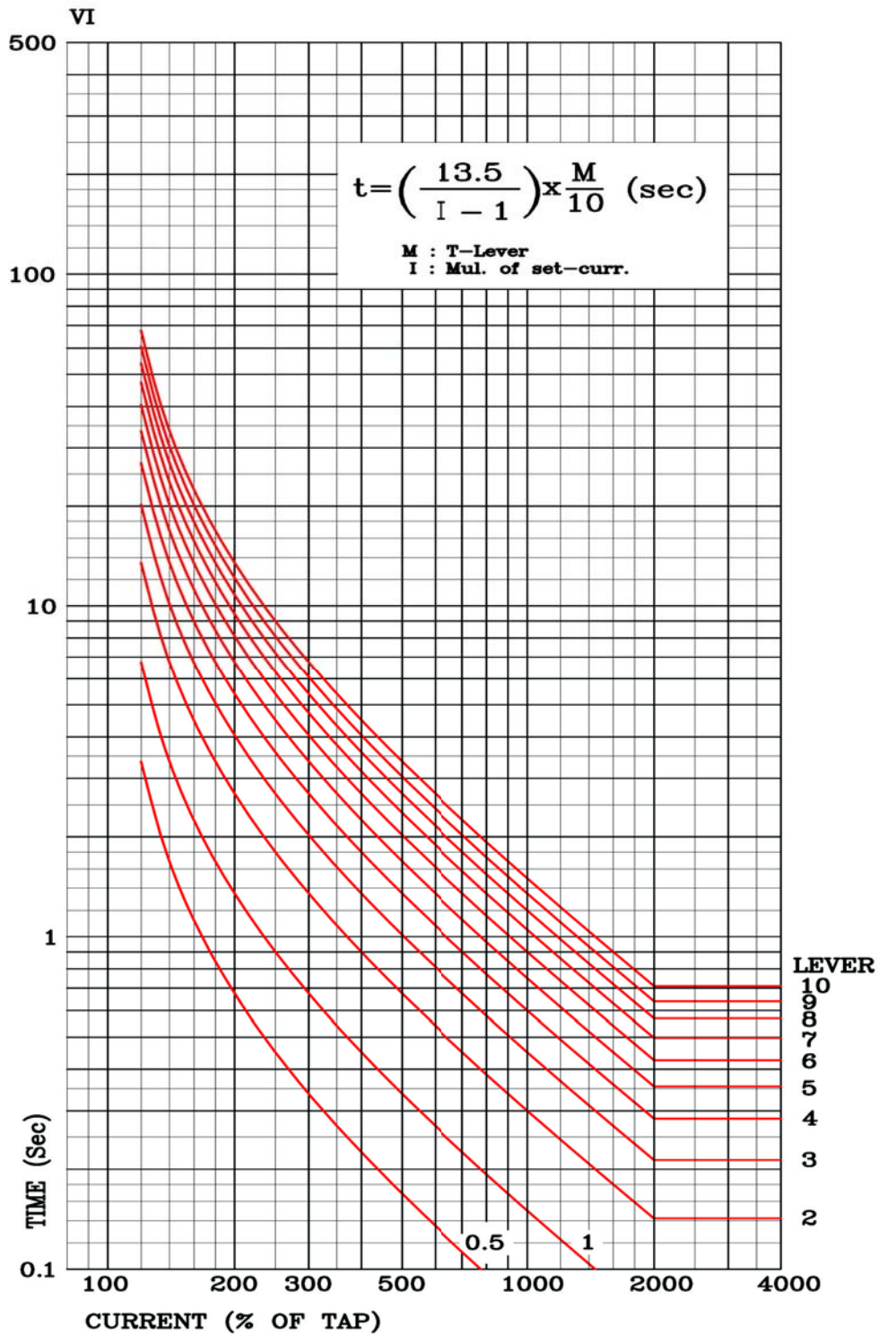
<부도 5.2 OCR 강반한시 특성 곡선>
