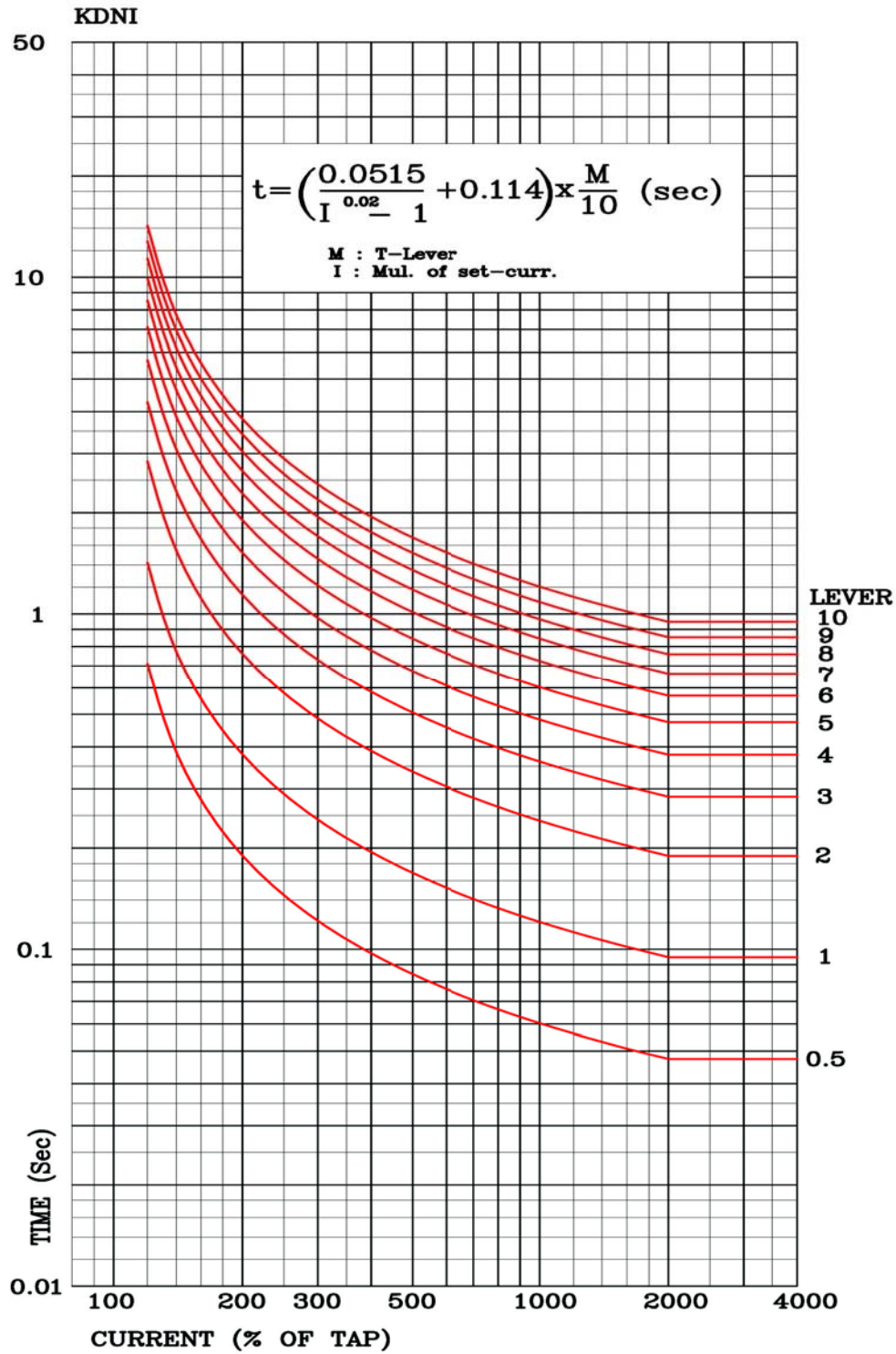
<부도 5.7 OCR 경보유도형 (KEPCO형) 방향성 반한시 특성 곡선>
