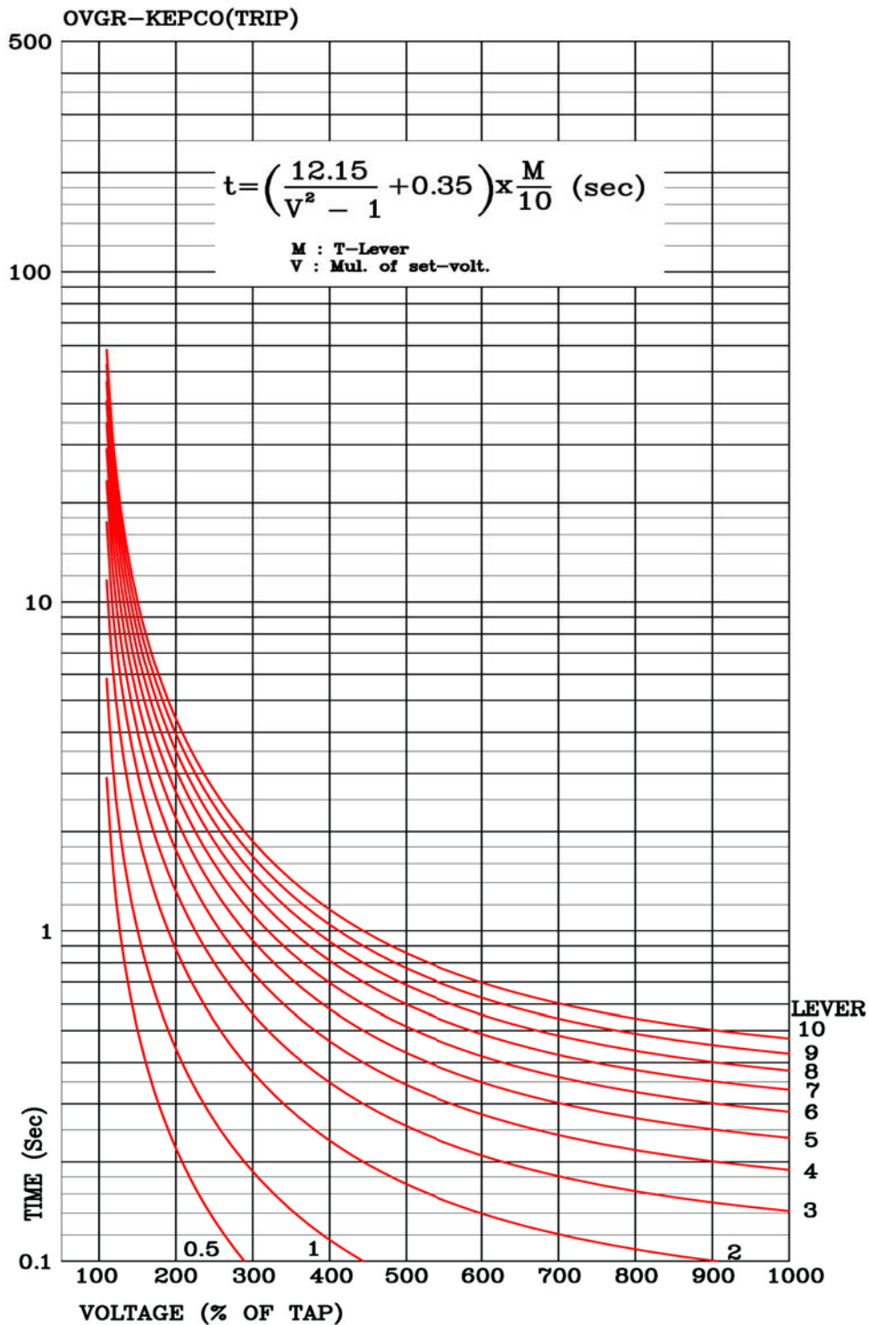
<부도 5.9 OVGR Trip용 반한시 특성 곡선>
