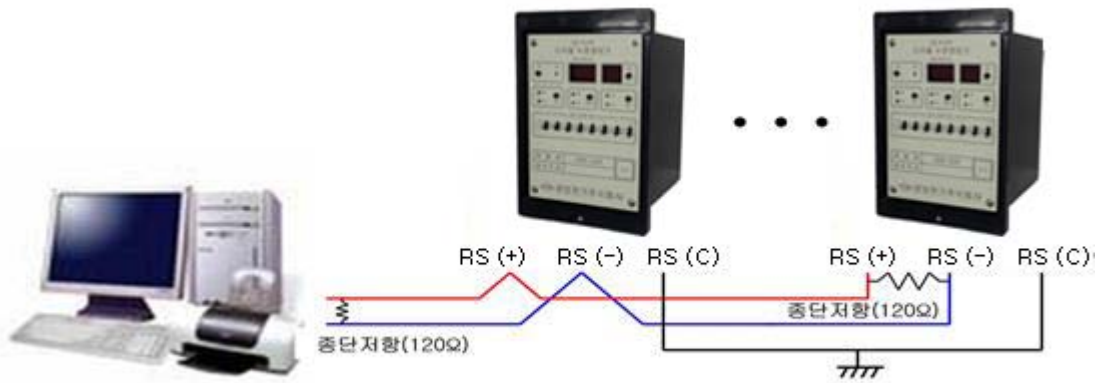
【Figure 1. RS-485 결선도】
