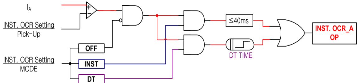
【그림 3.1】 INST. OCR(IOCR) Logic Diagram
