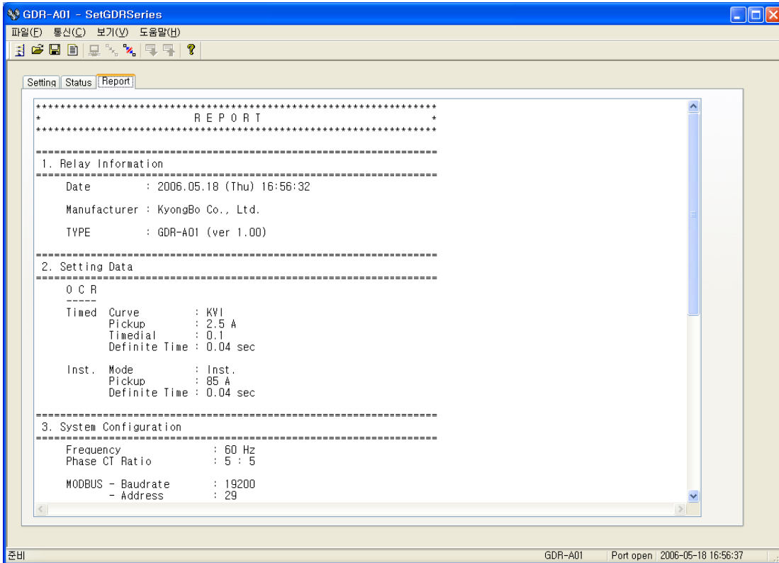
【그림 7.6】 GDR-A01 Report
