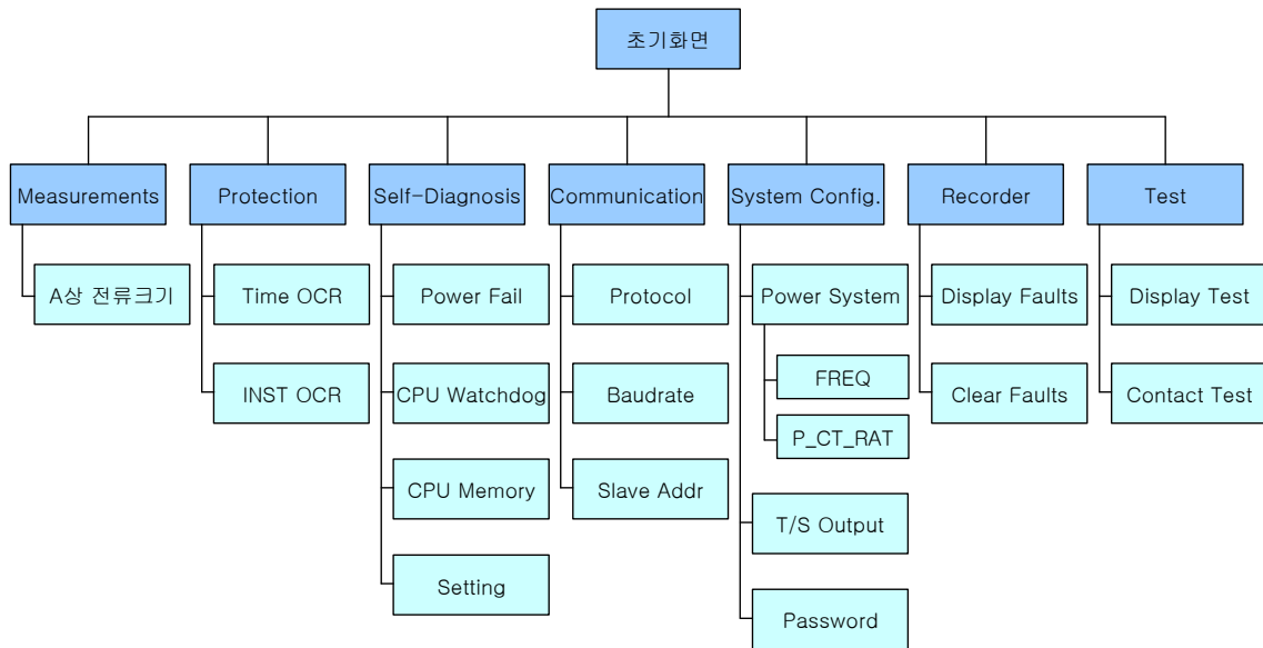
【그림 6.1】 Menu Tree
