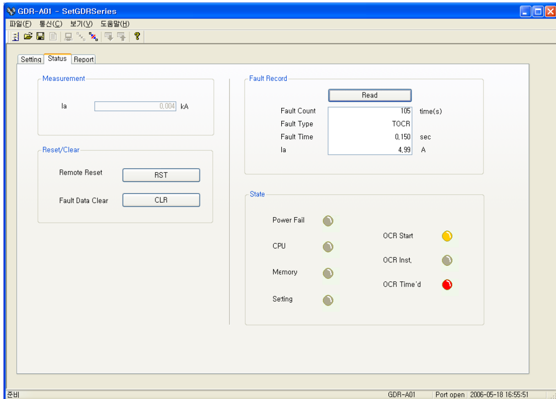
【그림 7.5】 GDR-A01 Status
