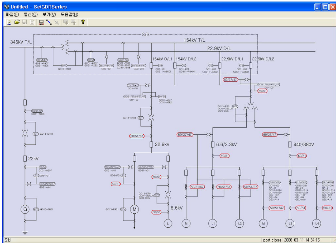
【그림 7.1】 SetGDRSeries 초기화면
