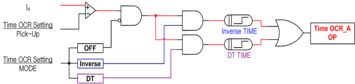
【그림 3.2】 Time OCR(TOCR) Logic Diagram
