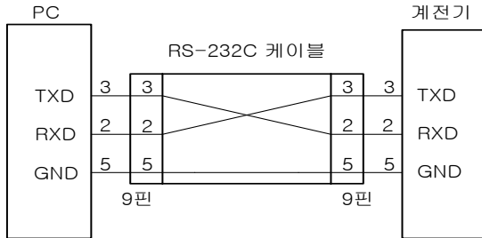
【그림 4.1】 RS-232C 회로도
