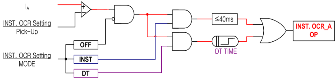
【그림 3.1】 INST. OCR(IOCR) Logic Diagram
