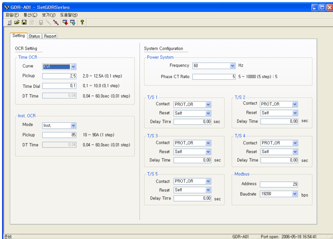
【그림 7.4】 GDR-A01 Setting
