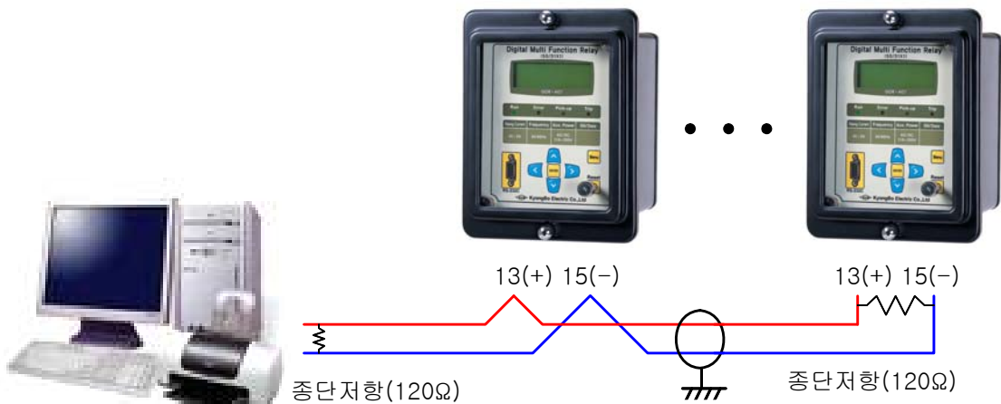
【그림 4.3】 RS-485C 결선도
