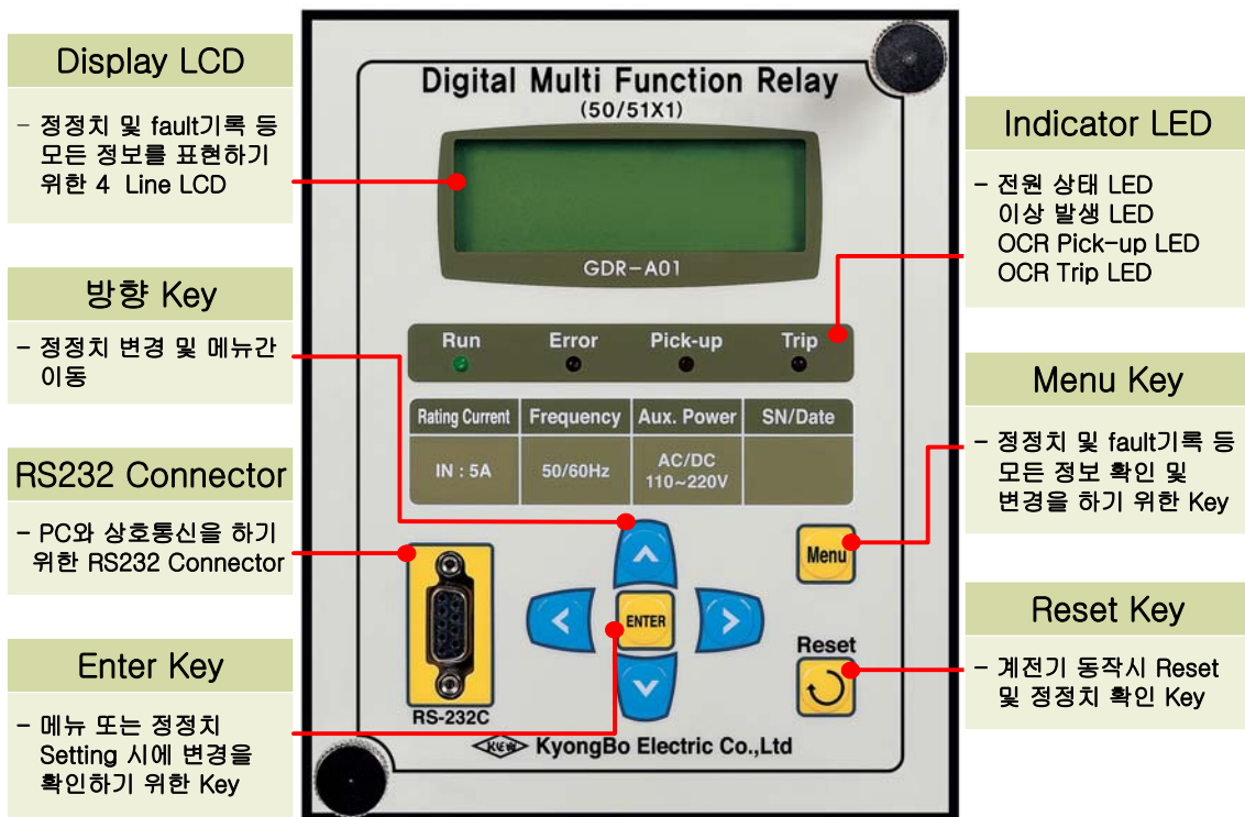
【그림 5.1】 전면 표시부
