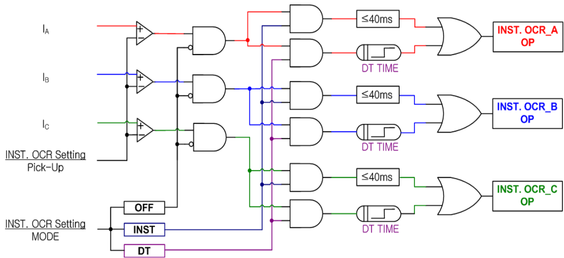
【그림 3.1】 INST.OCR(OCR) Logic Diagram
