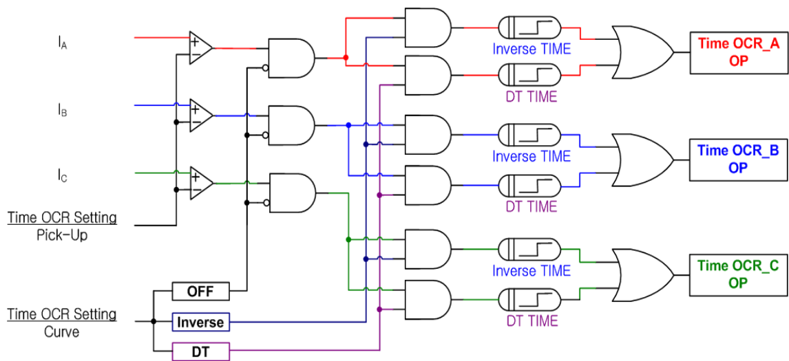
【그림 3.2】 Time OCR(OCR) Logic Diagram
