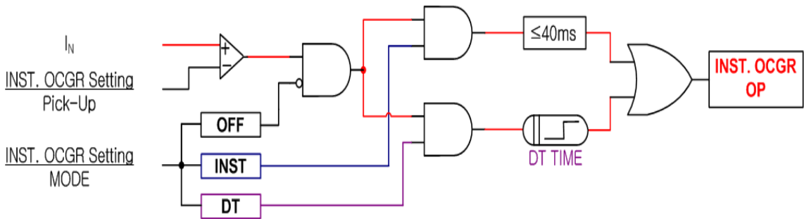
【그림 3.3】 INST.OCGR(IOCGR) Logic Diagram
