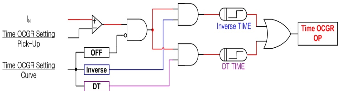
【그림 3.4】 Time OCGR(TOCGR) Logic Diagram
