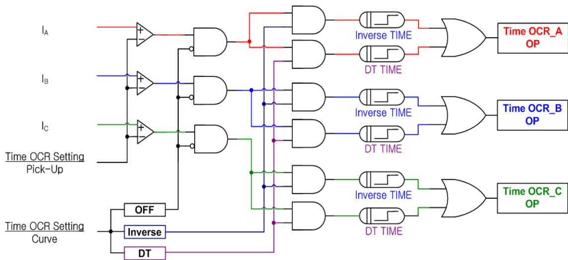
【그림 3.2】 Time OCR(TOCR) Logic Diagram
