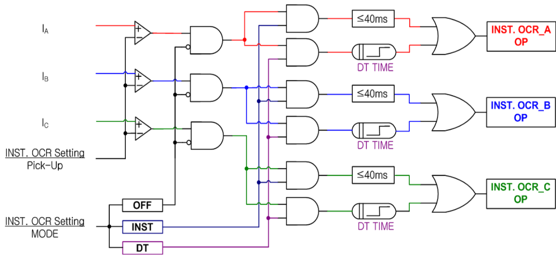
【그림 3.1】 INST.OCR(IOC) Logic Diagram
