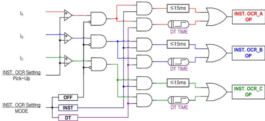
【그림 3.1】 INST.OCR(IOC) Logic Diagram
