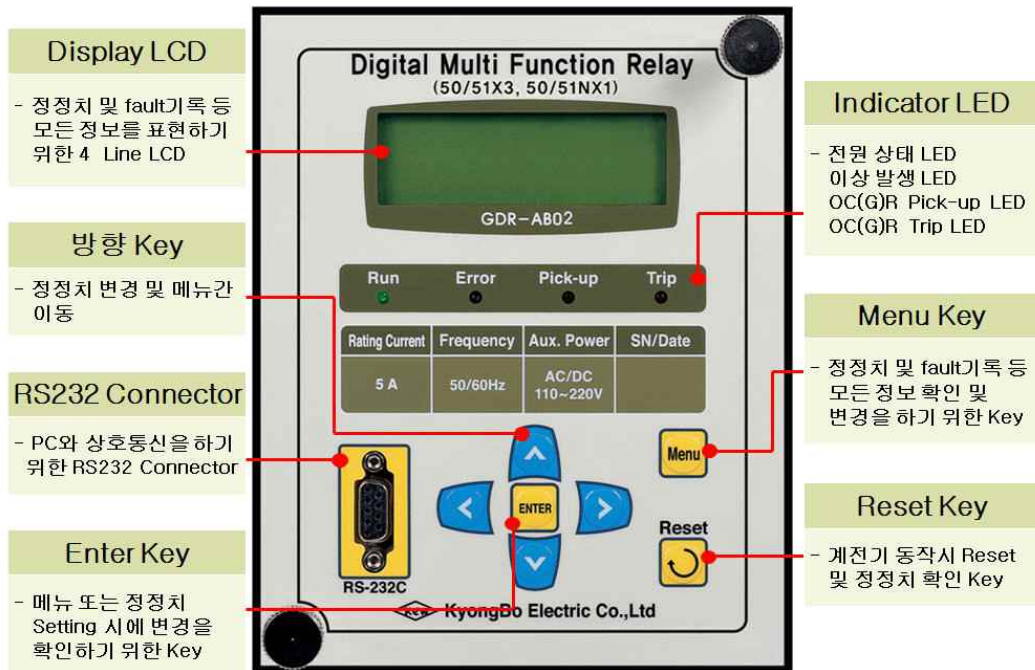
【그림 5.1】 전면 표시부
