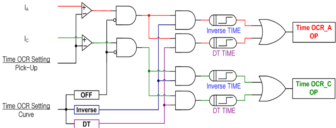
【그림 3.2】 Time OCR(OCR) Logic Diagram
