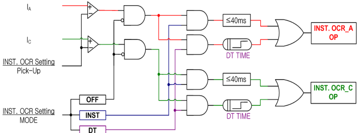
【그림 3.1】 INST. OCR(OCR) Logic Diagram
