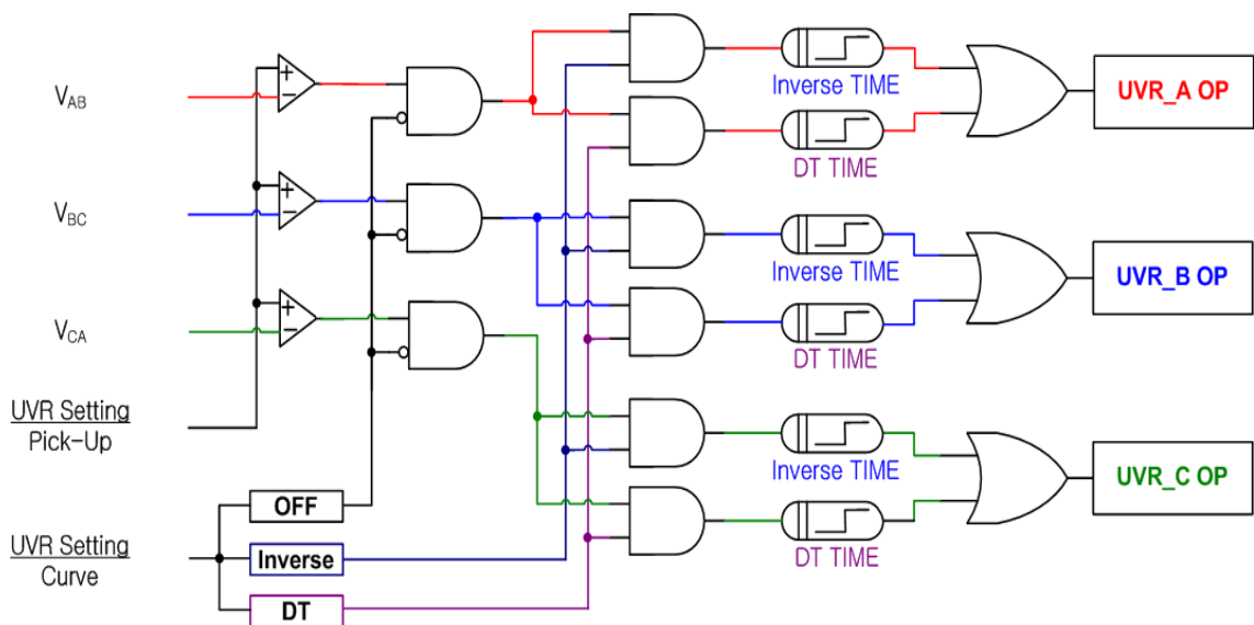
【그림 3.4】 UVR Logic Diagram
