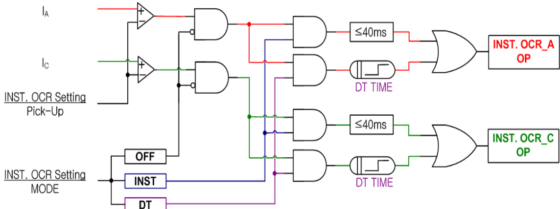
【그림 3.1】 INST. OCR(IOCR) Logic Diagram
