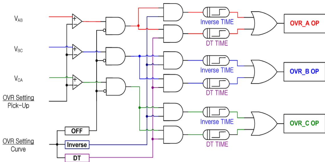
【그림 3.3】 OVR Logic Diagram
