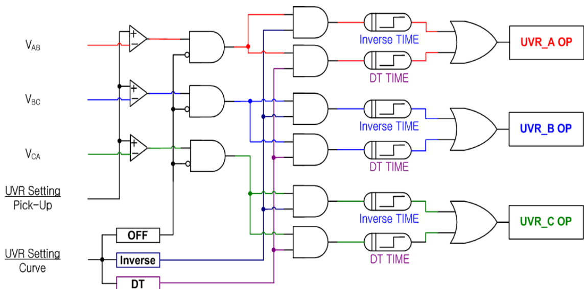
【그림 3.4】 UVR Logic Diagram
