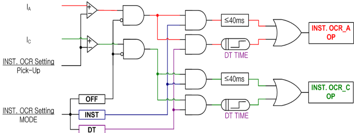
【그림 3.1】 INST. OCR(OCR) Logic Diagram
