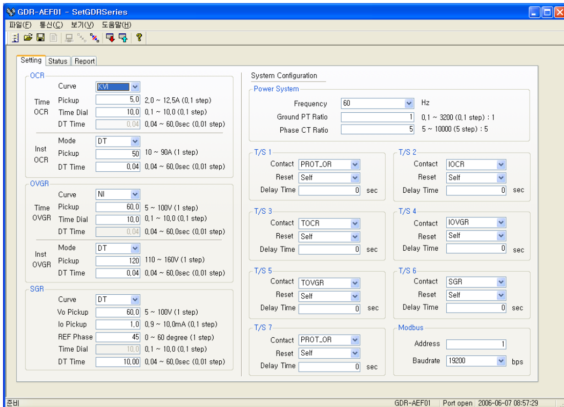
【그림 7.4】 GDR-AEF01 Setting
