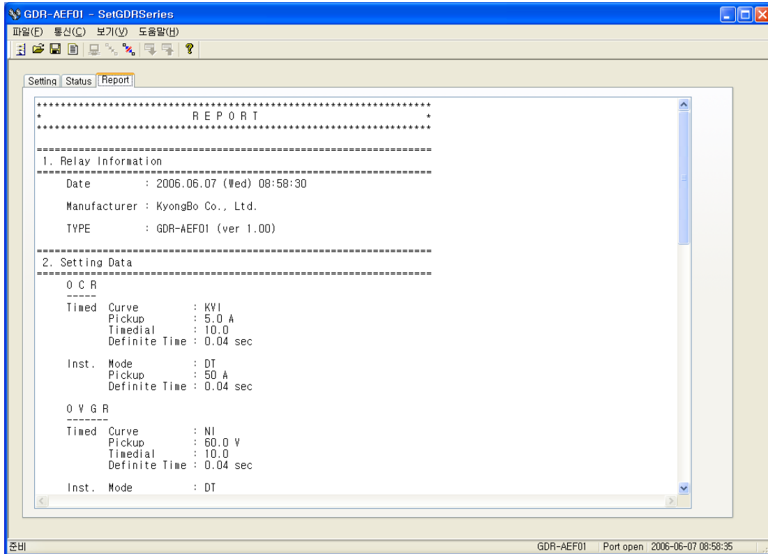
【그림 7.6】 GDR-AEF01 Report
