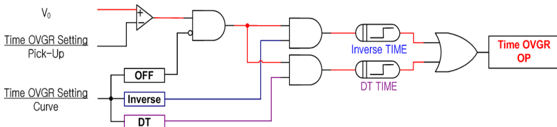
【그림 3.4】 TIME OVGR(TOVGR) Logic Diagram
