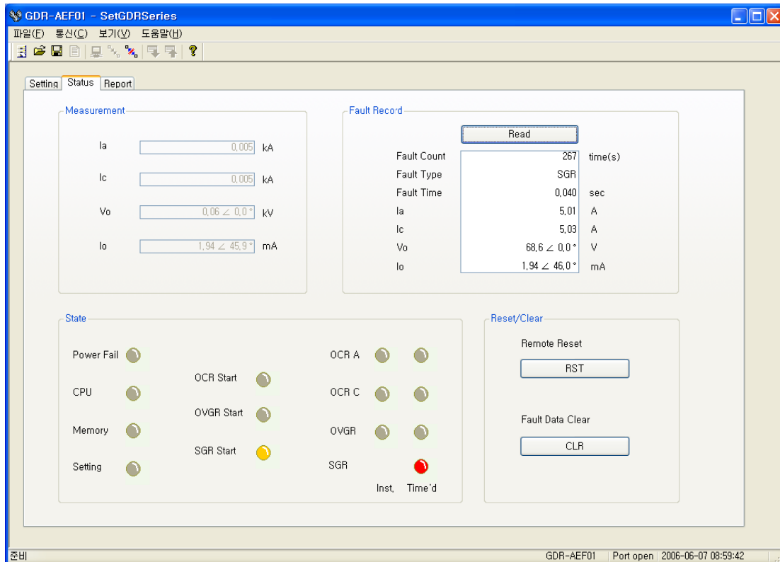
【그림 7.5】 GDR-AEF01 Status
