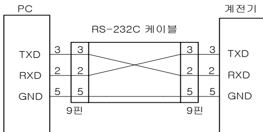
【그림 4.1】 RS-232C 회로도
