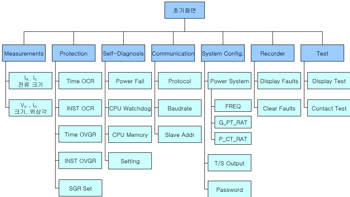
【그림 6.1】 Menu Tree
