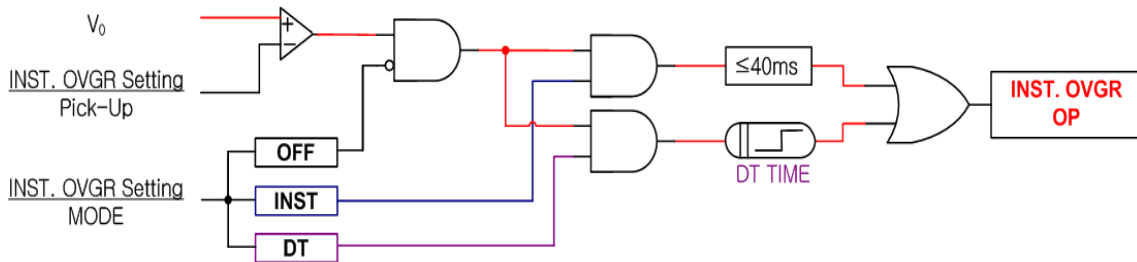
【그림 3.3】 INST. OVGR(IOVGR) Logic Diagram
