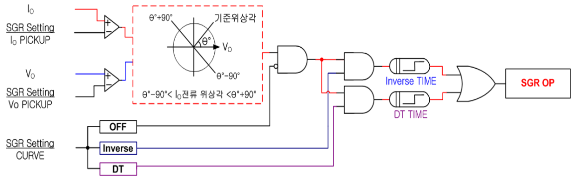
【그림 3.5】 SGR Logic Diagram
